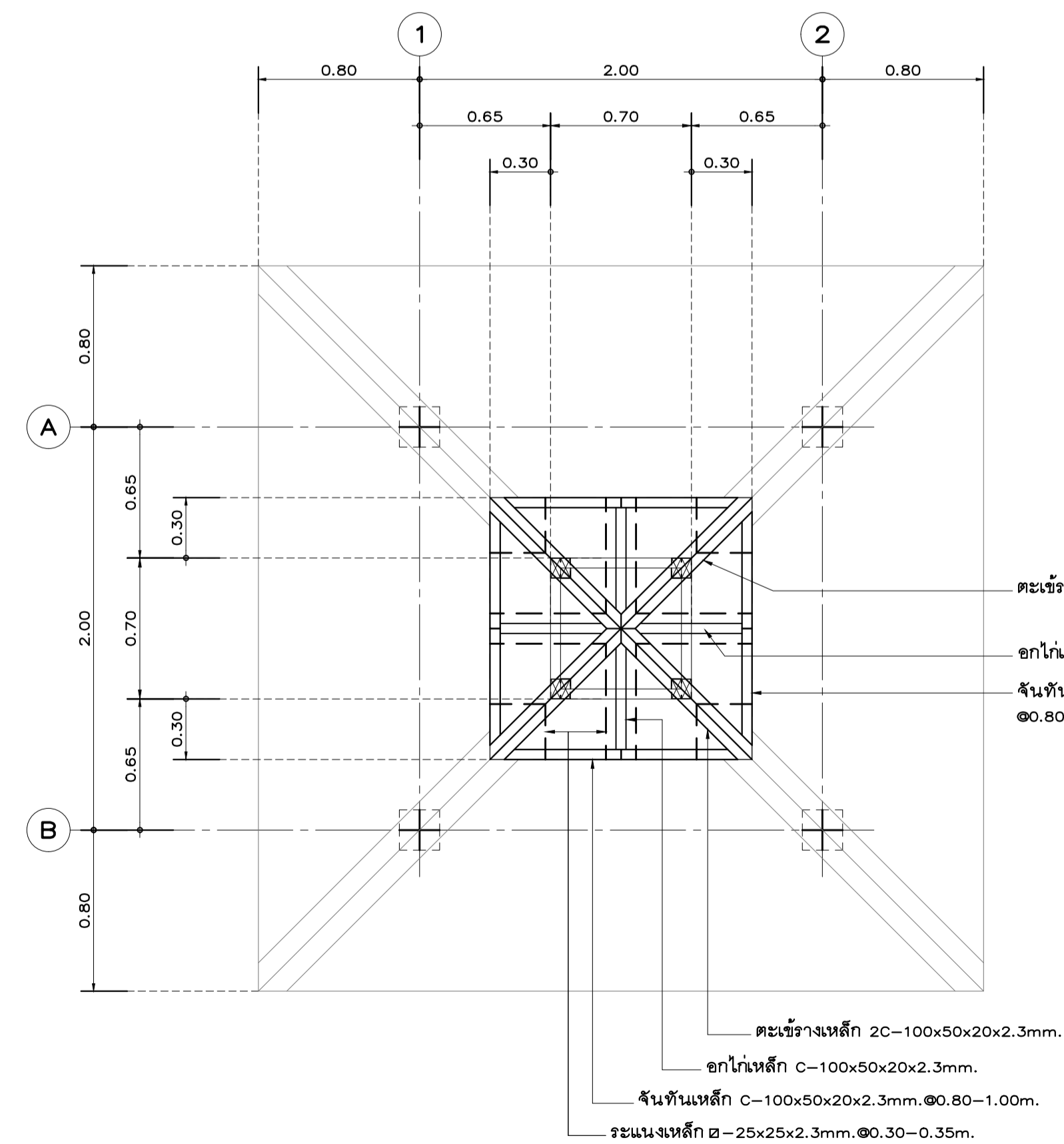
แปลนโครงสร้างหลังคา ชั้นที่ 2 ป้อมยาม มาตราส่วน 1:25
