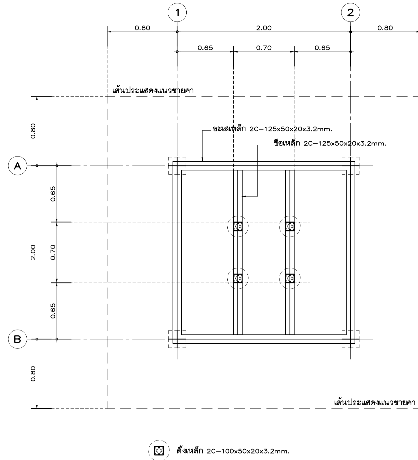
แปลนโครงสร้างอะเส ดั้ง ชั้นที่ 1 ป้อมยาม มาตราส่วน 1:25
