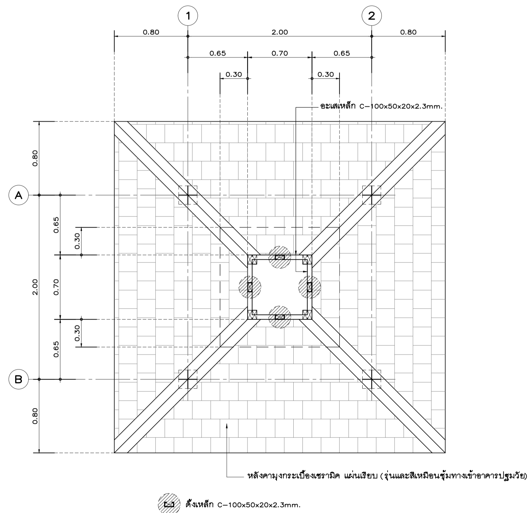
แปลนโครงสร้างอะเส ดั้ง ชั้นที่ 2 ป้อมยาม มาตราส่วน 1:25
