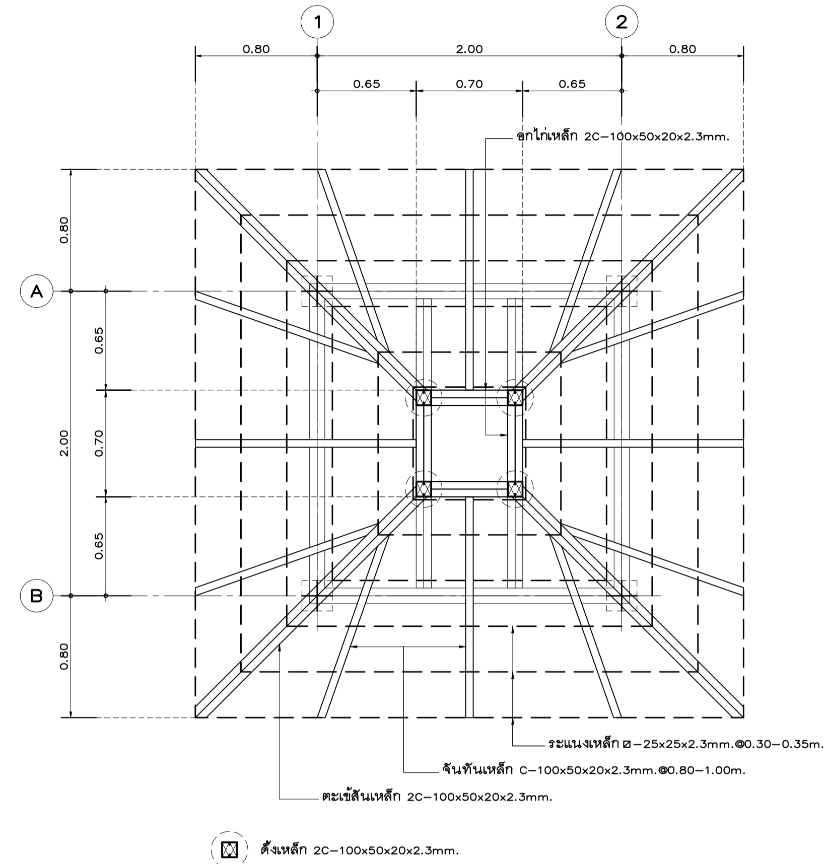
แปลนโครงสร้างหลังคา ชั้นที่ 1 ป้อมยาม มาตราส่วน 1:25
