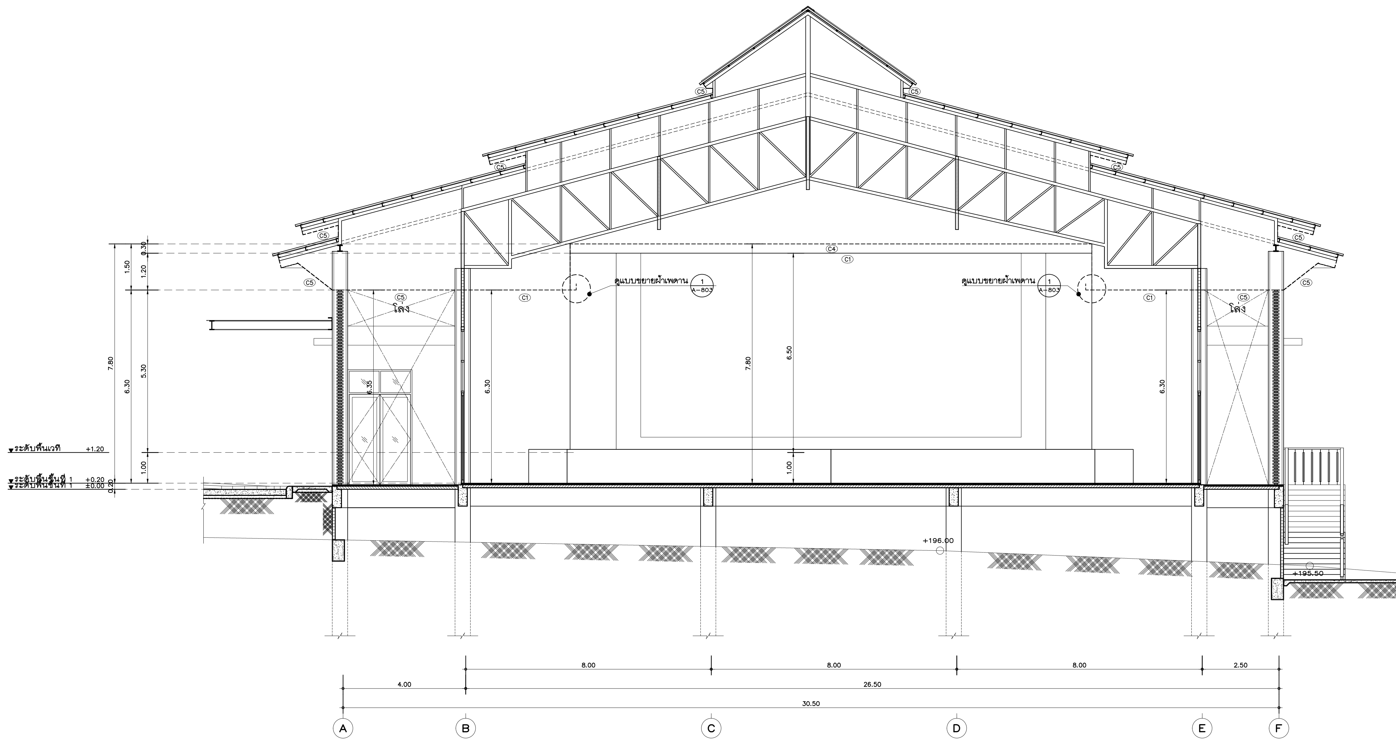
รูปตัดขยายผ้าเพดาน B-B มาตราส่วน 1: 75
