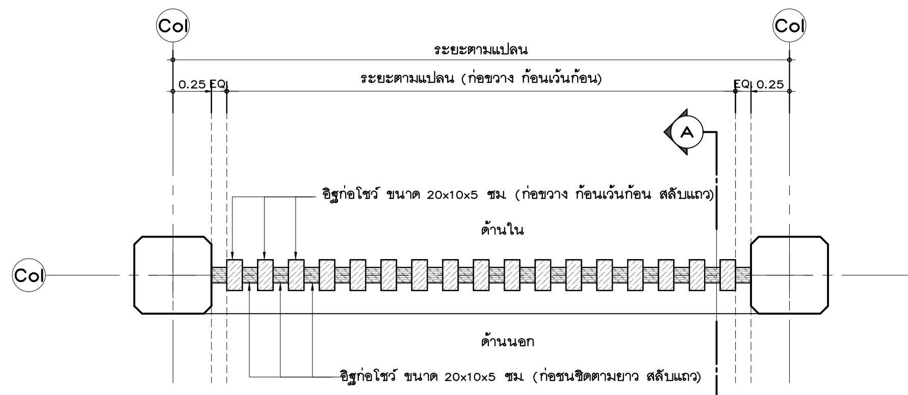
แปลนขยายผนังก่ออิฐโชว์ 5 มาตราส่วน 1:25
