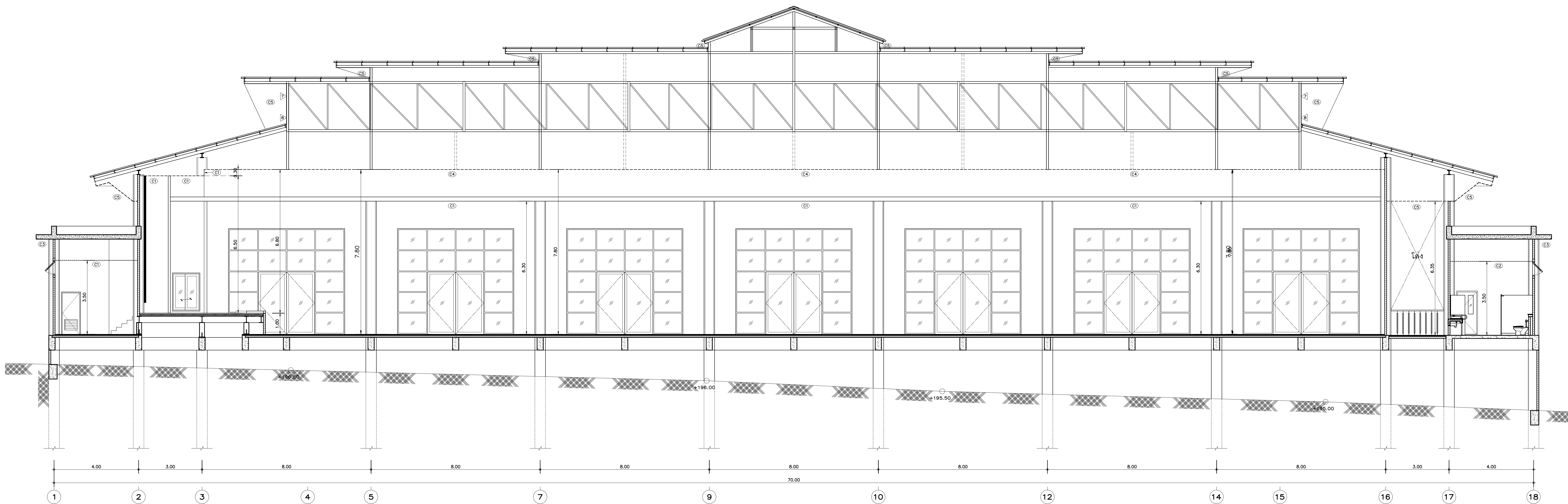
รูปตัดขยายผ้าเพดาน A-A มาตราส่วน 1: 75
