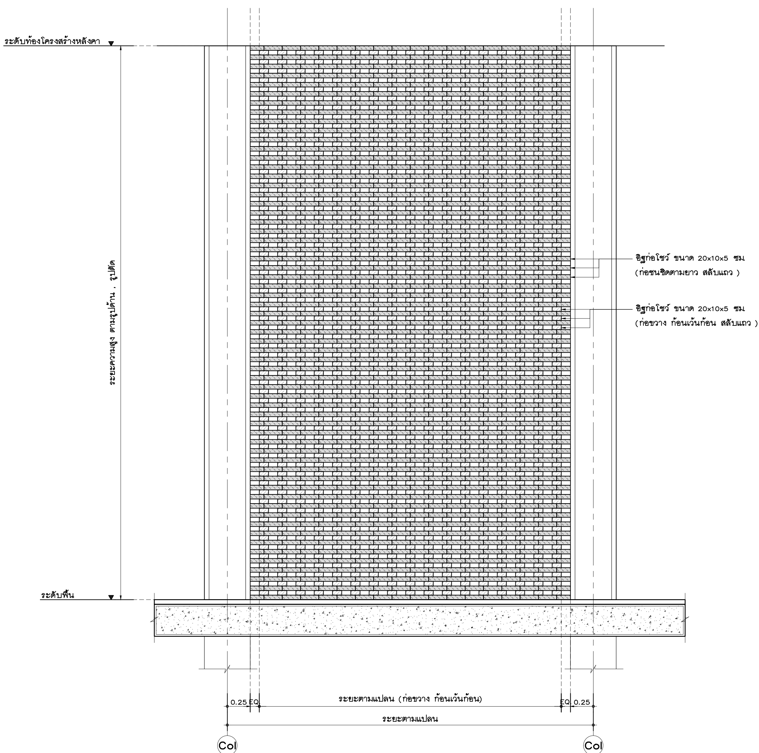
รูปด้านหน้า , ด้านหลัง มาตราส่วน 1:25
