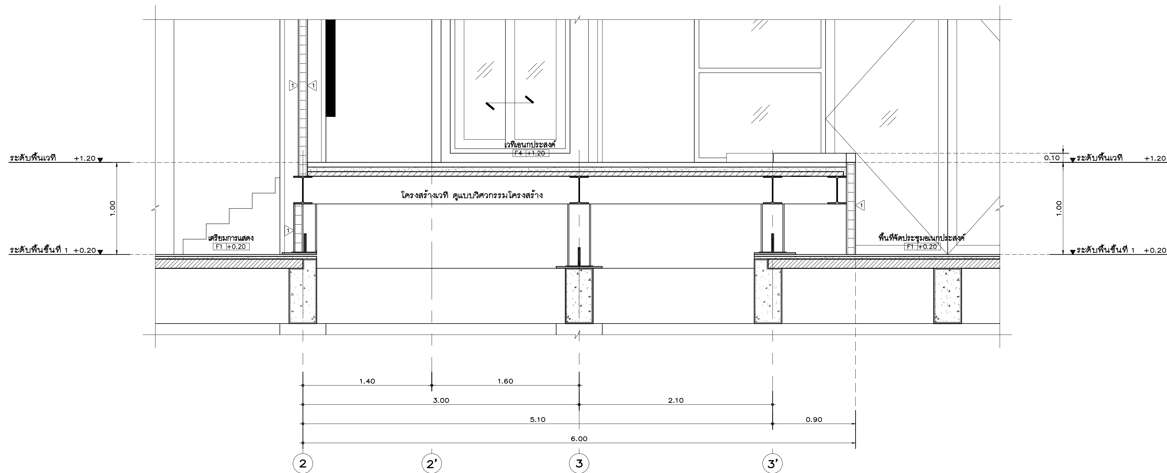
รูปตัด B-B
