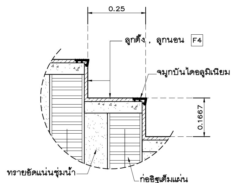
แบบขยายขึ้นบันได มาตราส่วน 1:10
