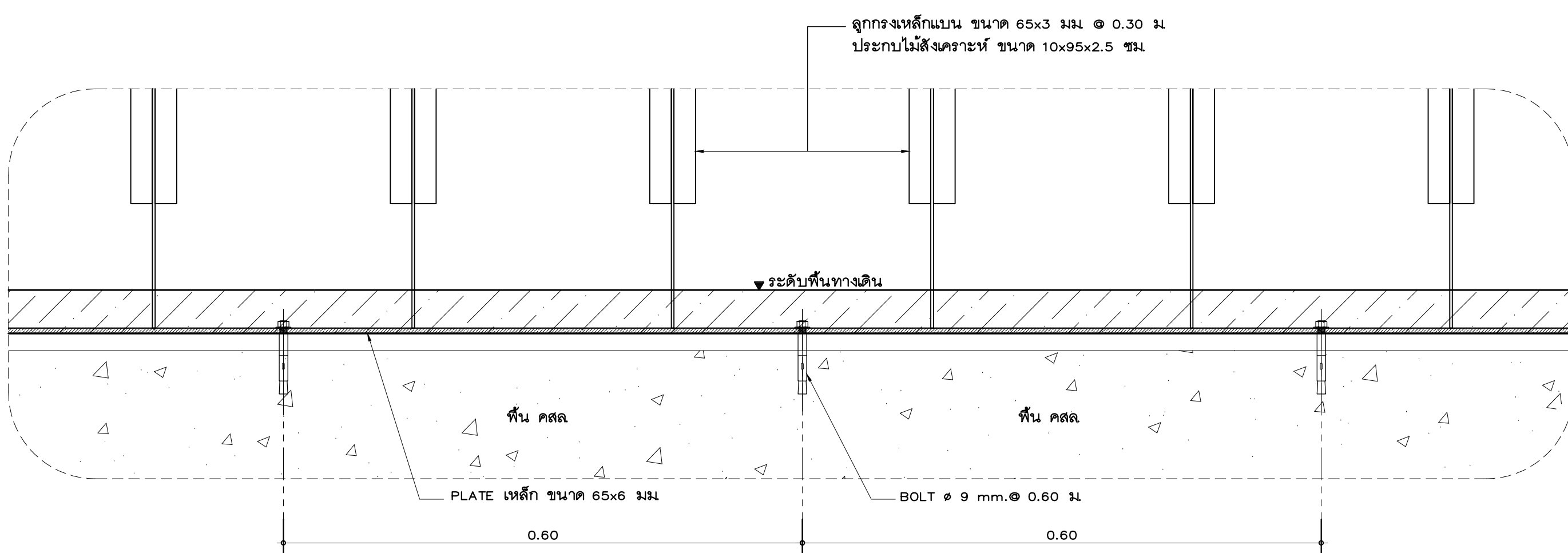
แบบขยาย DET-1 มาตราส่วน 1:5
