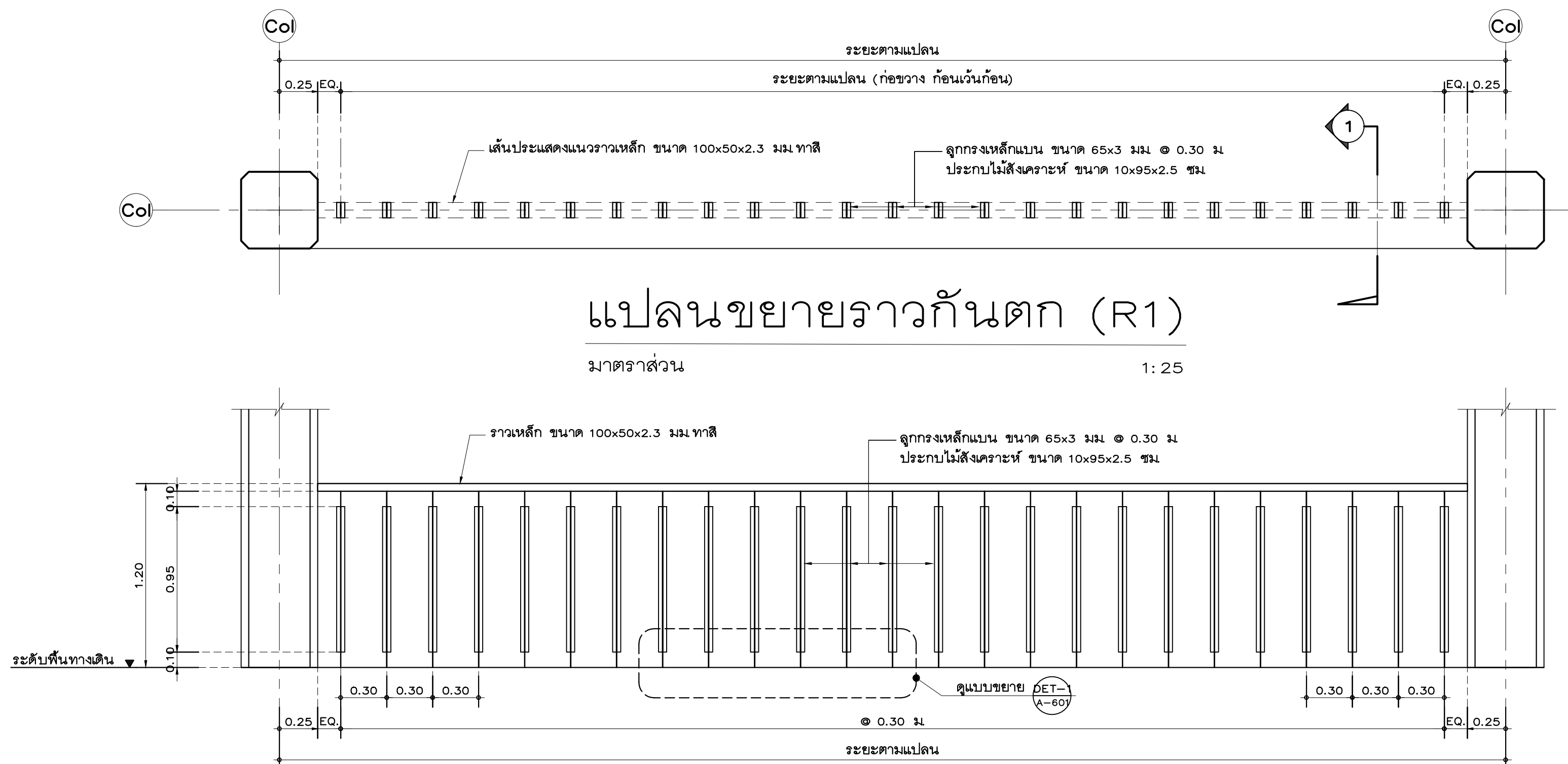
แปลนขยายราวกันตก (R1) มาตราส่วน 1:25
