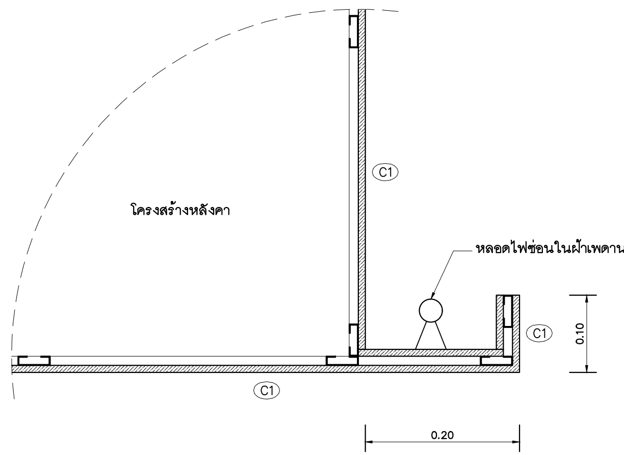
แบบขยายผ้าเพดาน 1 มาตราส่วน 1: 5
