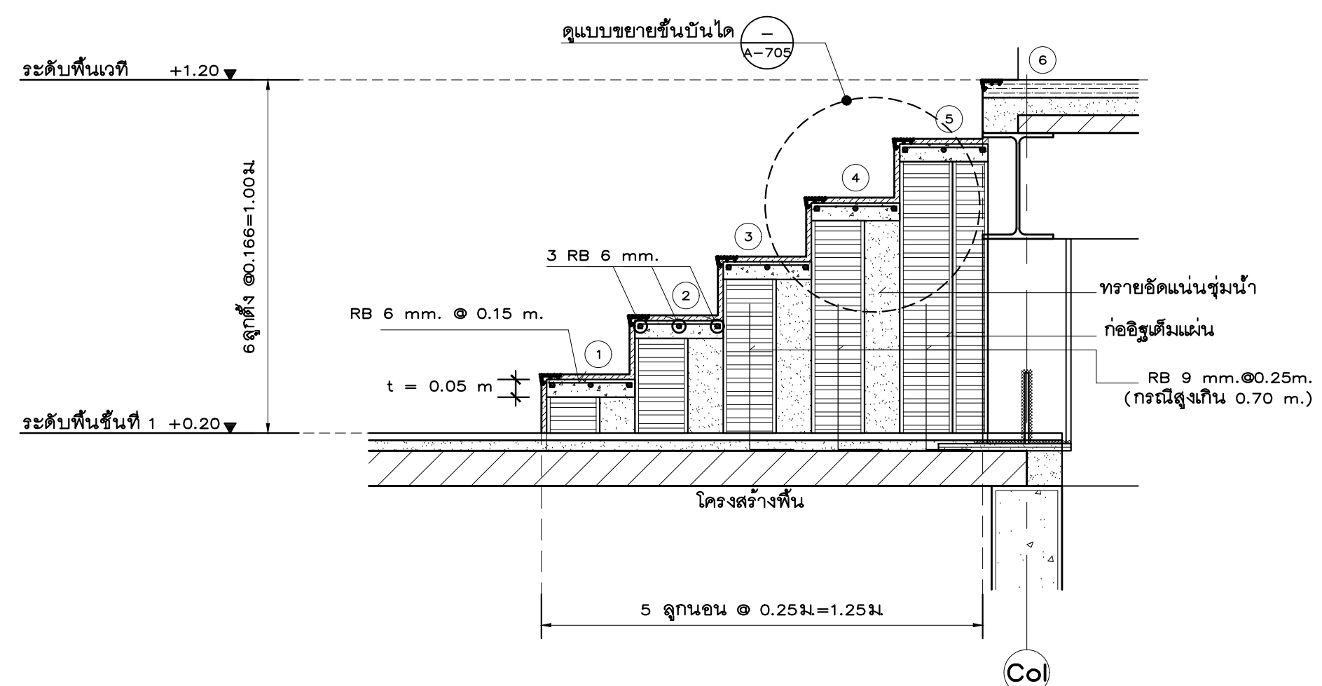
รูปตัดขยายบันได และการเสริมเหล็ก มาตราส่วน 1: 15
