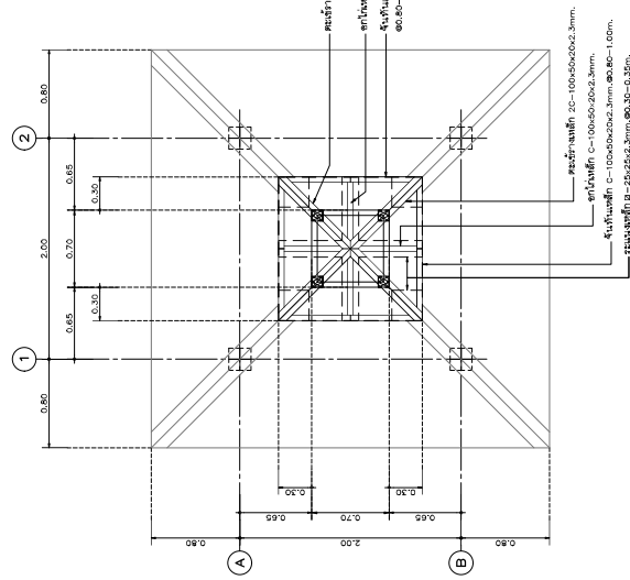
แปลนโครงสร้างหลังคา ชั้นที่ 2 ป้อมยาม
