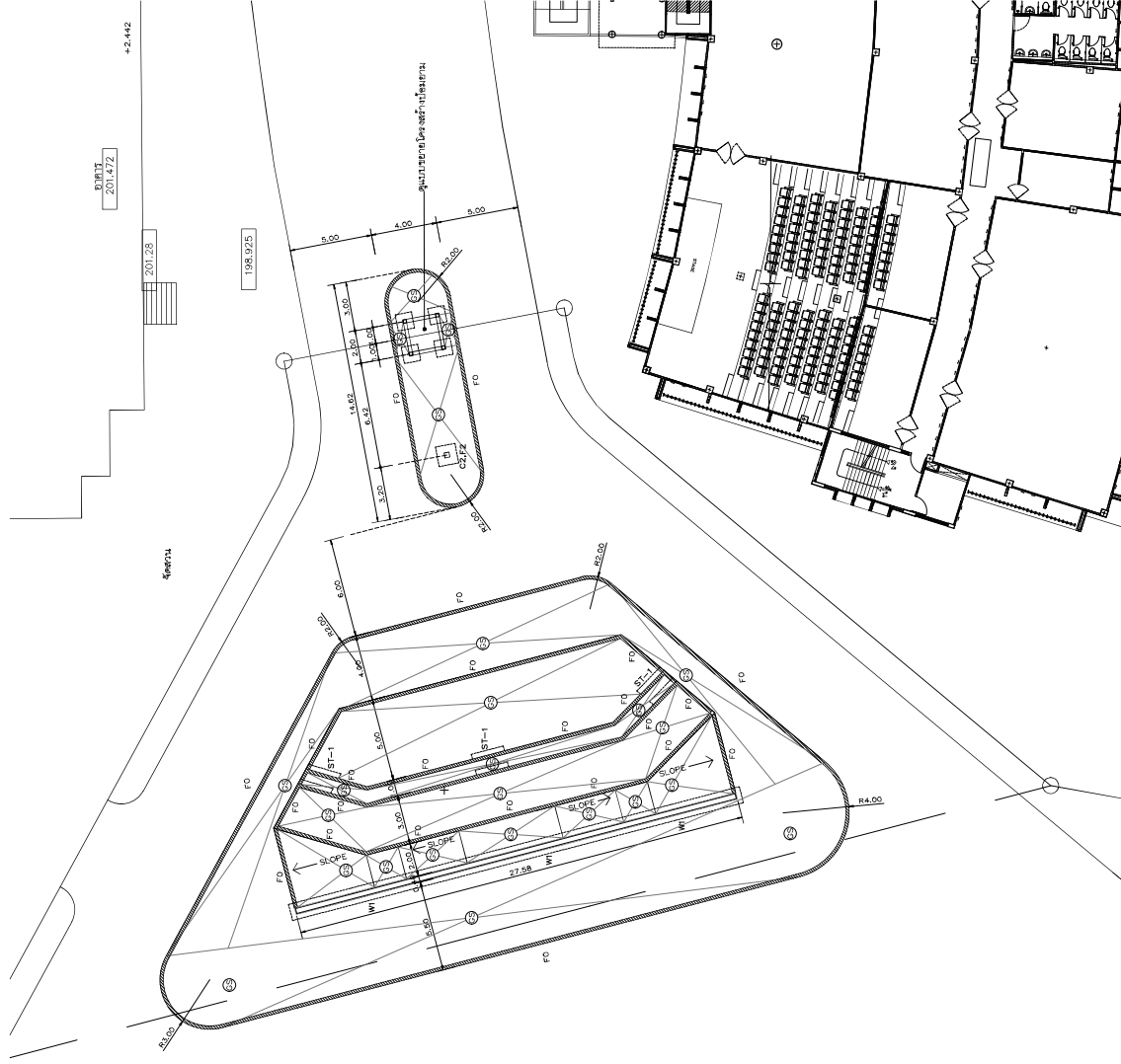
แปลนโครงสร้างลาน PLAZA
