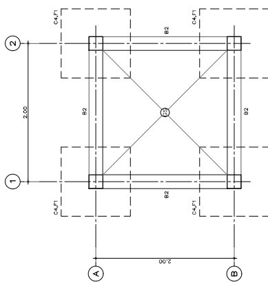
แปลนโครงสร้าง ป้อมยามชั้นล่าง
