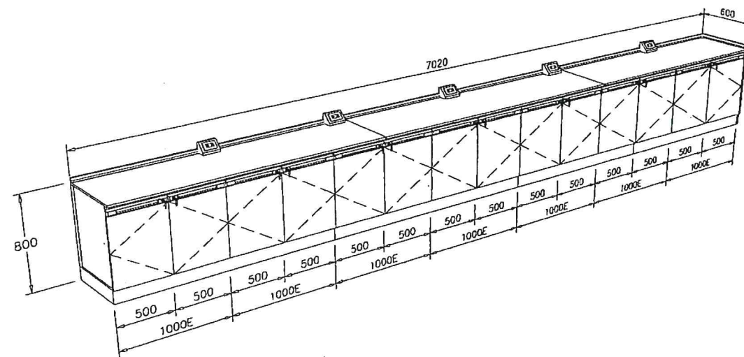
(F-8) : โต๊ะปฏิบัติการติดผนัง ขนาดไม่น้อยกว่า : 7020x600x800 มม.(ท.ล.ส) ห้องเก็บเครื่องมือ : 1 ชุด
