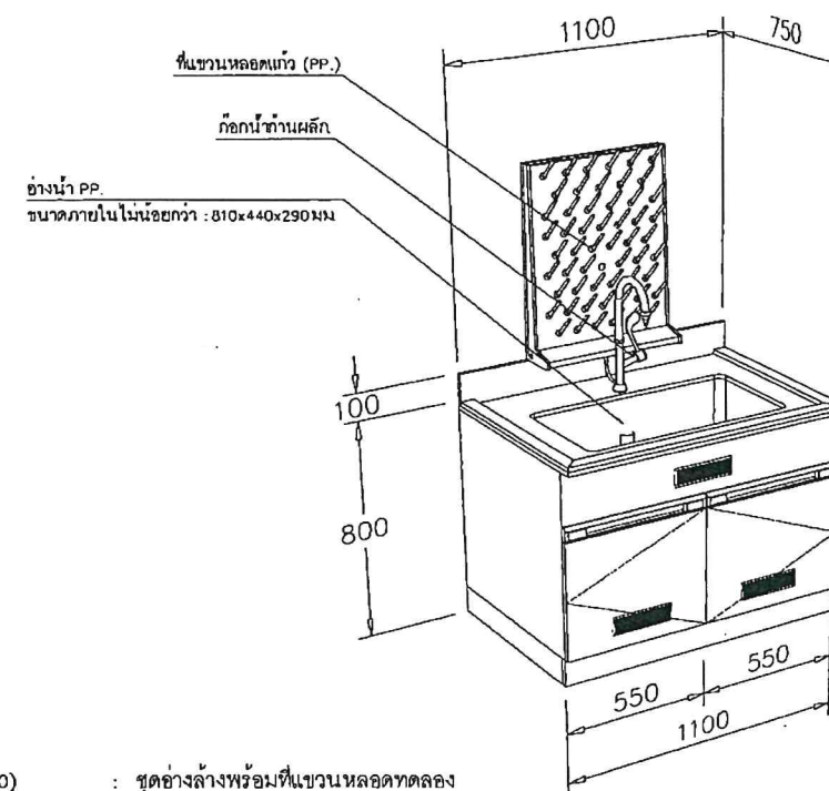
(F-10) : ชุดอ่างล้างพร้อมที่แขวนหลอดทดลอง
