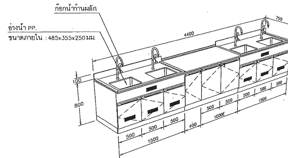
(F-3) : โต๊ะปฏิบัติการติดตั้งพร้อมอ่างล้าง
