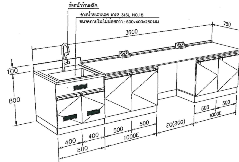
(F-15) : โต๊ะปฏิบัติการติดผนังพร้อมอ่างล้าง ขนาดไม่น้อยกว่า : 3600x750x800 มม.(กxลxส) ห้องเตรียมสารเคมี : 1 ชุด
