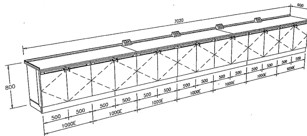
(F-26) : ใต้ปฏิบัติการติดผนัง
