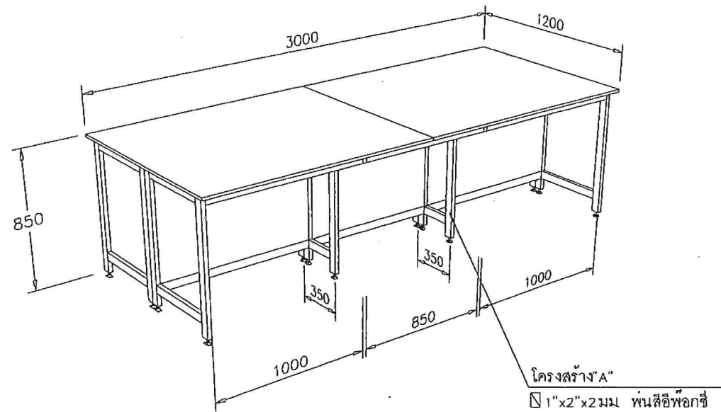
(F-6) : โต๊ะปฏิบัติการกลาง ขนาดไม่น้อยกว่า : 3000x1200x850 มม.(ท.ล.ส) ห้องเก็บเครื่องมือ : 1 ชุด
