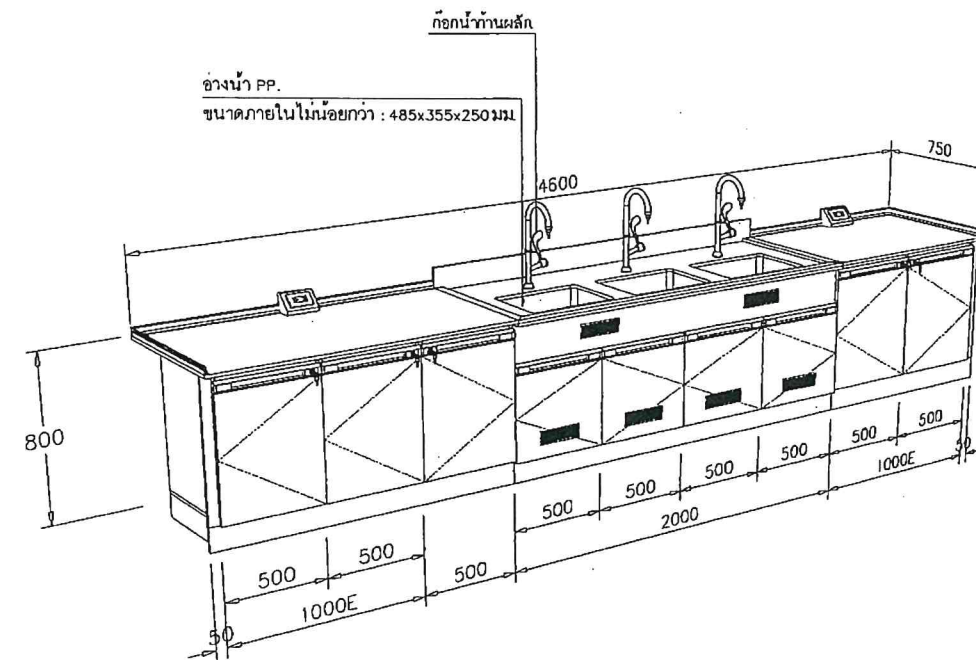
(F-43) : โต๊ะปฏิบัติการติดผนังพร้อมอ่างล้าง ขนาดไม่น้อยกว่า : 4600x750x800 มม.(กxลxส) ห้องเก็บอุปกรณ์ เครื่องแก้ว และห้องล้าง : 1 ชุด
