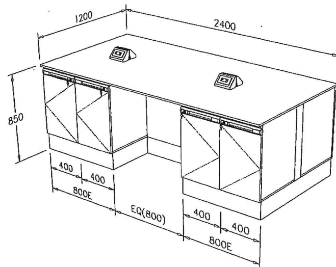
(F-5) : โต๊ะปฏิบัติการกลาง ขนาดไม่น้อยกว่า : 2400x1200x850 มม.(กxลxส) ห้องเก็บอุปกรณ์ เครื่องแก้ว และห้องล้าง : 1 ชุด
