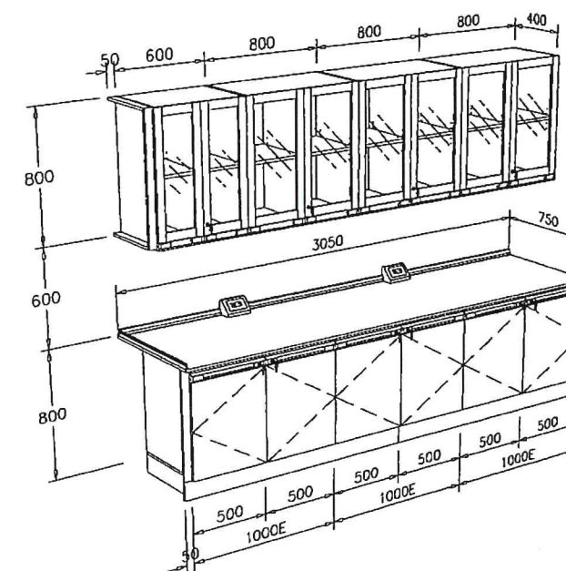
(F-22) : โต๊ะปฏิบัติการติดผนังพร้อมตู้แขวนลอย ขนาดไม่น้อยกว่า : 3050x750x800 มม.(กxลxส) ห้องปฏิบัติการฟิสิกส์ : 1 ชุด
