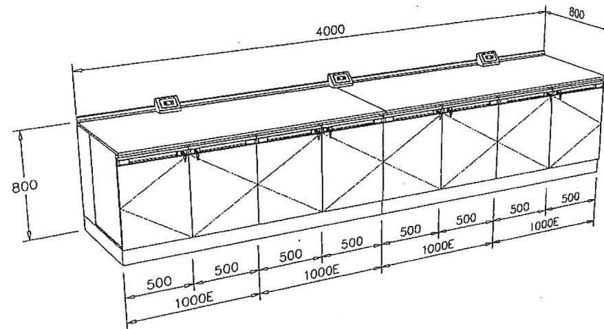
(F-42) : โต๊ะปฏิบัติการติดผนัง ขนาดไม่น้อยกว่า : 4000x800x800 มม.(กxลxส) ห้องเก็บอุปกรณ์ เครื่องแก้ว และห้องล้าง : 1 ชุด
