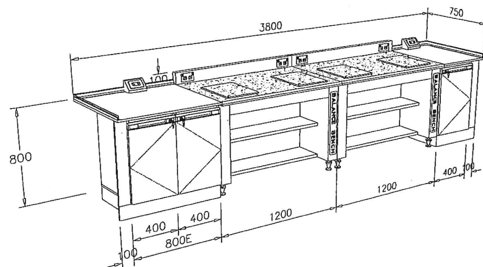
(F-13) : โต๊ะปฏิบัติการติดผนังพร้อมโต๊ะวางเครื่องชั่ง ขนาดไม่น้อยกว่า : 3800x750x800 มม.(กxลxส) ห้องเครื่องชั่ง : 1 ชุด
