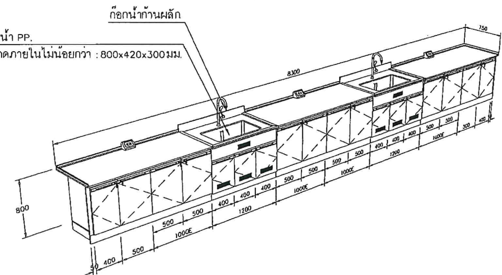
(F-7) : โต๊ะปฏิบัติการติดผนังพร้อมอ่างล้าง ขนาดไม่น้อยกว่า : 8300x750x800 มม.(ท.ล.ส) ห้องเก็บเครื่องมือ : 1 ชุด
