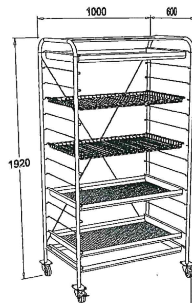
(F-44) : ชั้นสแตนเลสตากอุปกรณ์และเครื่องแก้ว ขนาดไม่น้อยกว่า : 1000x600x1920 มม.(กxลxส) ห้องเก็บอุปกรณ์ เครื่องแก้ว และห้องล้าง : 2 ชุด
