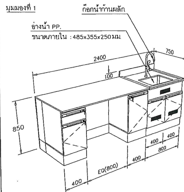
(F-10) : โต๊ะปฏิบัติการกลางพร้อมอ่างล้าง ขนาดไม่น้อยกว่า : 2400x750x850 มม.(กxลxส) ห้องปฏิบัติการฟิสิกส์ : 1 ชุด
