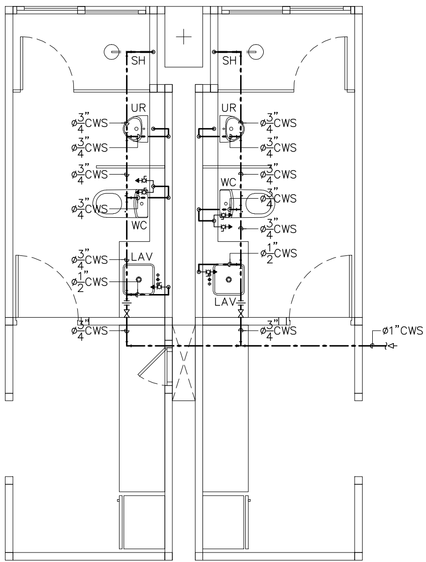
แบบขยายการเดินท่อ CWS ภายในชุดห้องน้ำ 3(อาคาร 2)
