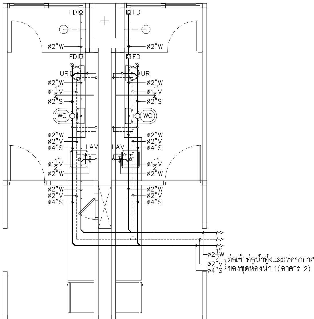
แบบขยายการเดินท่อ S,W,V ภายในชุดห้องน้ำ 3(อาคาร 2)
