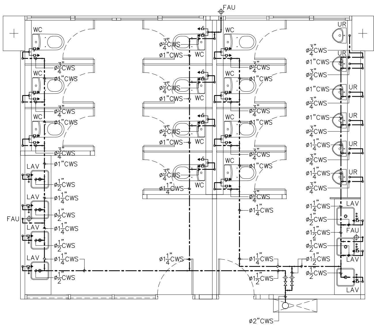
แบบขยายการเดินท่อ CWS ภายในชุดห้องน้ำ 1(อาคาร 2)
