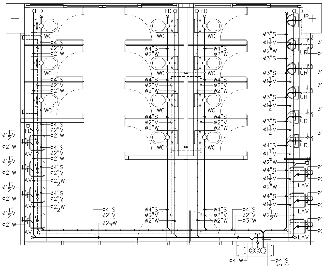
แบบขยายการเดินท่อ S,W,V ภายในชุดห้องน้ำ 1(อาคาร 2)
