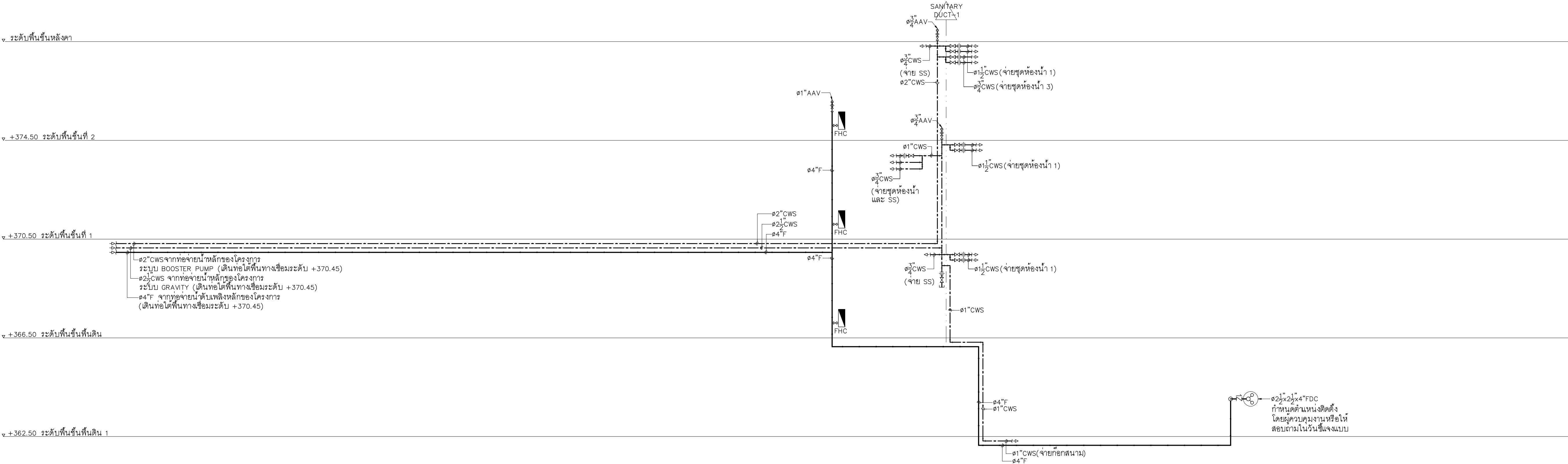
ผังท่อแนวดิ่งของระบบท่อ CWS,F ไม่แสดงขนาดวาล์ว
