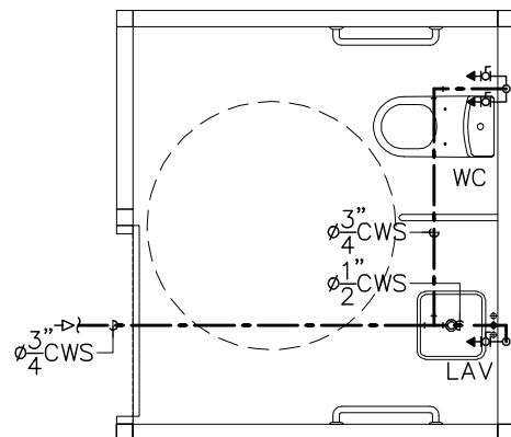
แบบขยายการเดินท่อ CWS ภายในชุดห้องน้ำ 2(อาคาร 4)
