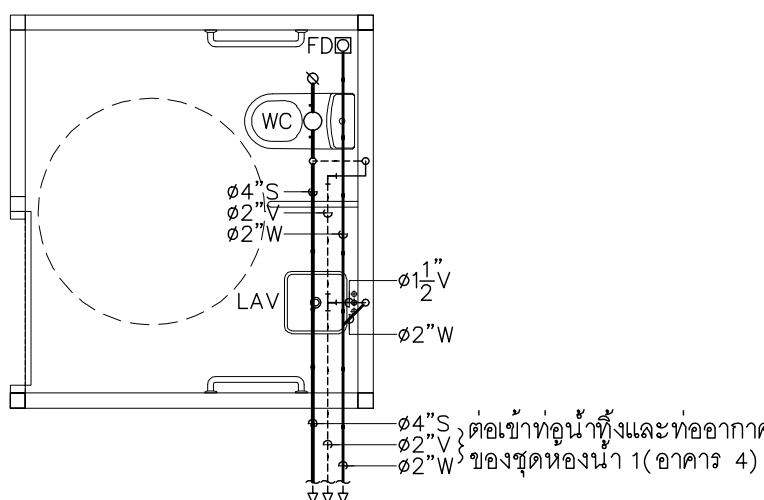
แบบขยายการเดินท่อ S,W,V ภายในชุดห้องน้ำ 2(อาคาร 4)
