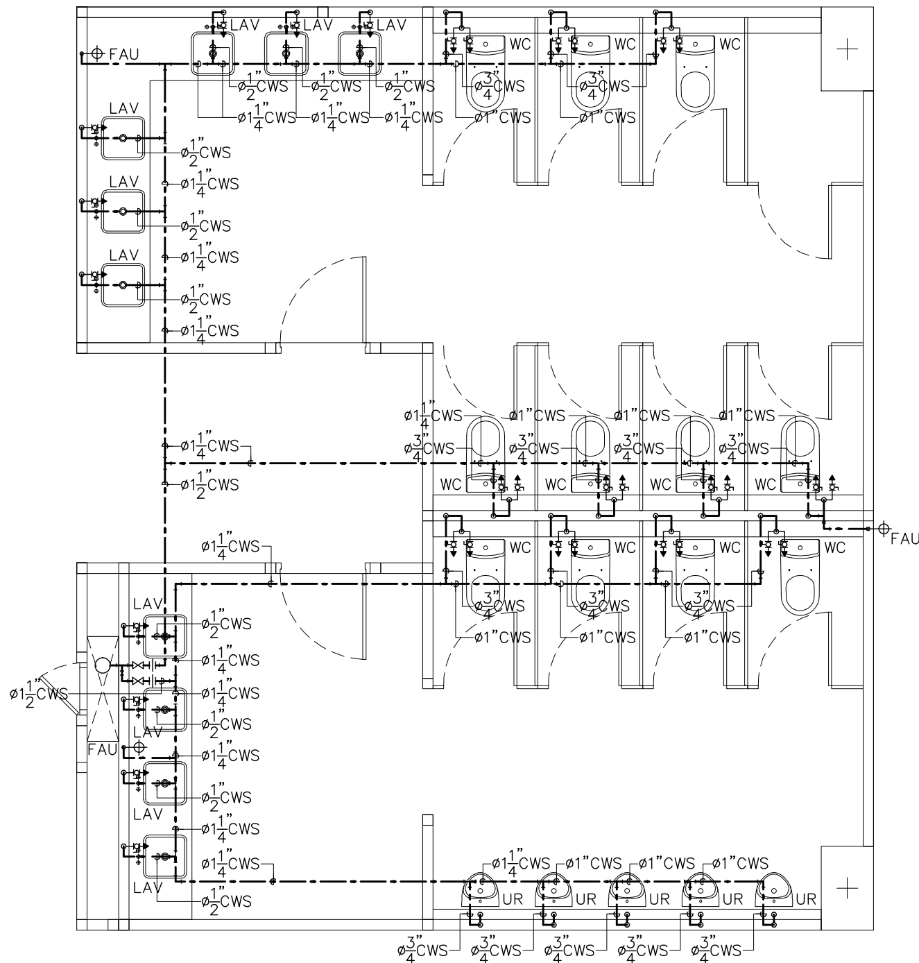
แบบขยายการเดินท่อ CWS ภายในชุดห้องน้ำ 1(อาคาร 4)
