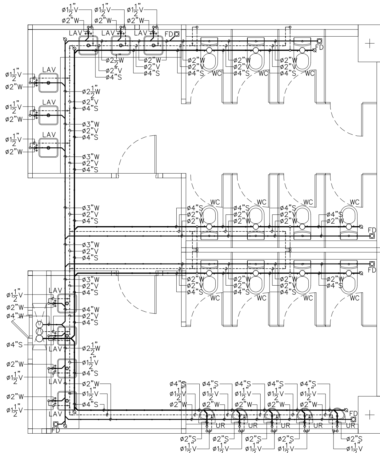
แบบขยายการเดินท่อ S,W,V ภายในชุดห้องน้ำ 1(อาคาร 4)
