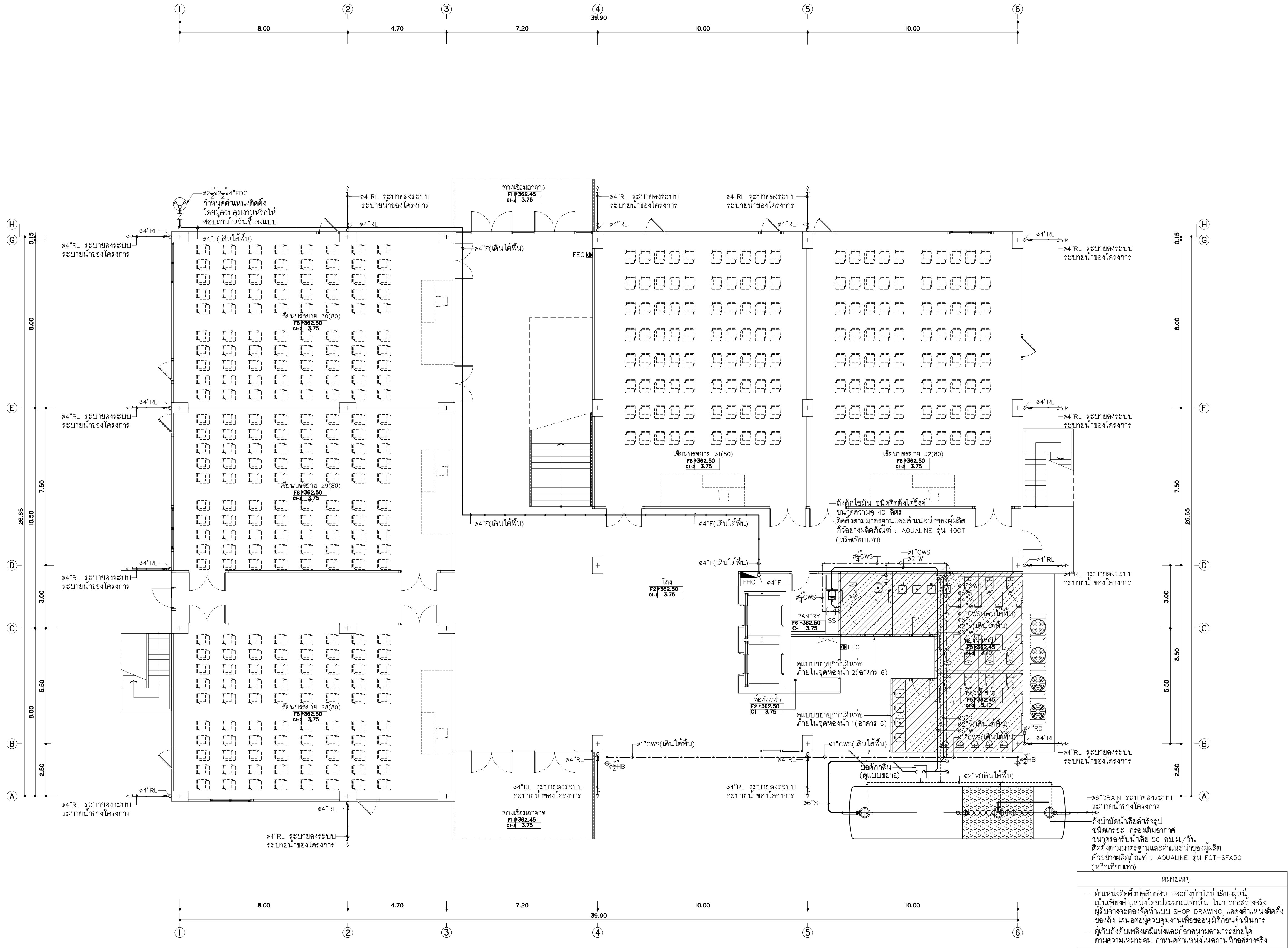
แปลนระบบสุขาภิบาลพื้นที่ชั้นพื้นดิน(อาคาร 6)
