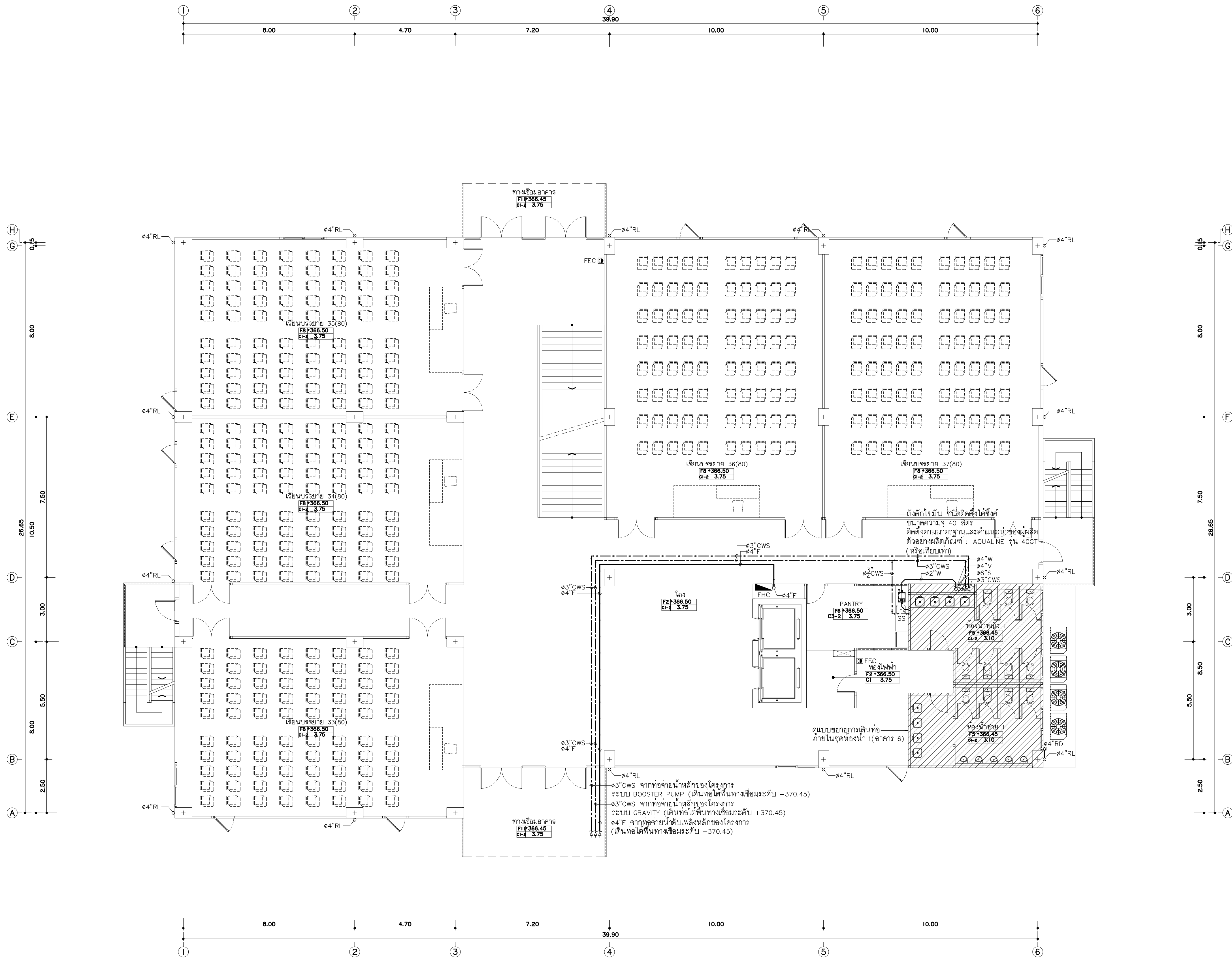
แปลนระบบสุขาภิบาลพื้นที่ 1(อาคาร 6) มาตราส่วน 1 : 100
