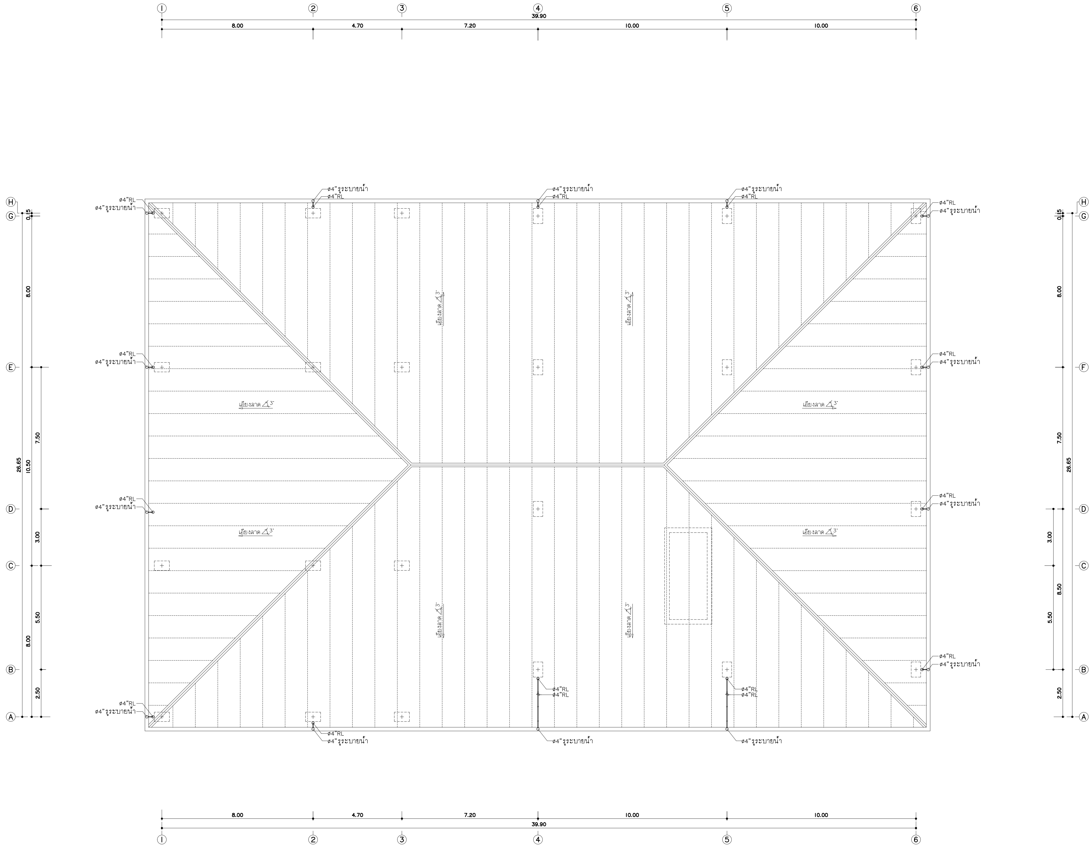
แปลนระบบสุขาภิบาลพื้นที่ชั้นหลังคา(อาคาร 6)
