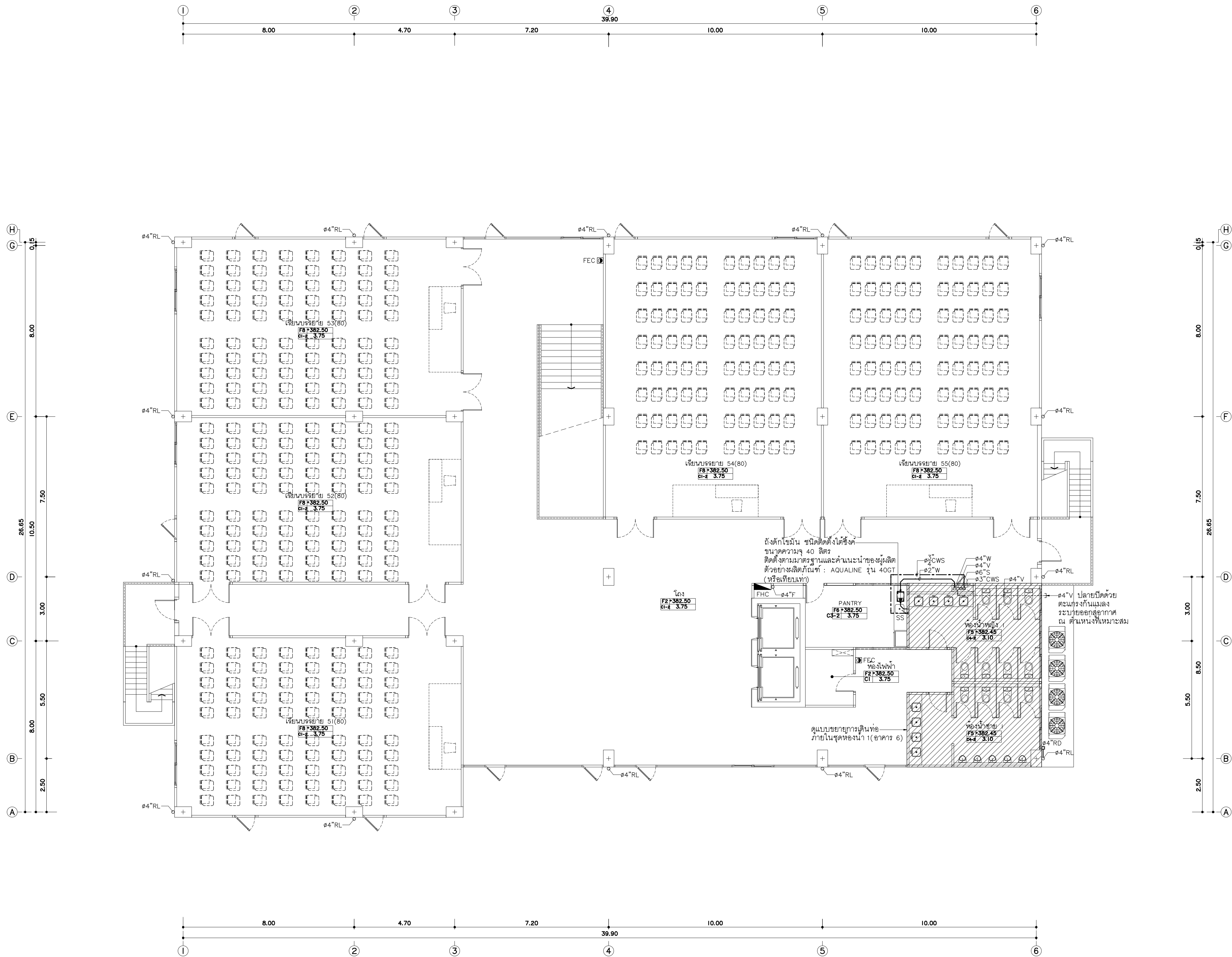
แปลนระบบสุขาภิบาลพื้นที่ 5(อาคาร 6) มาตราส่วน 1 : 100
