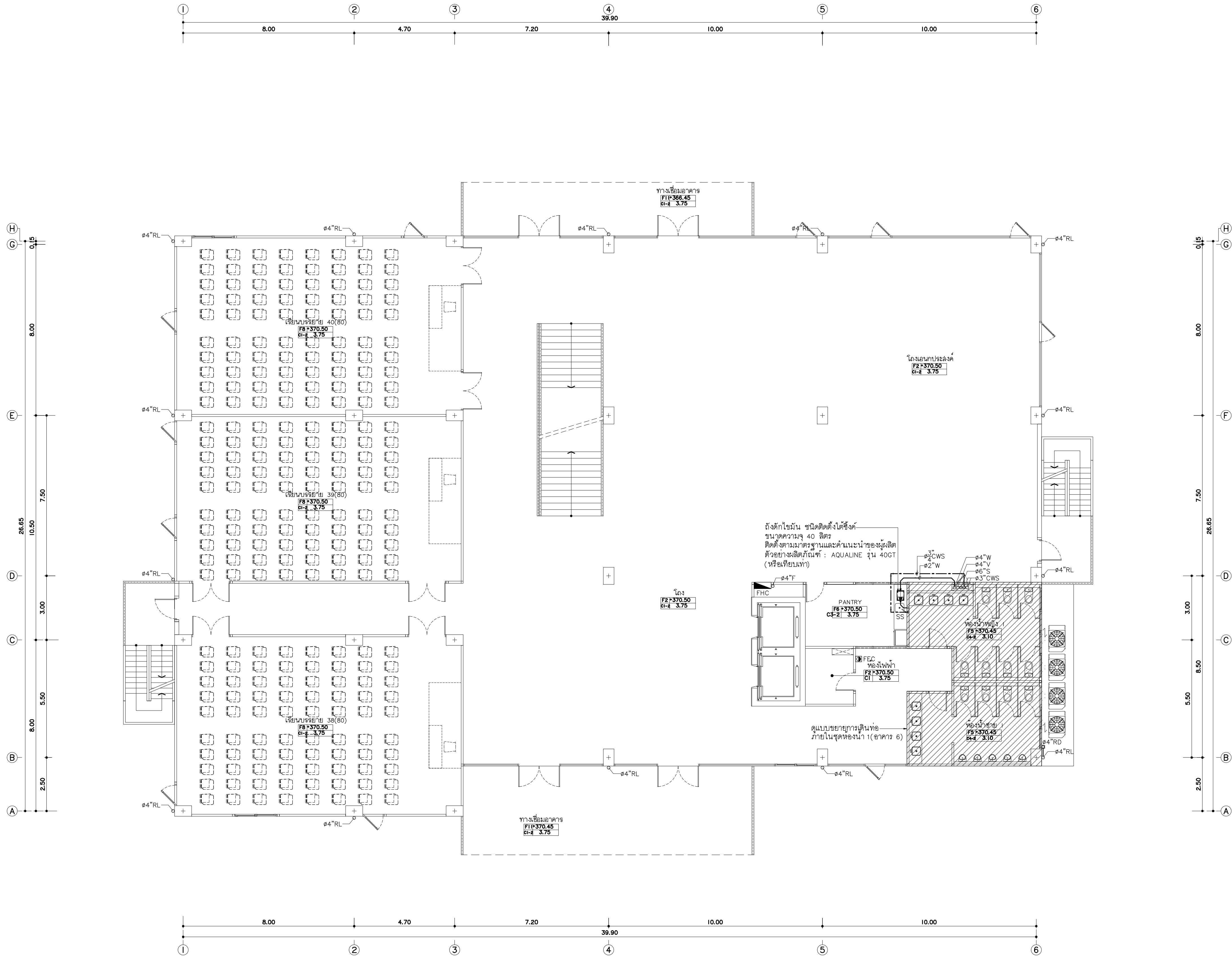
แปลนระบบสุขาภิบาลพื้นที่ 2(อาคาร 6) มาตราส่วน 1 : 100
