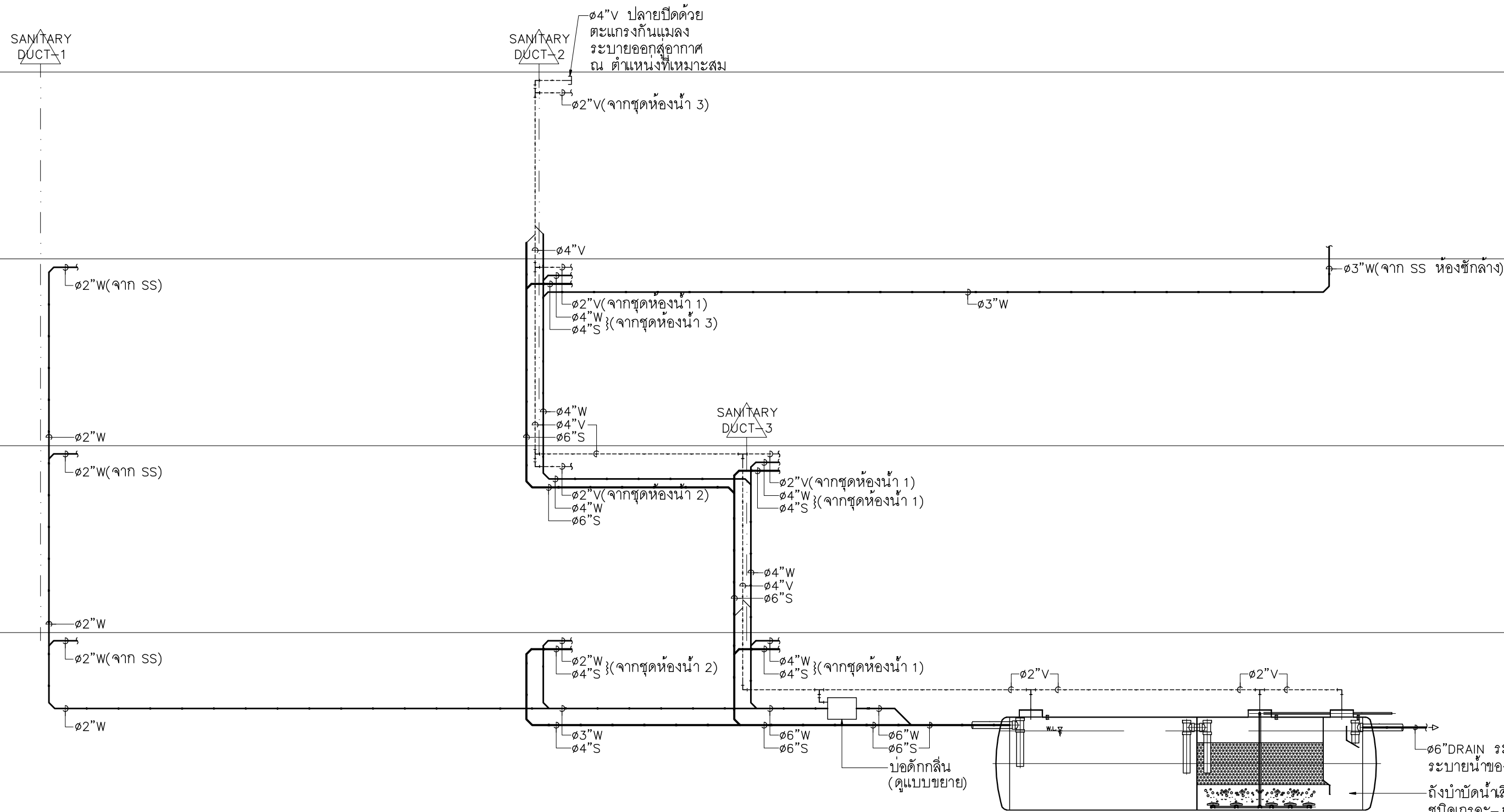
ผังท่อแนวตั้งของระบบท่อ S,W,V(อาคาร 8)
