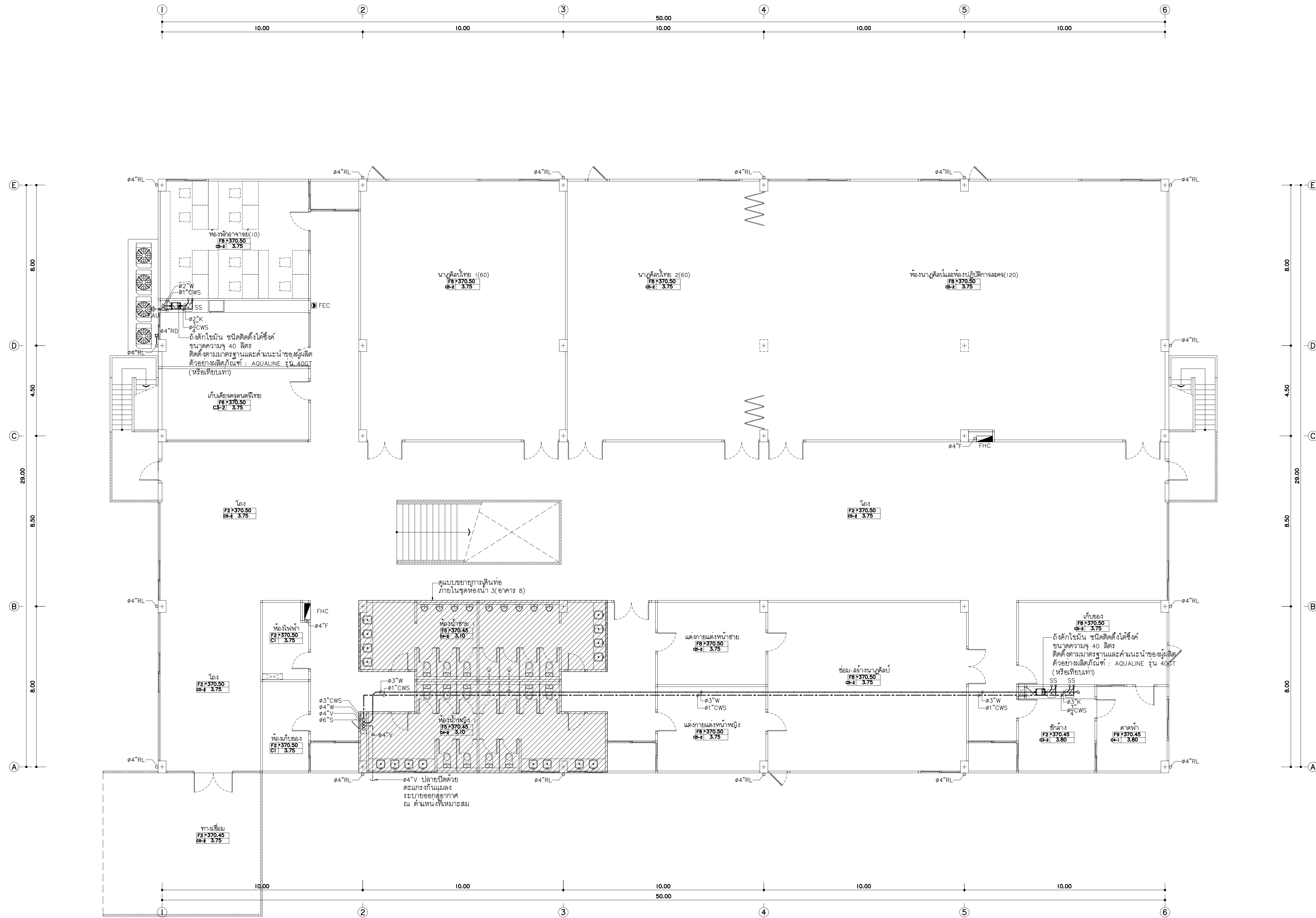
แปลนระบบสุขาภิบาลพื้นที่ 2(อาคาร 8) มาตราส่วน 1 : 100
