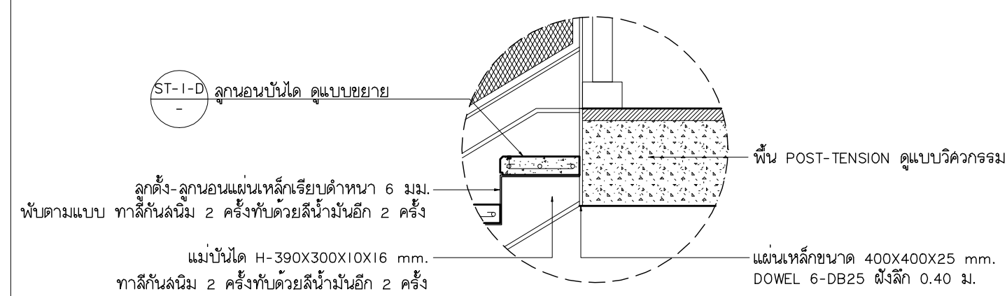
แบบขยาย ST-1-B มาตราส่วน 1:20
