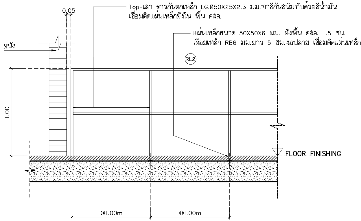
แบบขยายจากรับคาน RL2 มาตราส่วน 1:25
