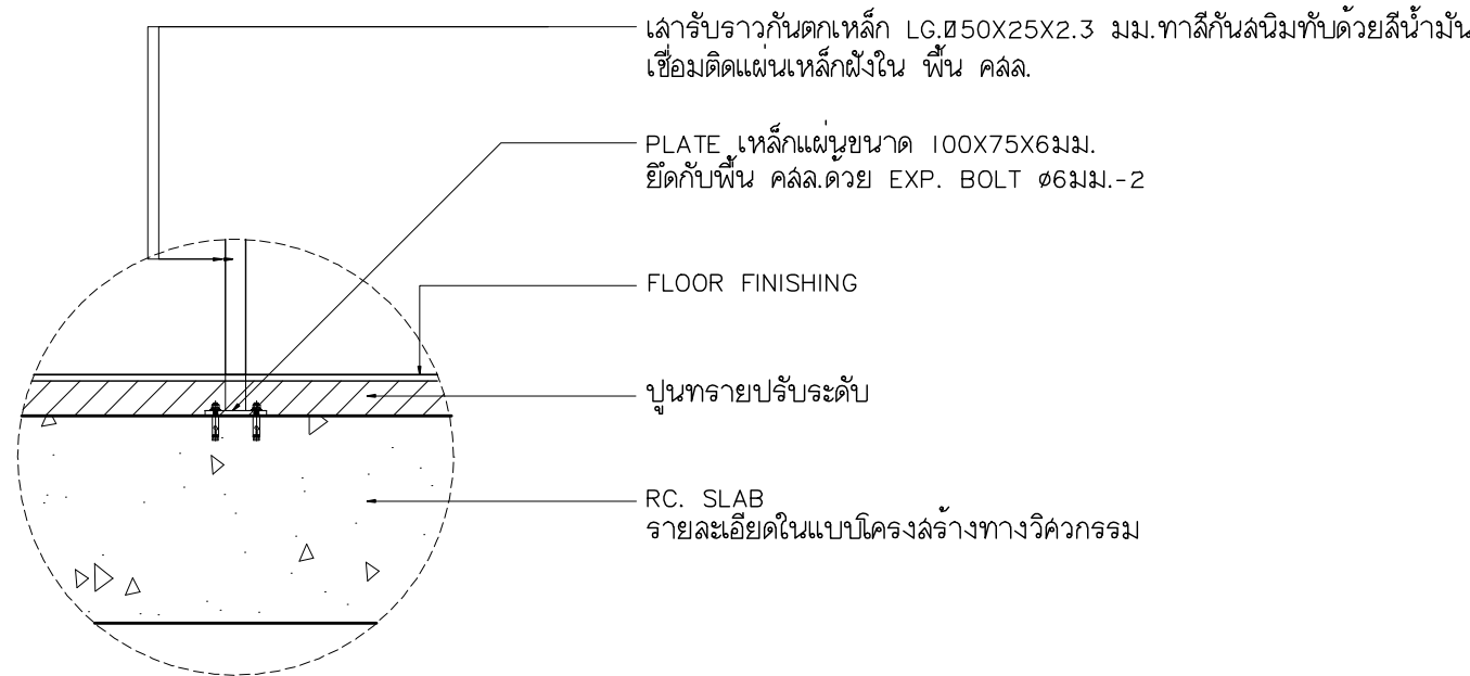
แบบขยาย GT2-1 มาตราส่วน 1:20
