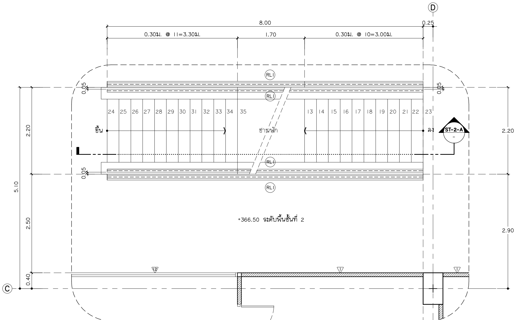
แบบขยายบันได ST-2 ชั้นที่ 2 มาตราส่วน 1:50
