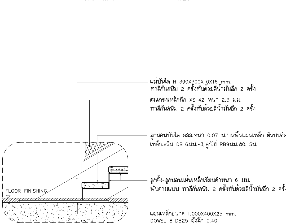
แบบขยาย ST-2-E มาตราส่วน 1:20
