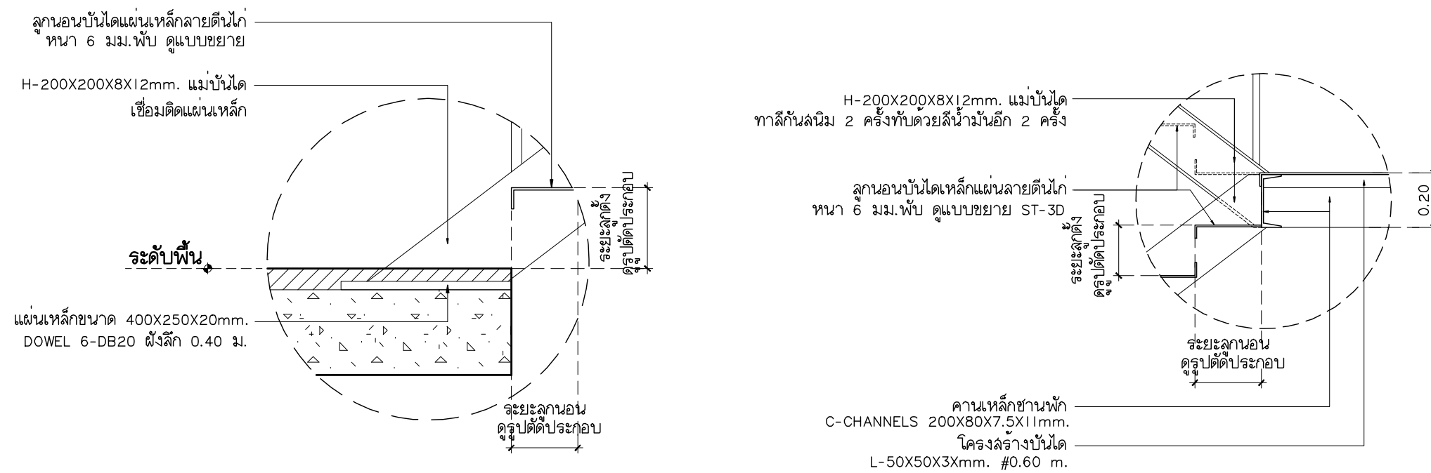
แบบขยาย ST-3-A มาตราส่วน 1:20
