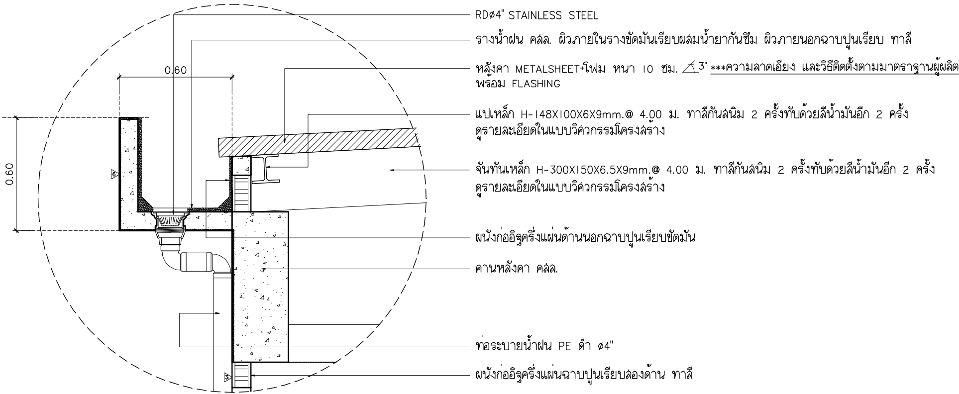
แบบขยาย GTI มาตราส่วน 1:20
