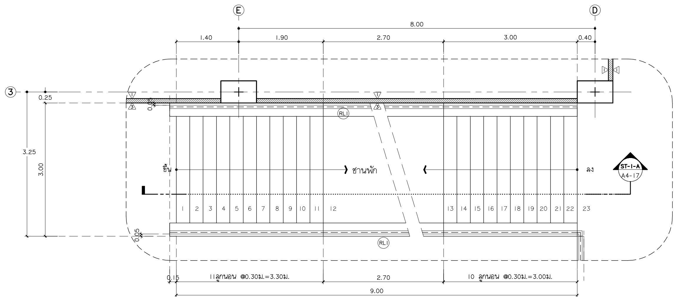
แบบขยายบันได ST-1 แพลน มาตราส่วน 1:50
