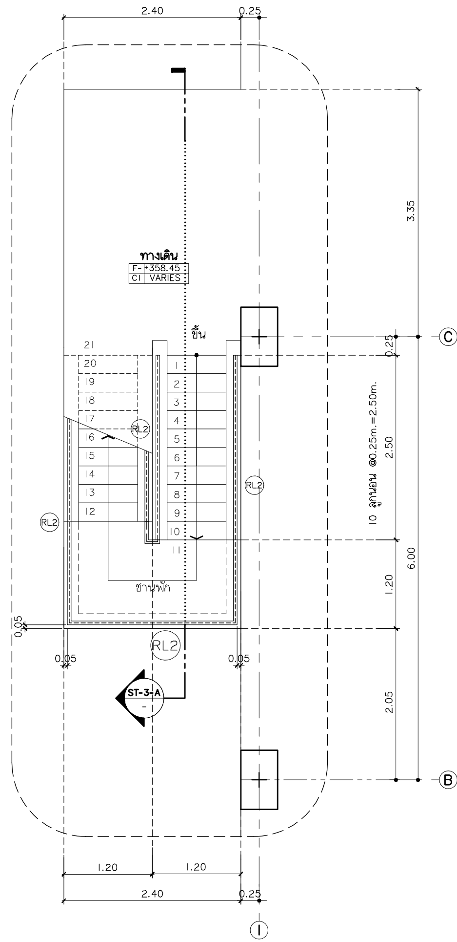
แบบขยายบันได ST-3 ชั้นพื้นดิน มาตราส่วน 1:50
