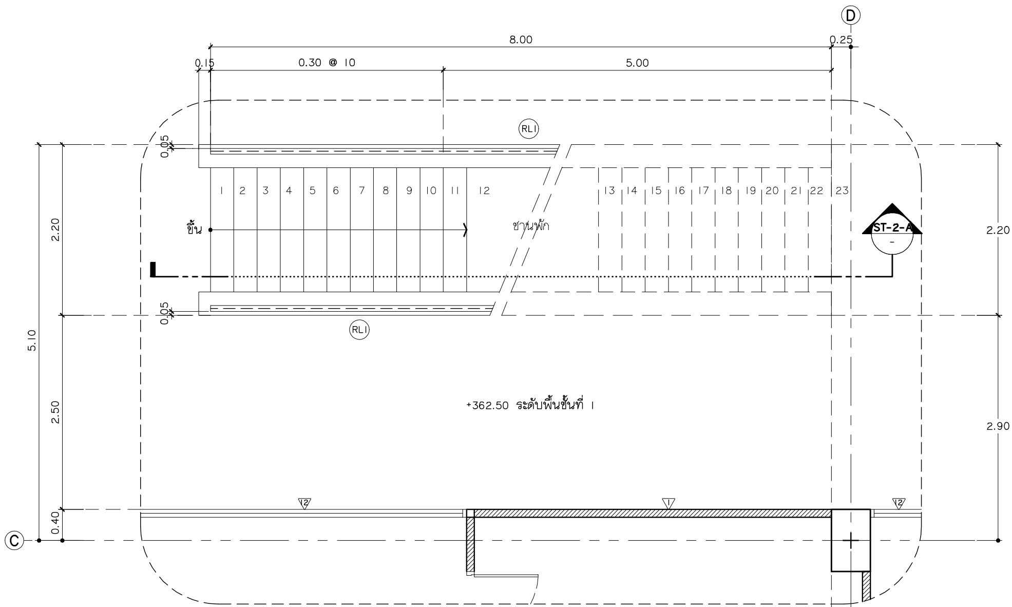
แบบขยายบันได ST-2 ชั้นที่ 1 มาตราส่วน 1:50
