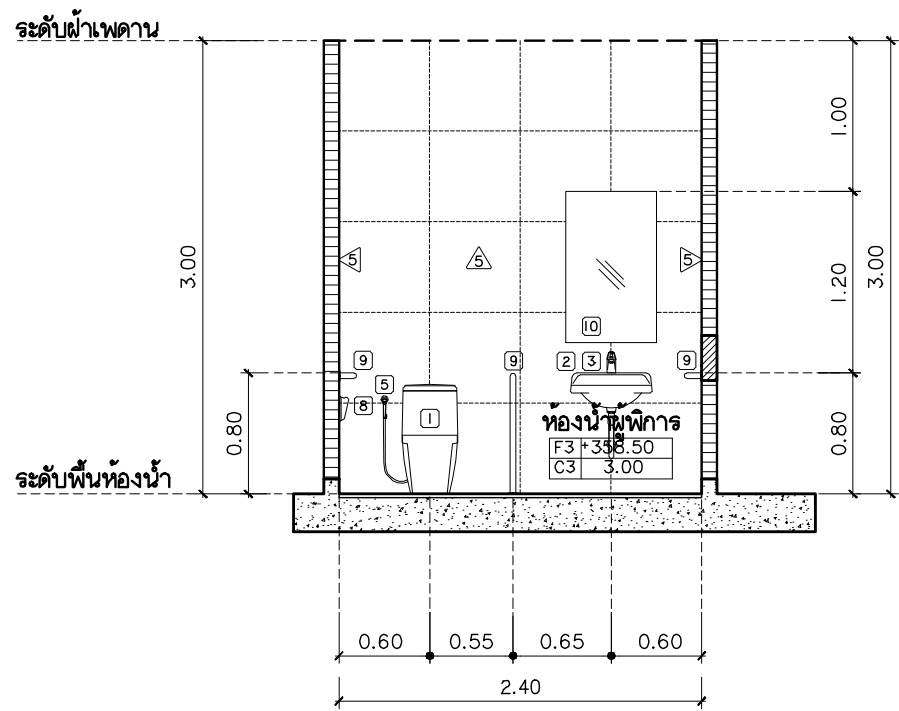
รูปตัด I-A มาตราส่วน 1:50
