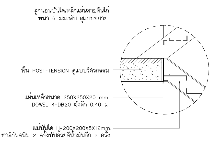
แบบขยาย ST-3-E มาตราส่วน 1:20
