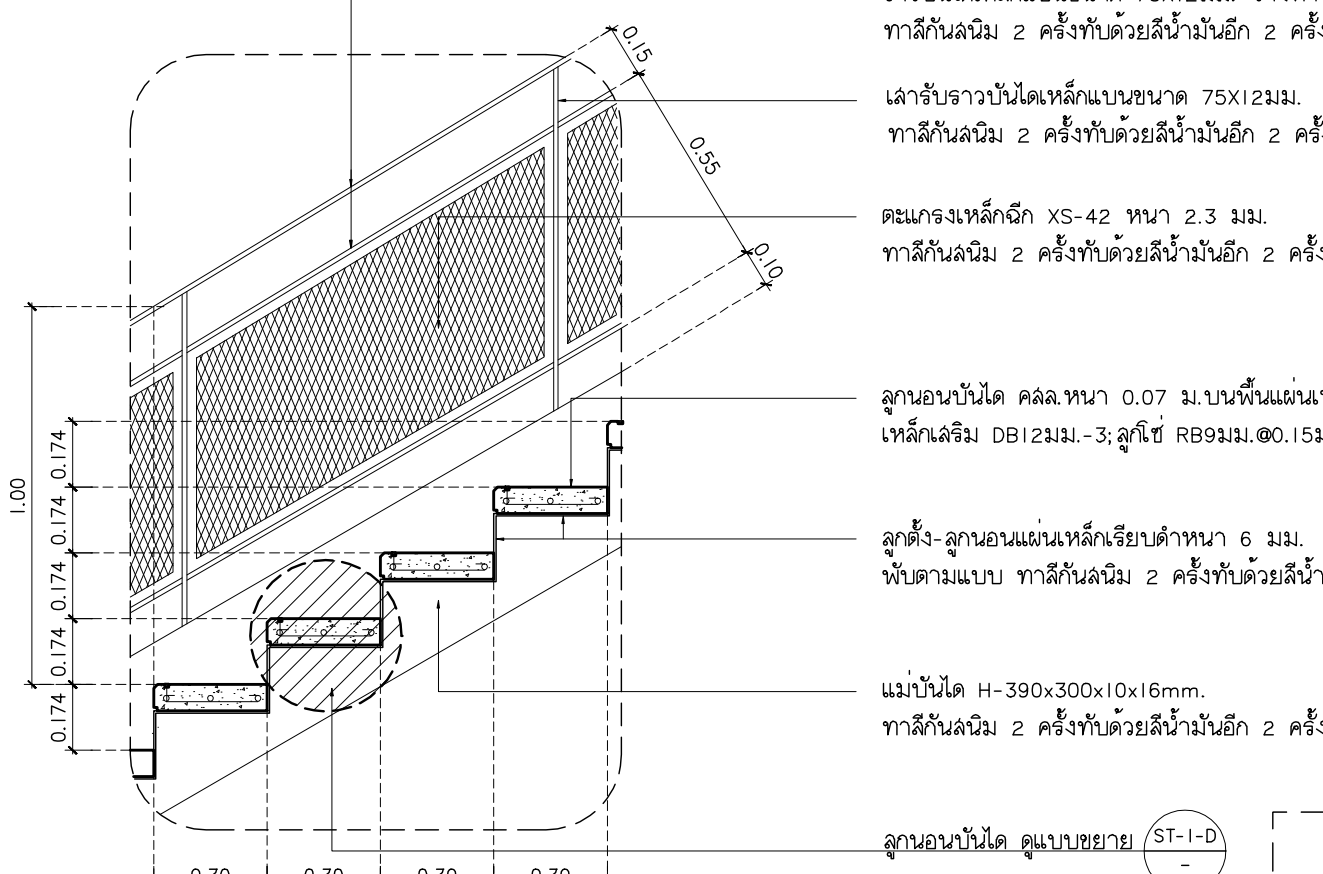
แบบขยายบันได ST-1-C มาตราส่วน 1:20
