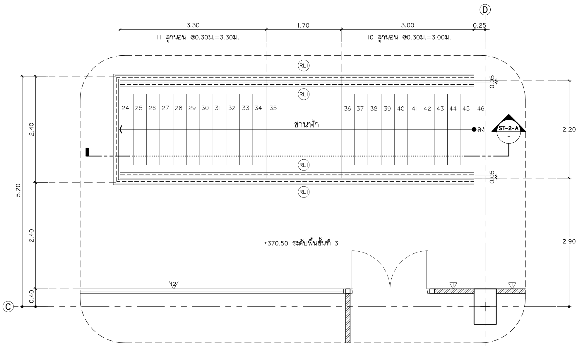
แบบขยายบันได ST-2 ชั้นที่ 3 มาตราส่วน 1:50
