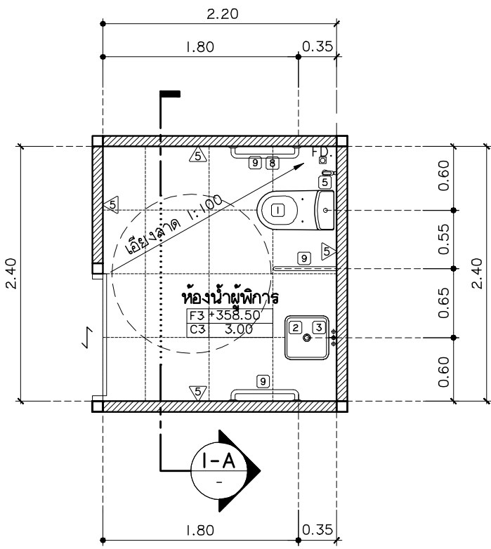
แบบขยายห้องน้ำคนพิการ มาตราส่วน 1:50
