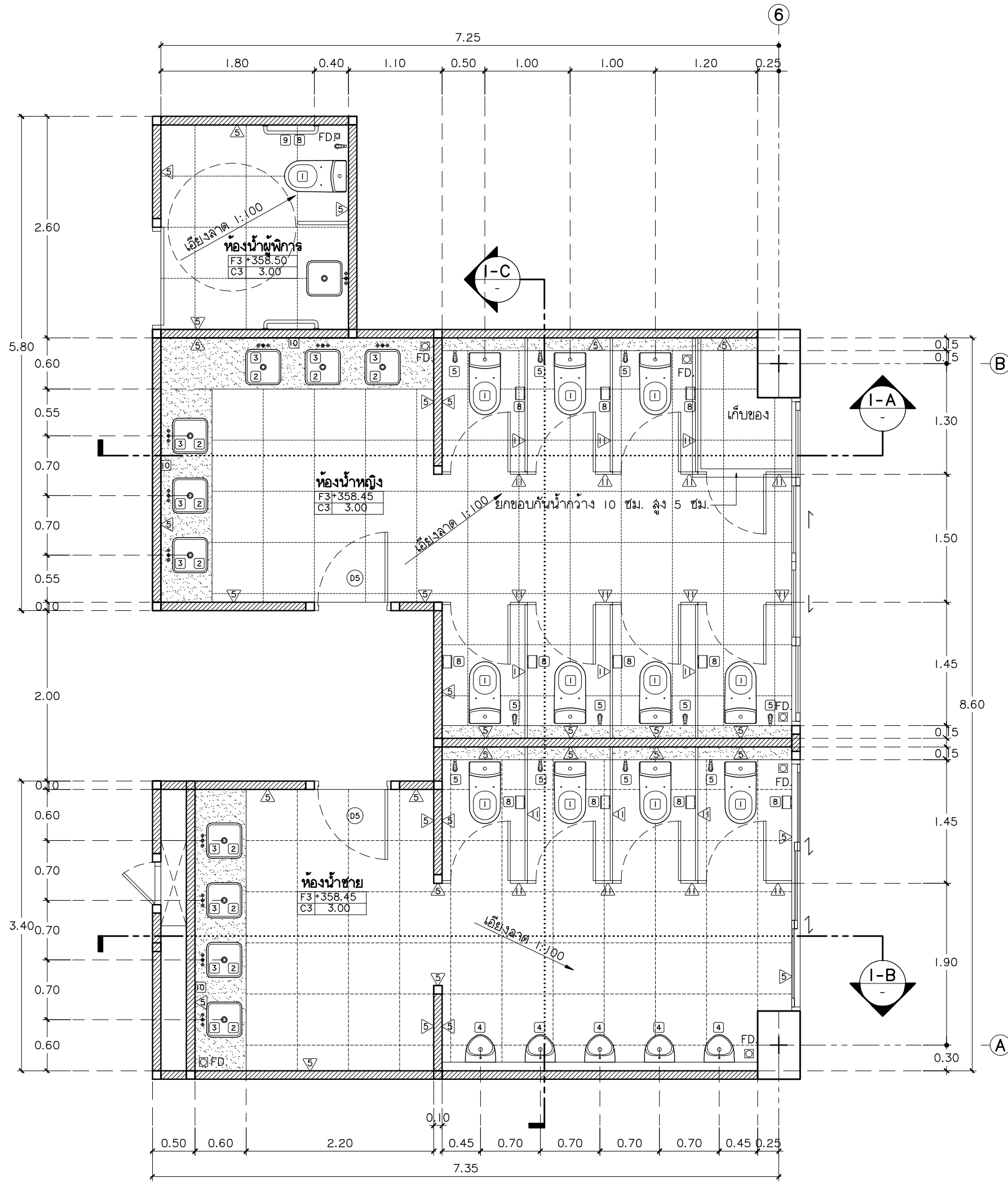
แบบขยายห้องน้ำ ชาย-หญิง มาตราส่วน 1:50
