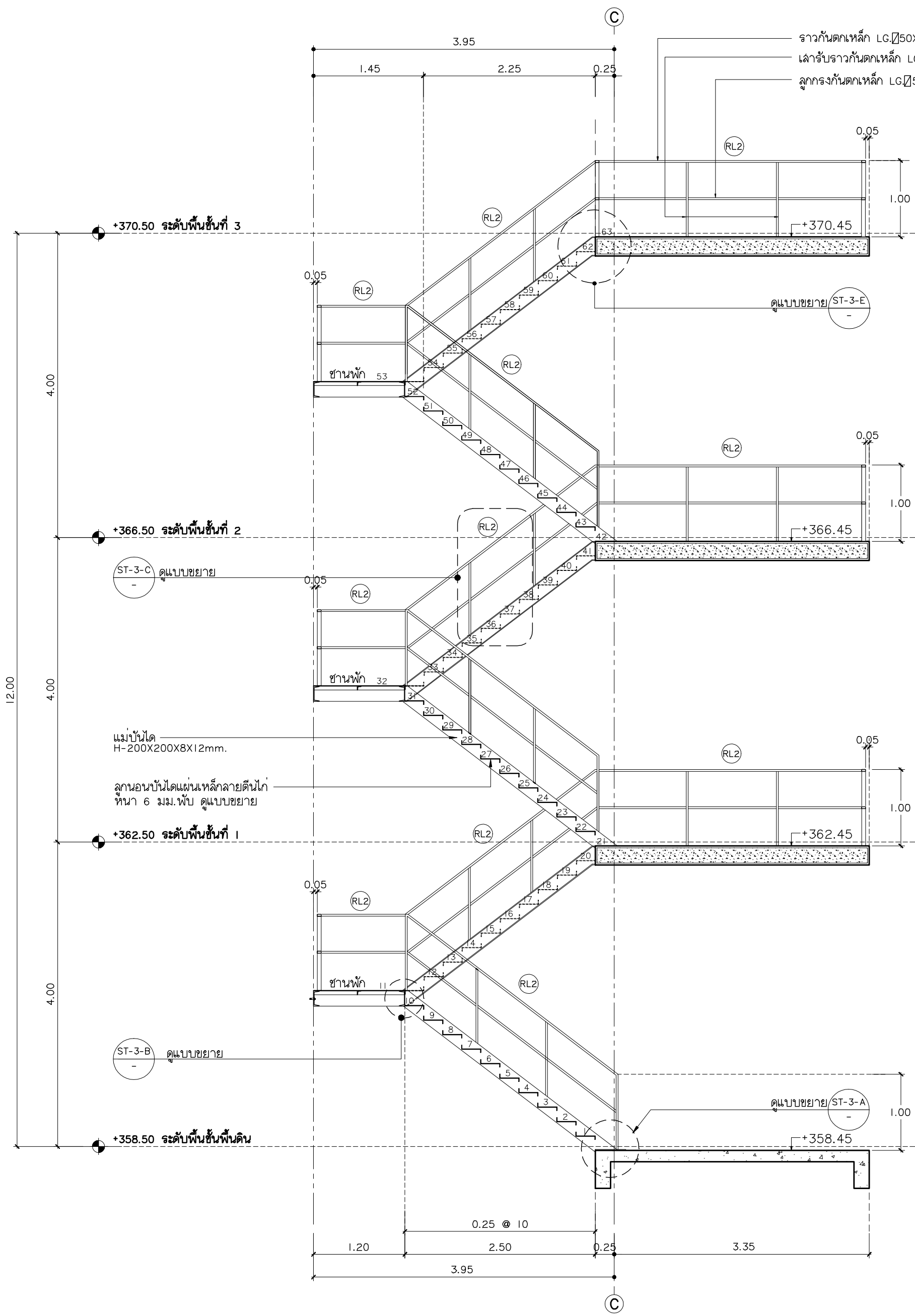
รูปตัด ST-3-A มาตราส่วน 1:50
