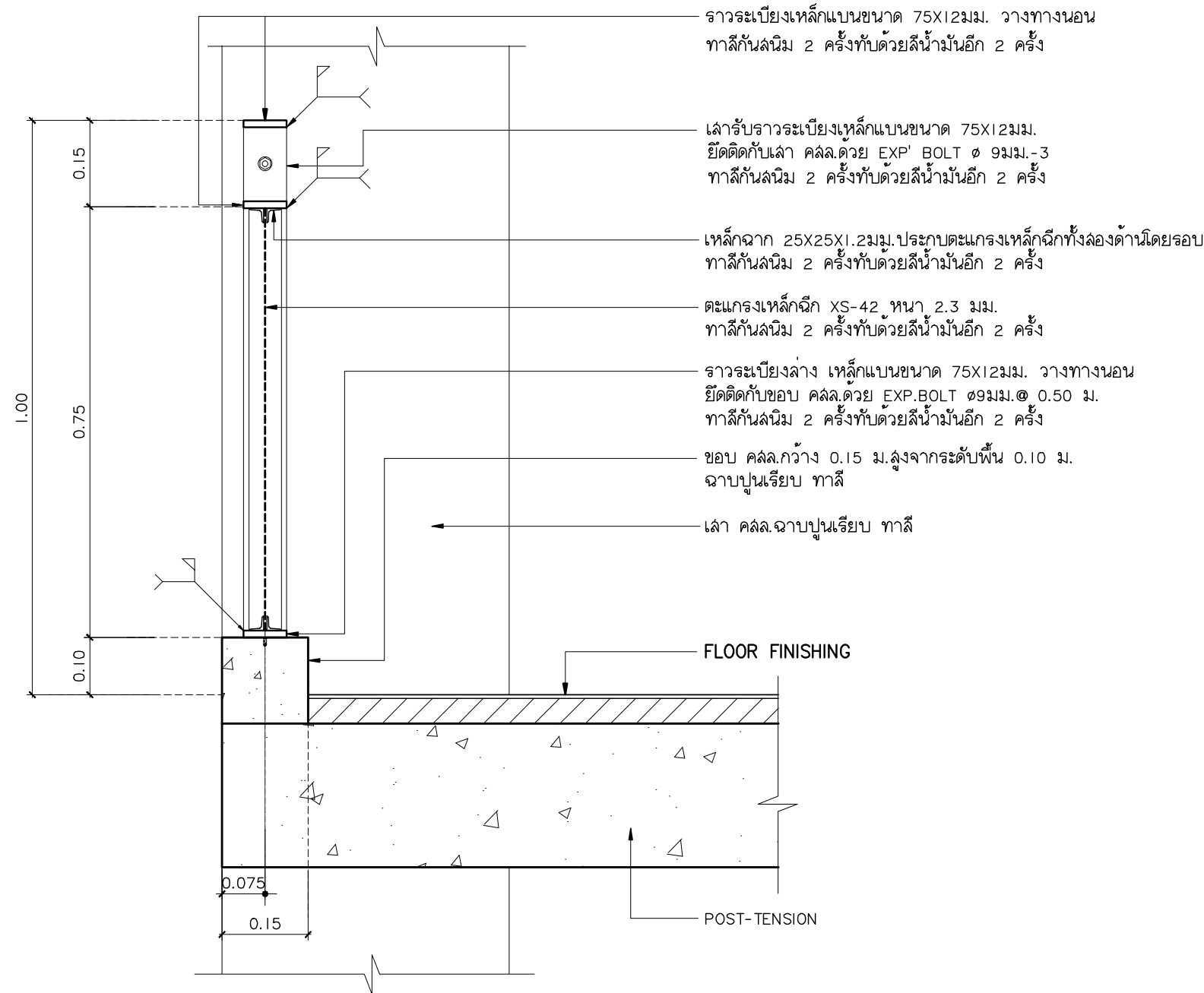
แบบขยายจากระเบียง รูปตัด RLI-A มาตราส่วน 1:10
