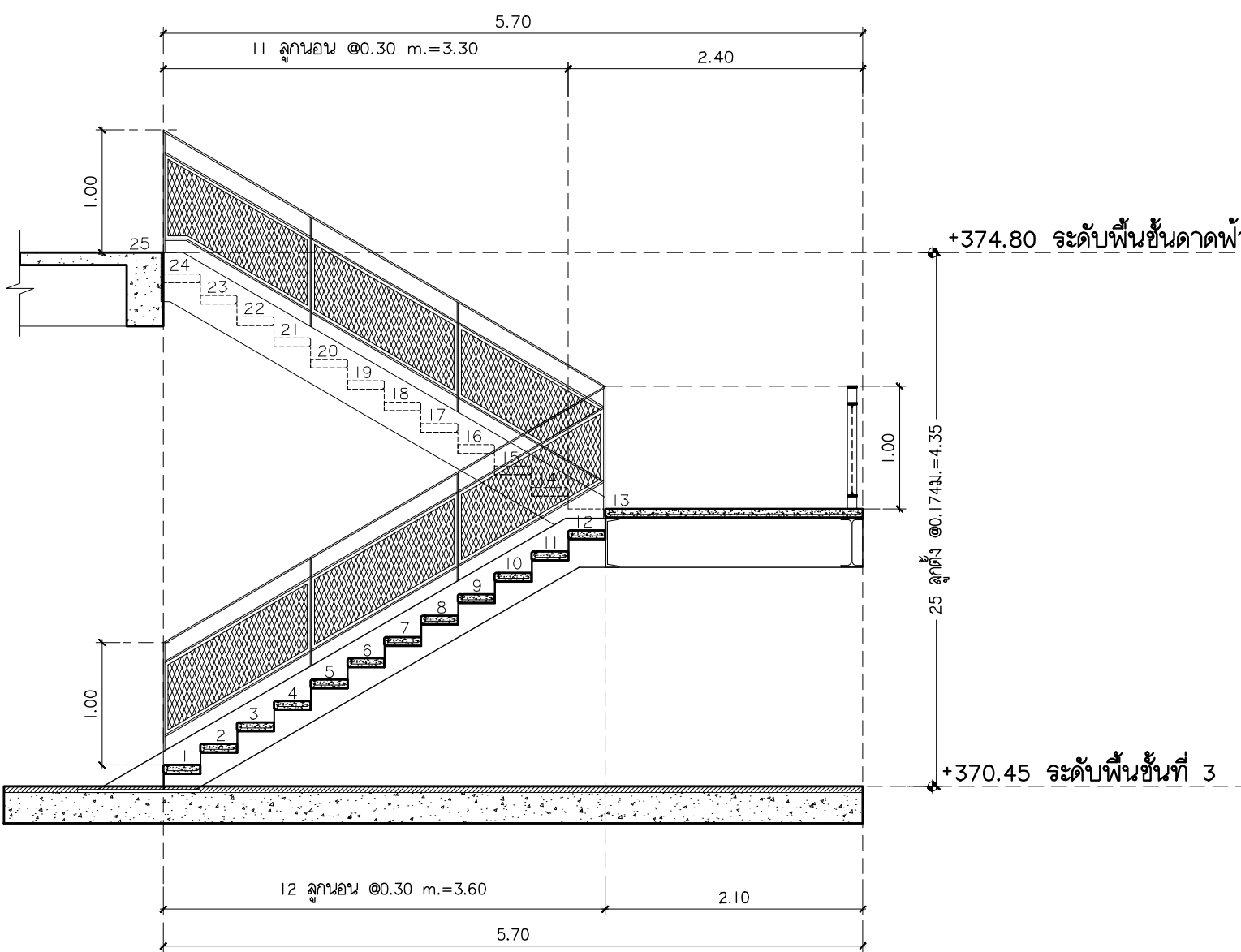
รูปตัด ST-5-A มาตราส่วน 1:50
