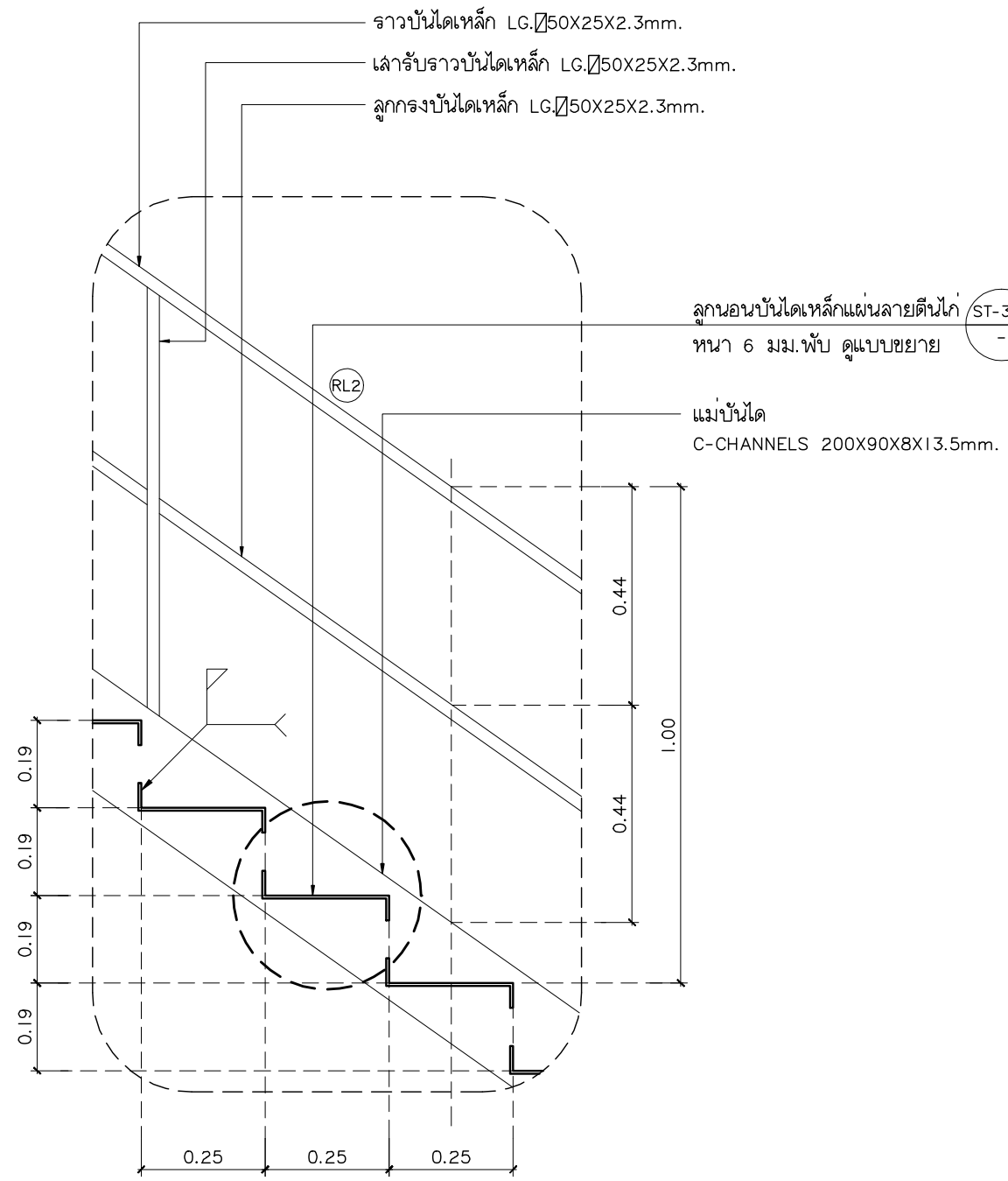
แบบขยาย ST-3-C มาตราส่วน 1:20
