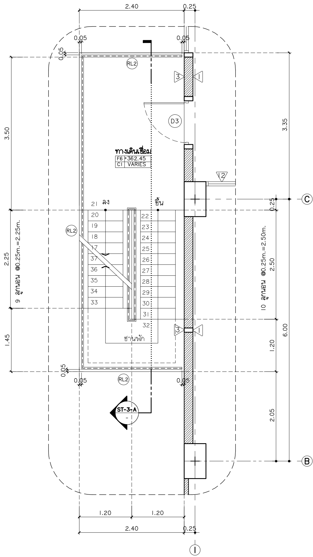
แบบขยายบันได ST-3 ชั้นที่ 1 มาตราส่วน 1:50
