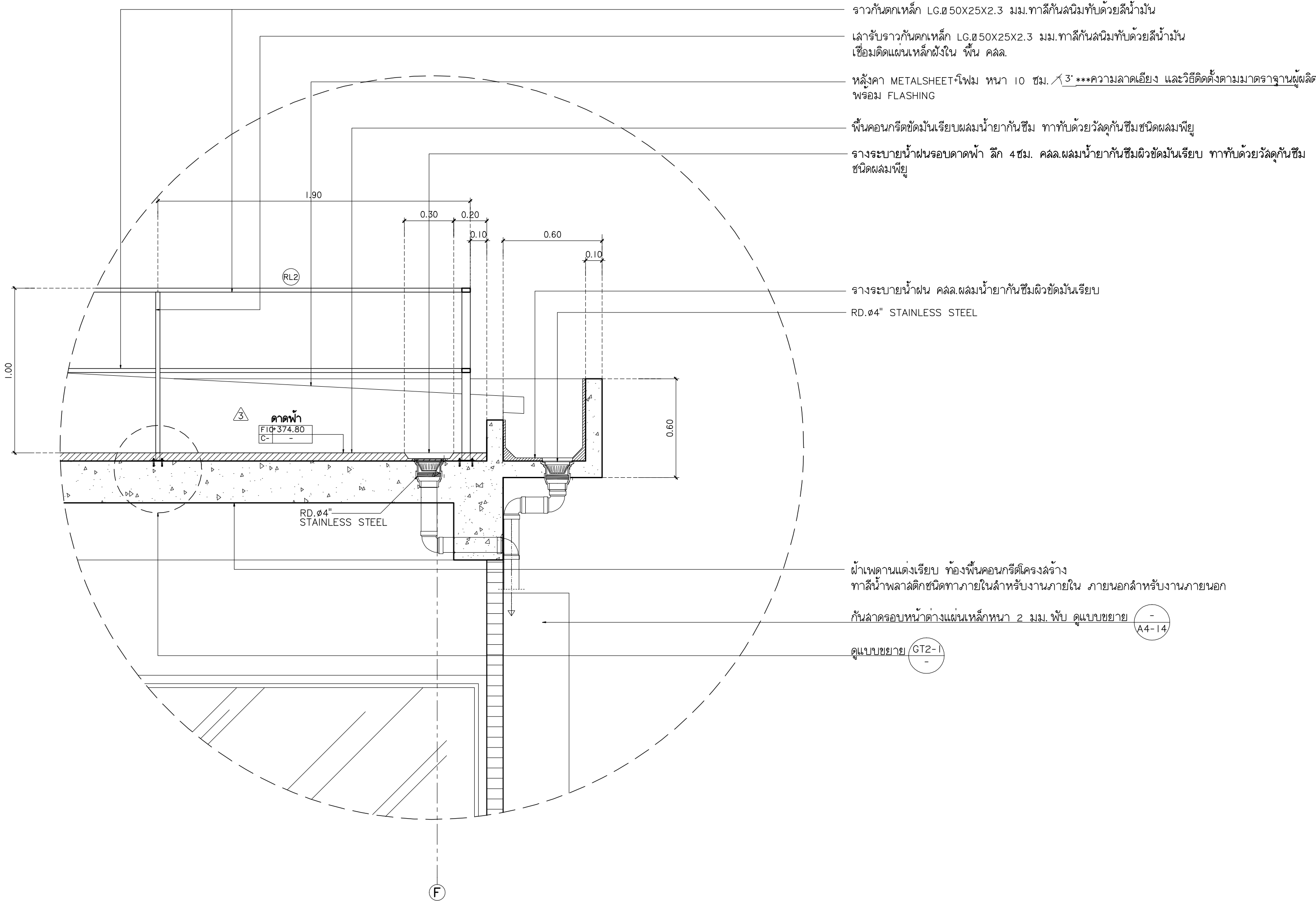
แบบขยาย GT2 มาตราส่วน 1:20
