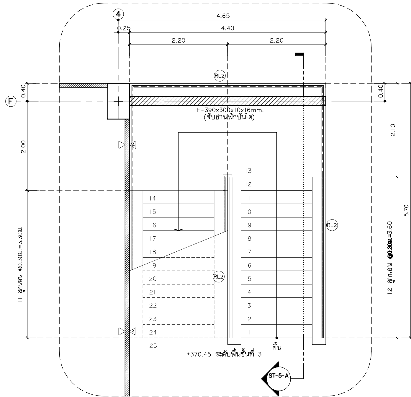
แบบขยายบันได ST-5 ขั้นที่ 3 มาตราส่วน 1:50
