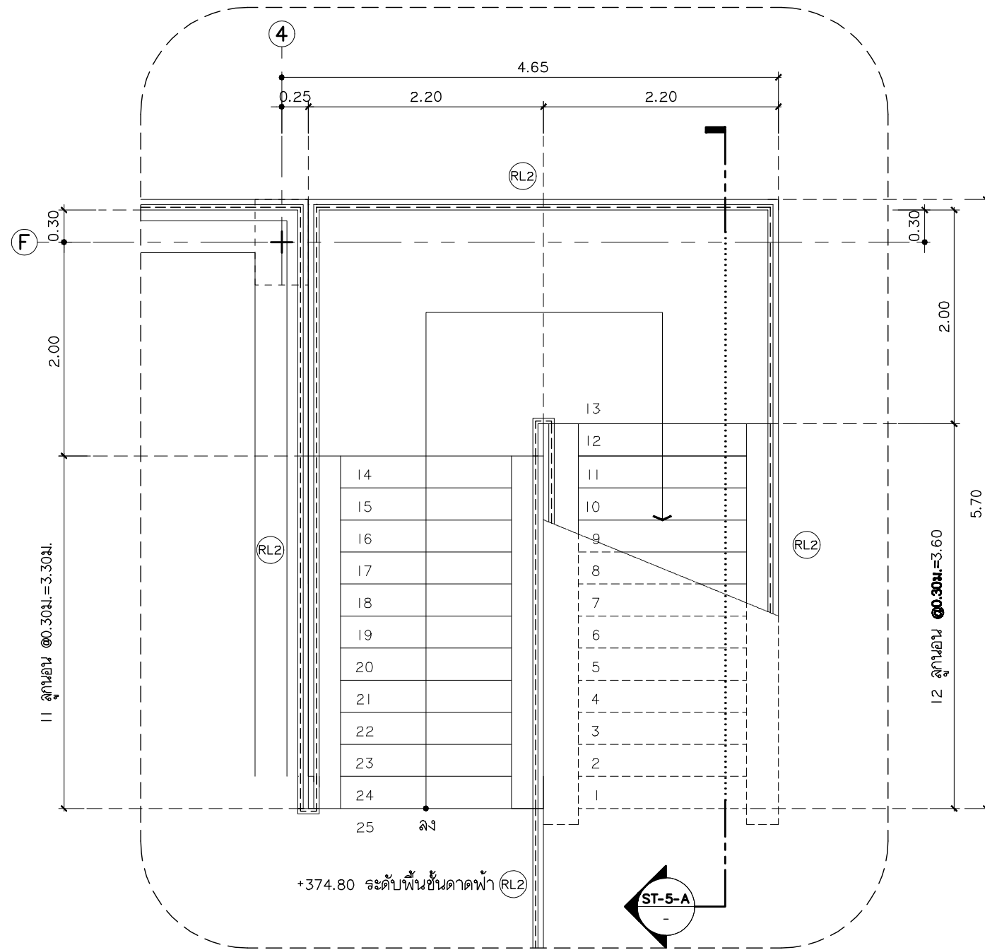
แบบขยายบันได ST-5 ขั้นคานฟ้า มาตราส่วน 1:50
