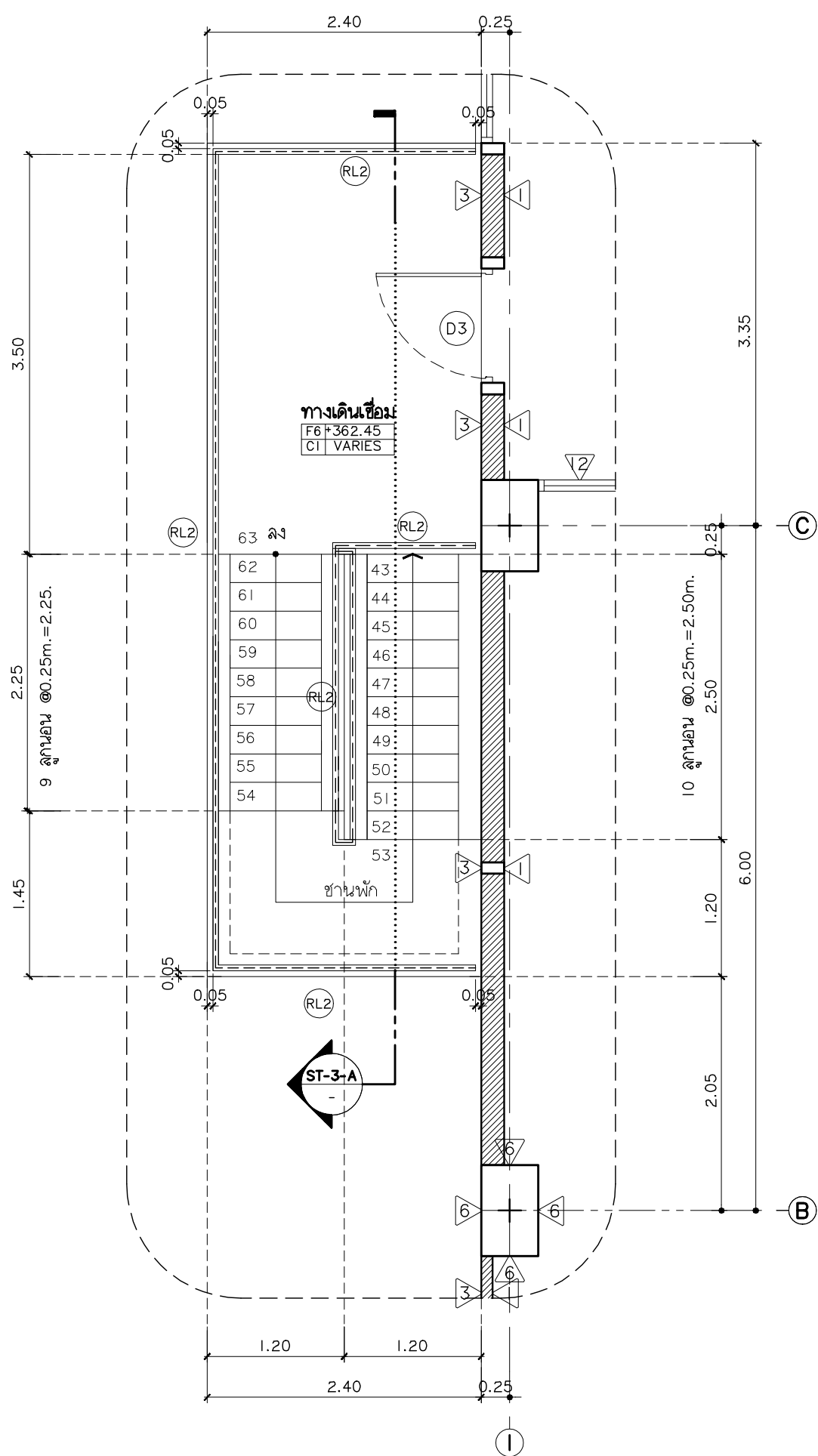
แบบขยายบันได ST-3 ชั้นที่ 3 มาตราส่วน 1:50
