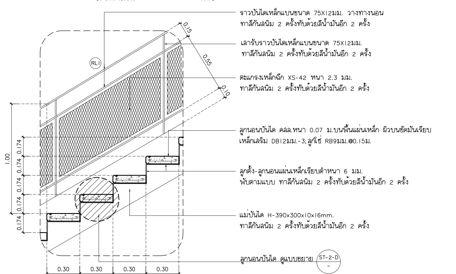
แบบขยายลูกนอนบันได ST-2-C มาตราส่วน 1:20
