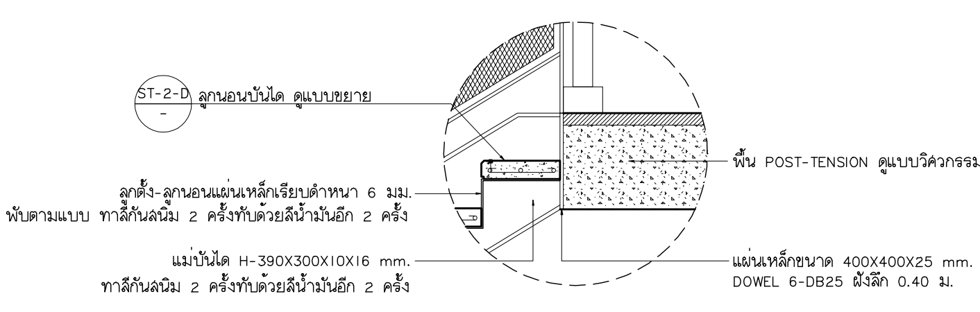
แบบขยาย ST-2-B มาตราส่วน 1:20
