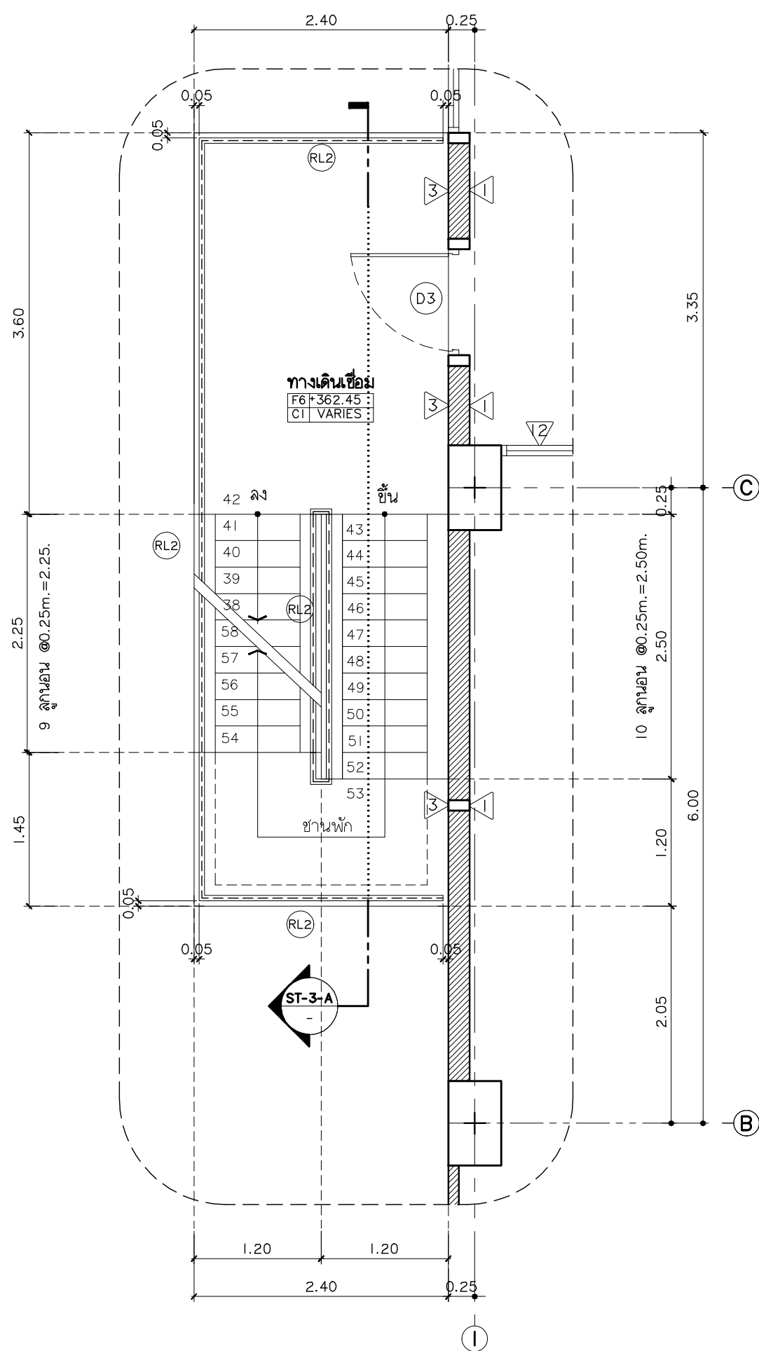
แบบขยายบันได ST-3 ชั้นที่ 2 มาตราส่วน 1:50
