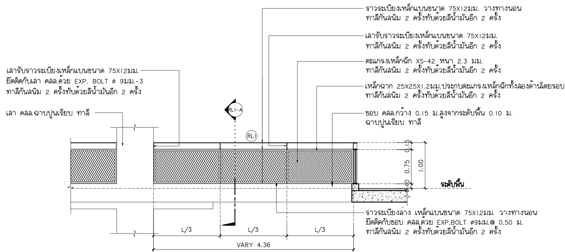
แบบขยายจากระเบียง RLI รูปด้าน มาตราส่วน 1:50
