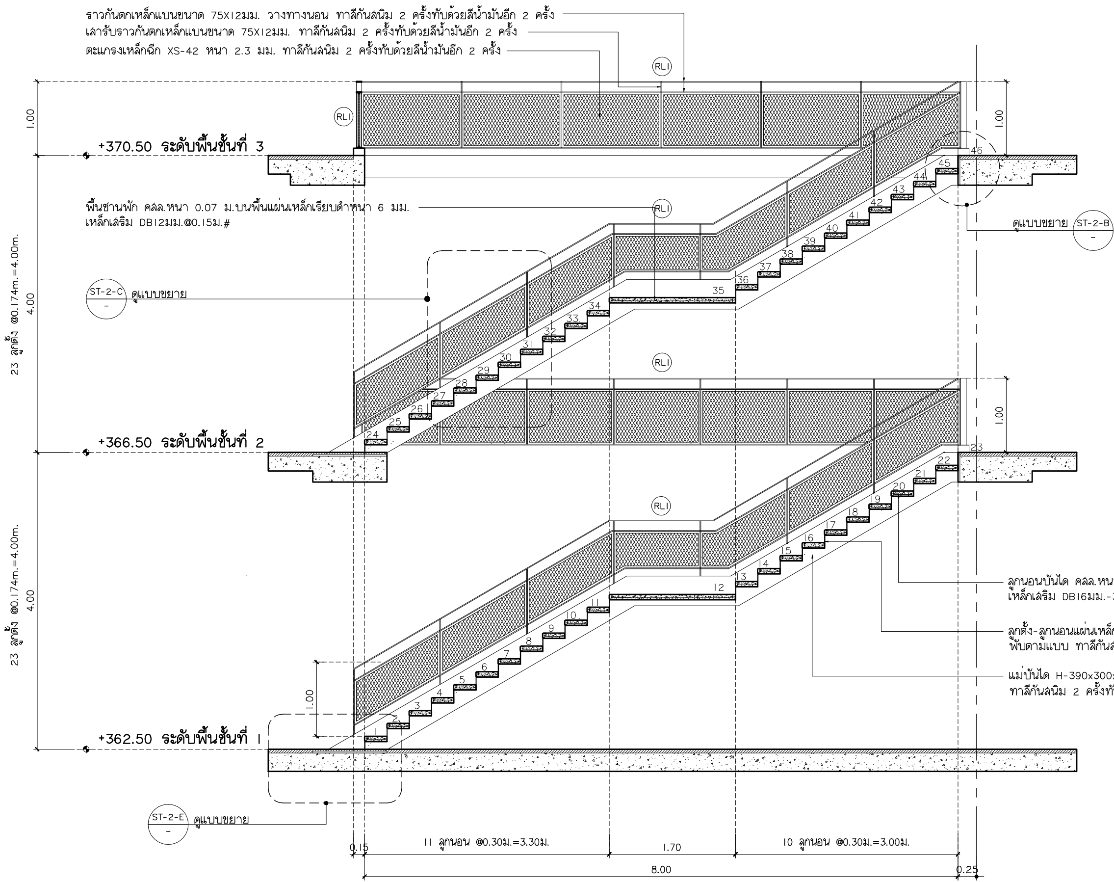
รูปตัด ST-2-A มาตราส่วน 1:50
