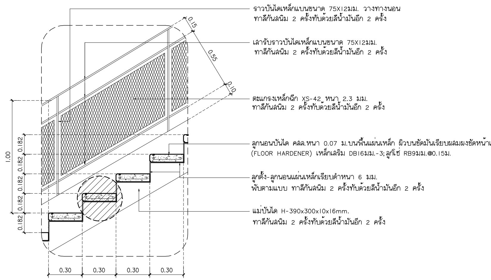
รูปตัด ST-5-A มาตราส่วน 1:50
