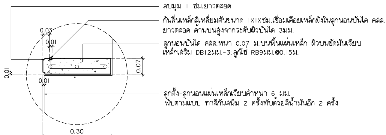
แบบขยาย ST-2-D มาตราส่วน 1:10
