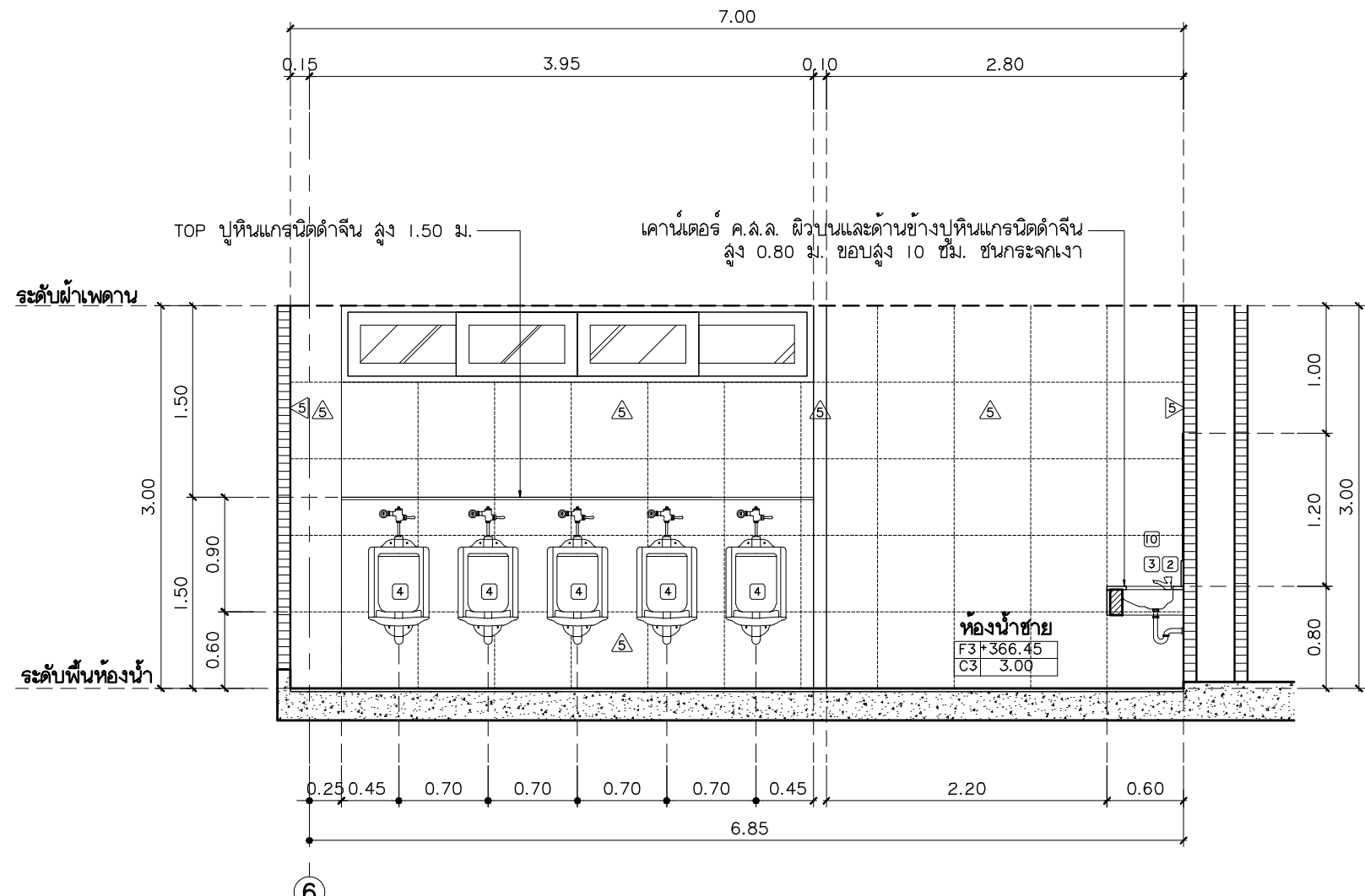
รูปตัด I-B มาตราส่วน 1:50
