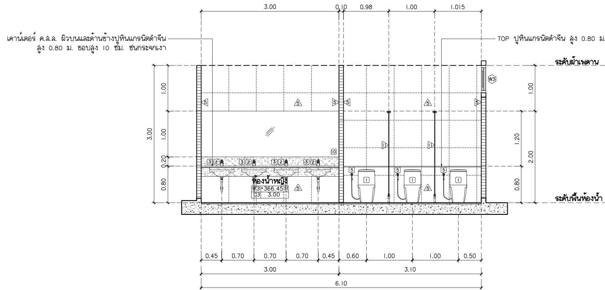
รูปตัด I-A มาตราส่วน 1:50
