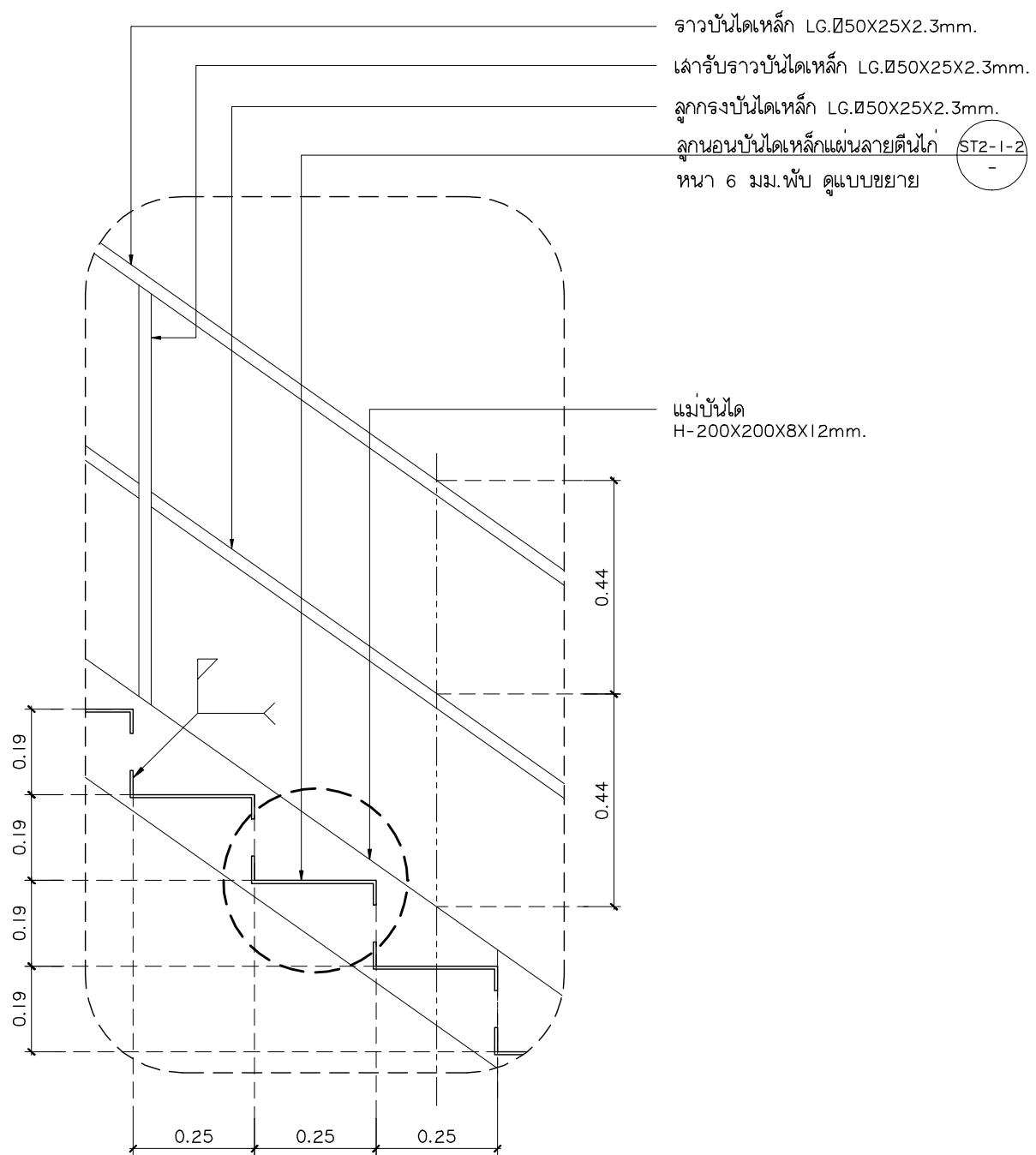
แบบขยาย ST2-1-1 มาตราส่วน 1:20
