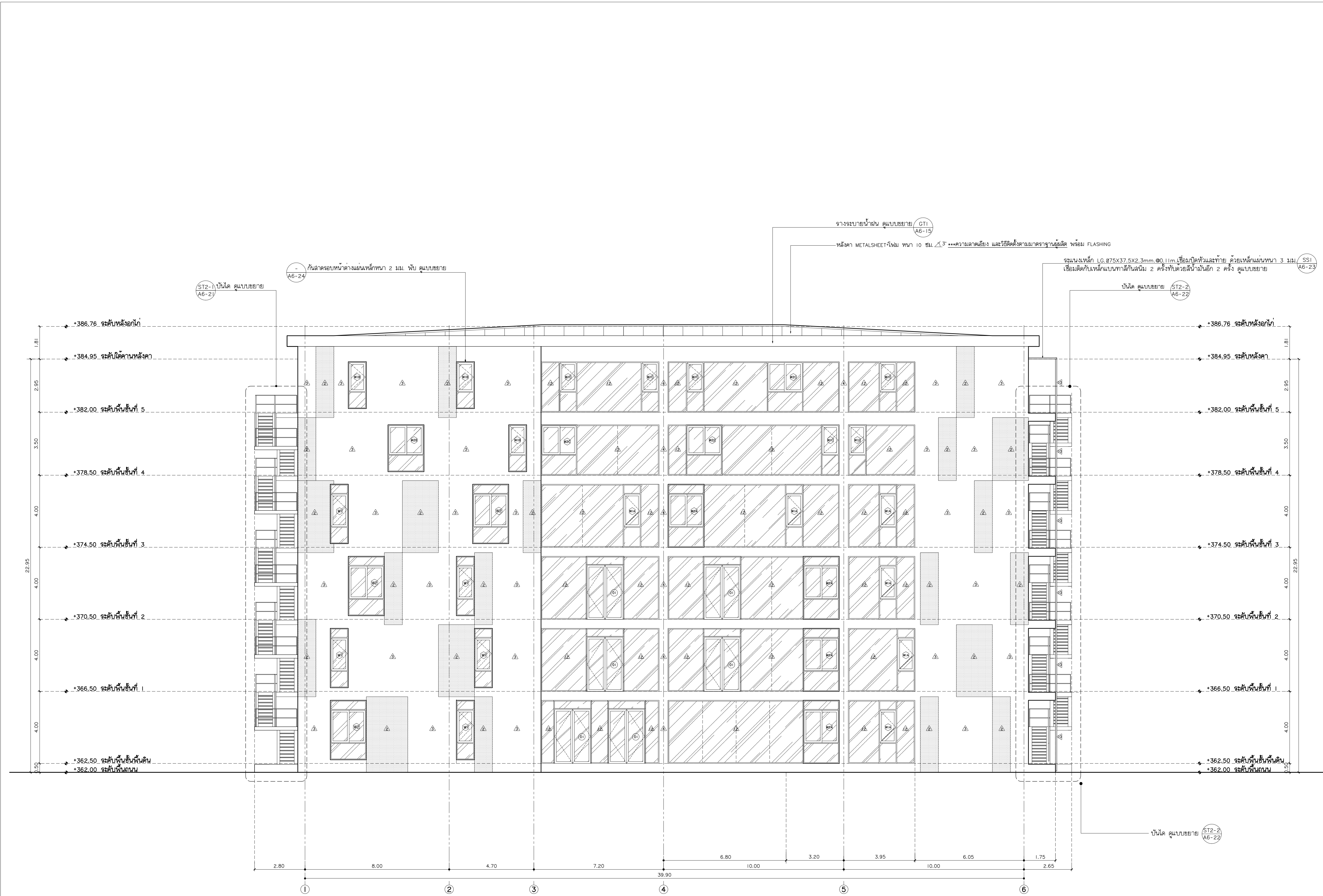
รูปด้าน E1 มาตราส่วน 1:100
