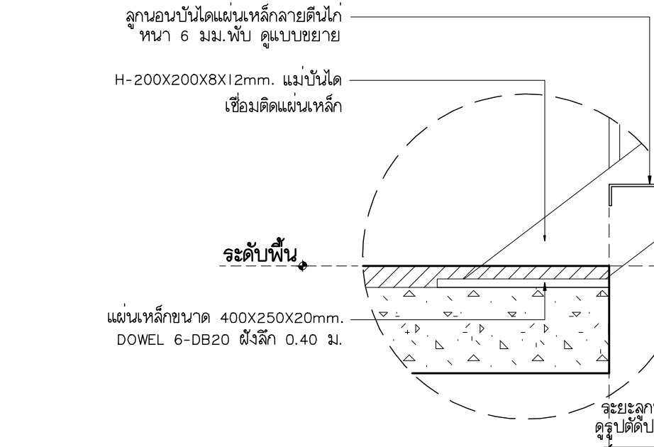
แบบขยายบันได ST2-2 แปลนพื้นที่พื้นดิน มาตราส่วน 1:50
