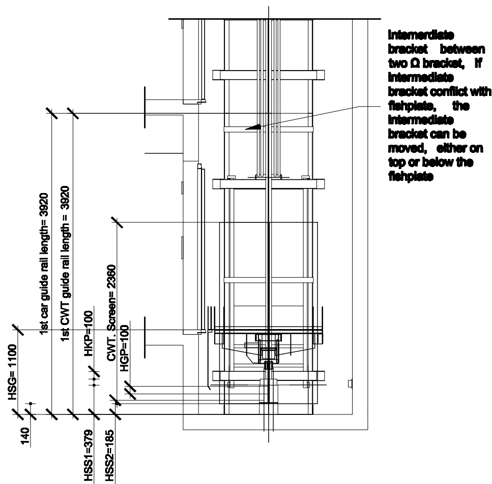
แบบขยาย LTI-A-1 มาตราส่วน 1:25
