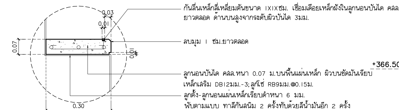
แบบขยาย ST-1-D มาตราส่วน 1:10
