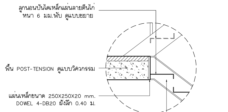
พื้น POST-TENSION สลับริดจิ้ง แผ่นเหล็กขนาด 250x250x20 mm. DOWEL 4-DB20 เส้นผ่า 0.40 ม.
