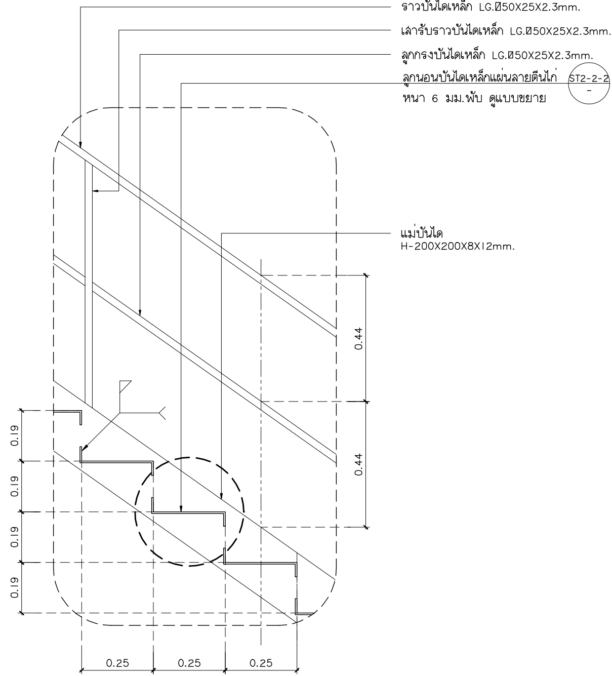
แบบขยาย ST2-2-1 มาตราส่วน 1:20
