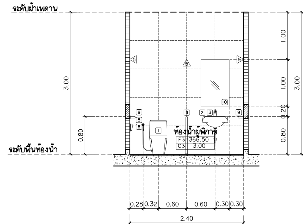
รูปตัด 2-A มาตราส่วน 1:50
