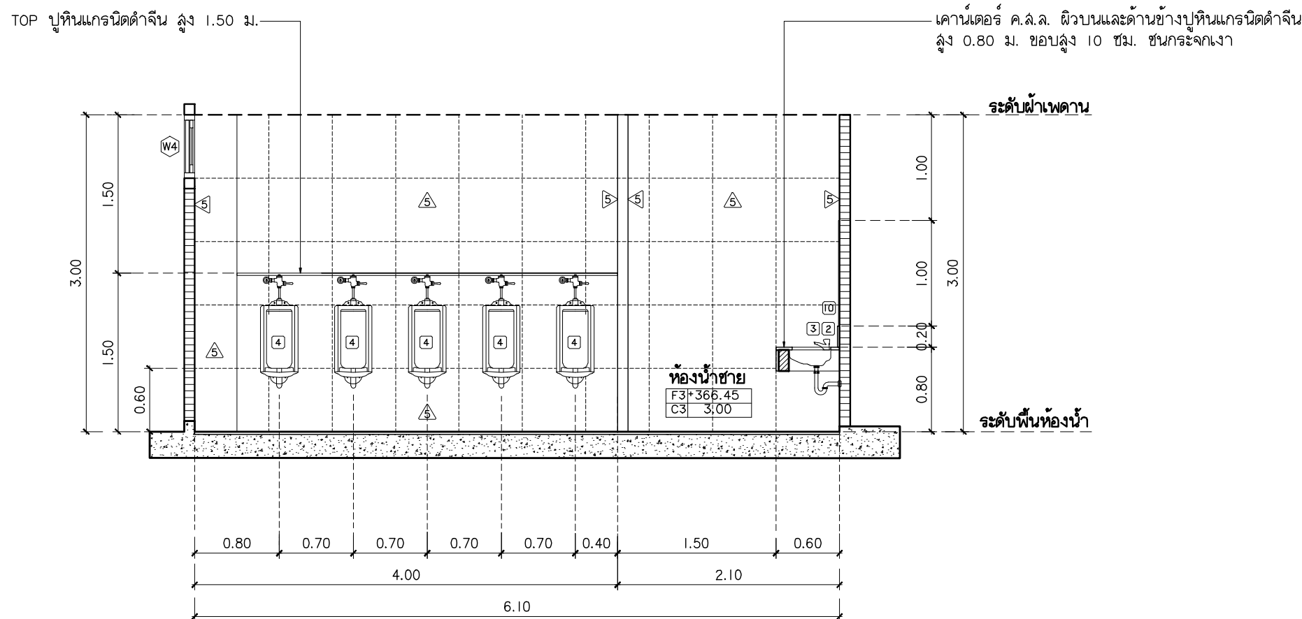
รูปตัด I-B มาตราส่วน 1:50
