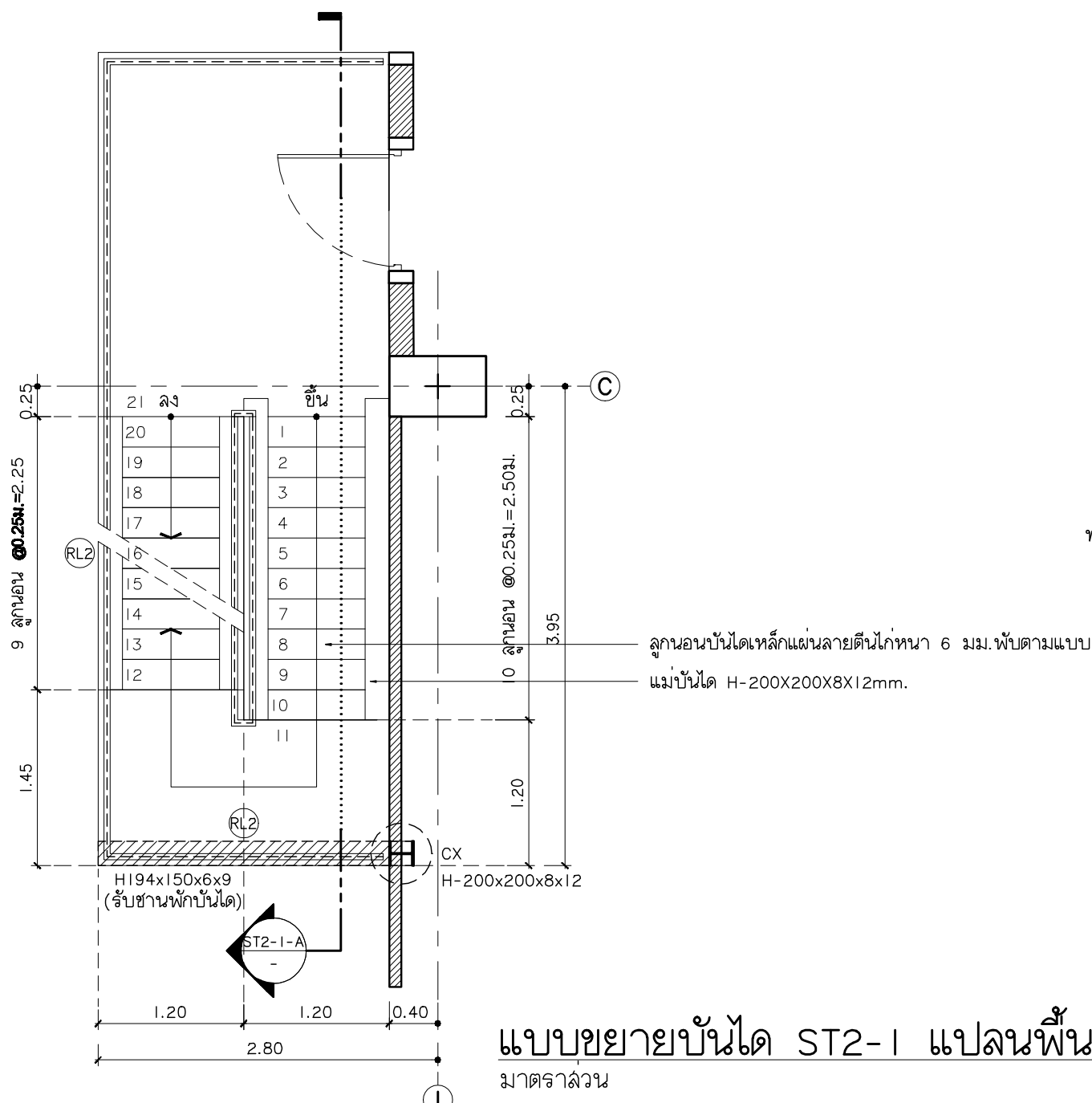
แบบขยายบันได ST2-1 แปลนพื้นที่ 4-5 มาตราส่วน 1:50
