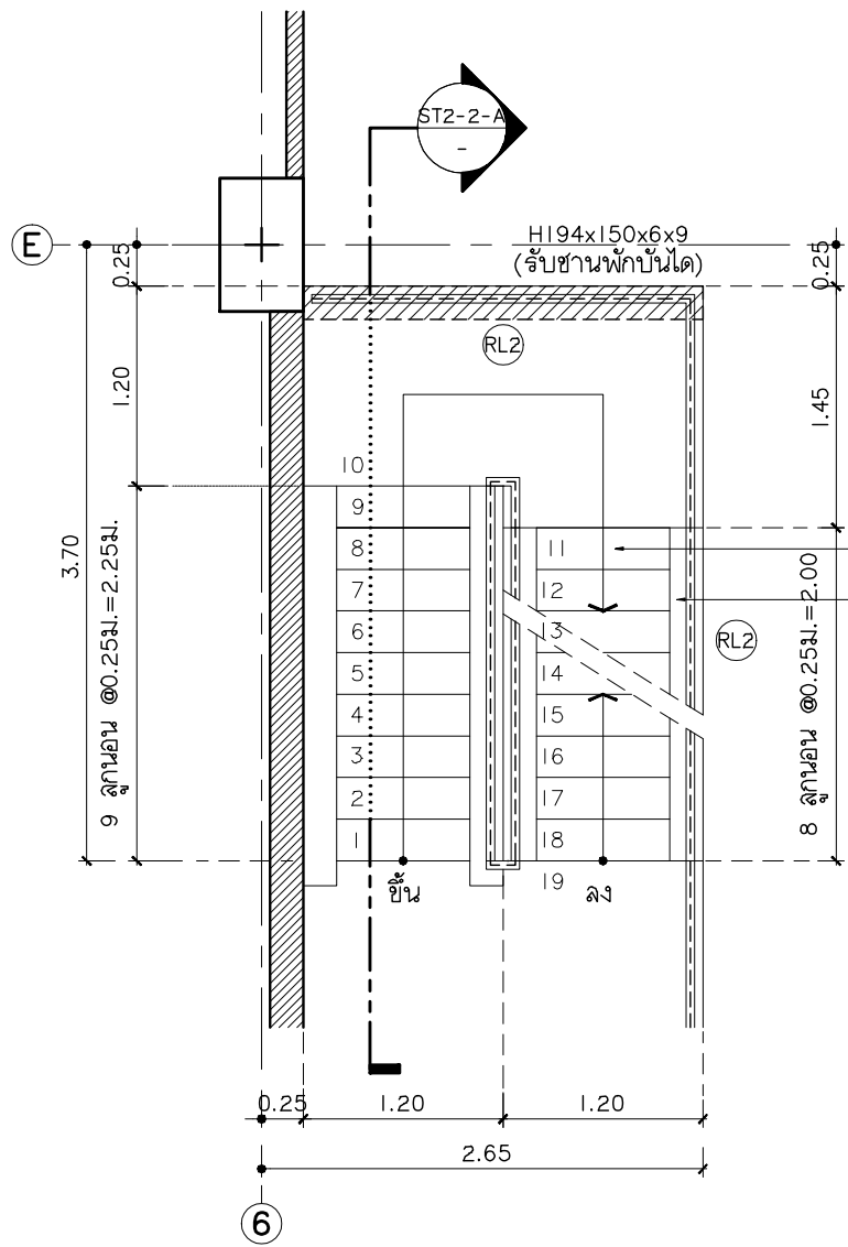
แบบขยายบันได ST2-2 แปลนพื้นที่ 4-5 มาตราส่วน 1:50
