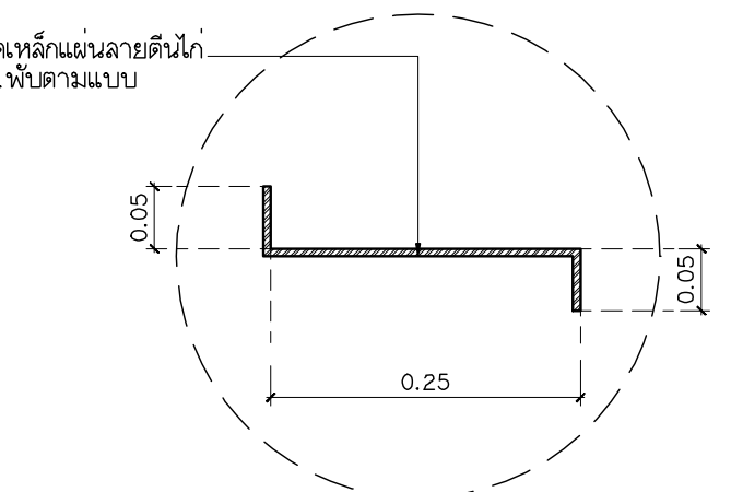
แบบขยาย ST2-2-2 มาตราส่วน 1:20
