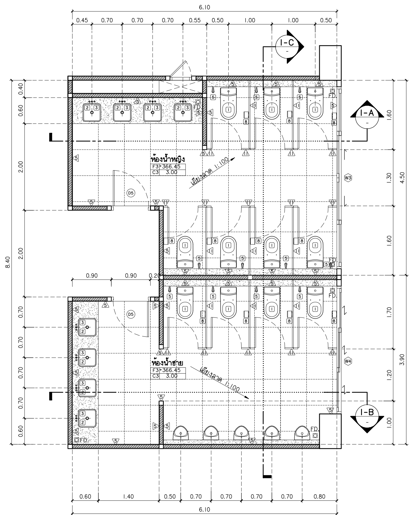
แบบขยายห้องน้ำ ชาย - หญิง มาตราส่วน 1:50
