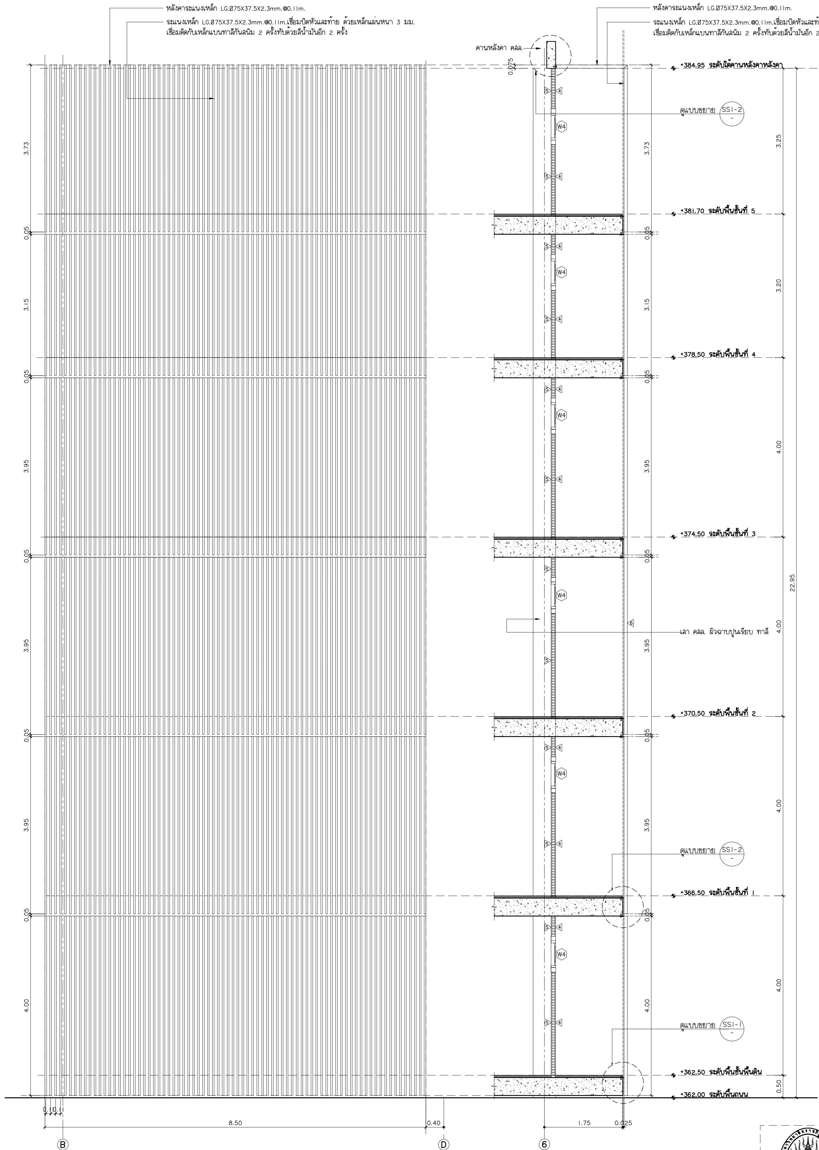
แบบขยาย SSI รูปด้าน I มาตราส่วน 1:50
