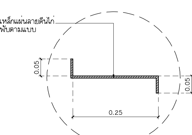
แบบขยาย ST2-1-2 มาตราส่วน 1:20
