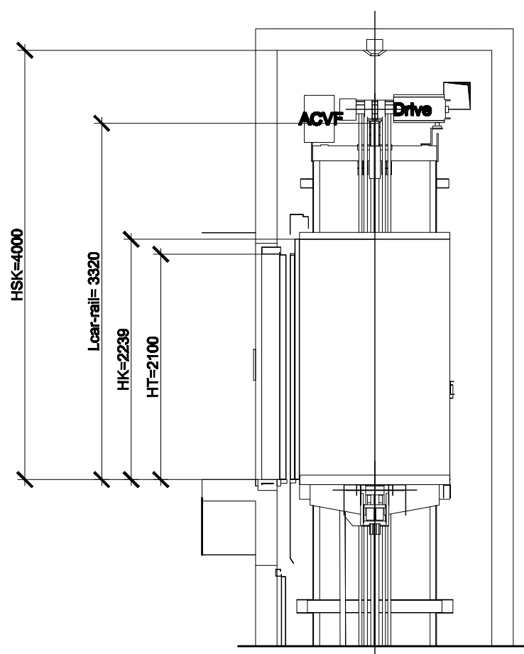
แบบขยาย LTI-A-2 มาตรา ๖๖ 1:25
