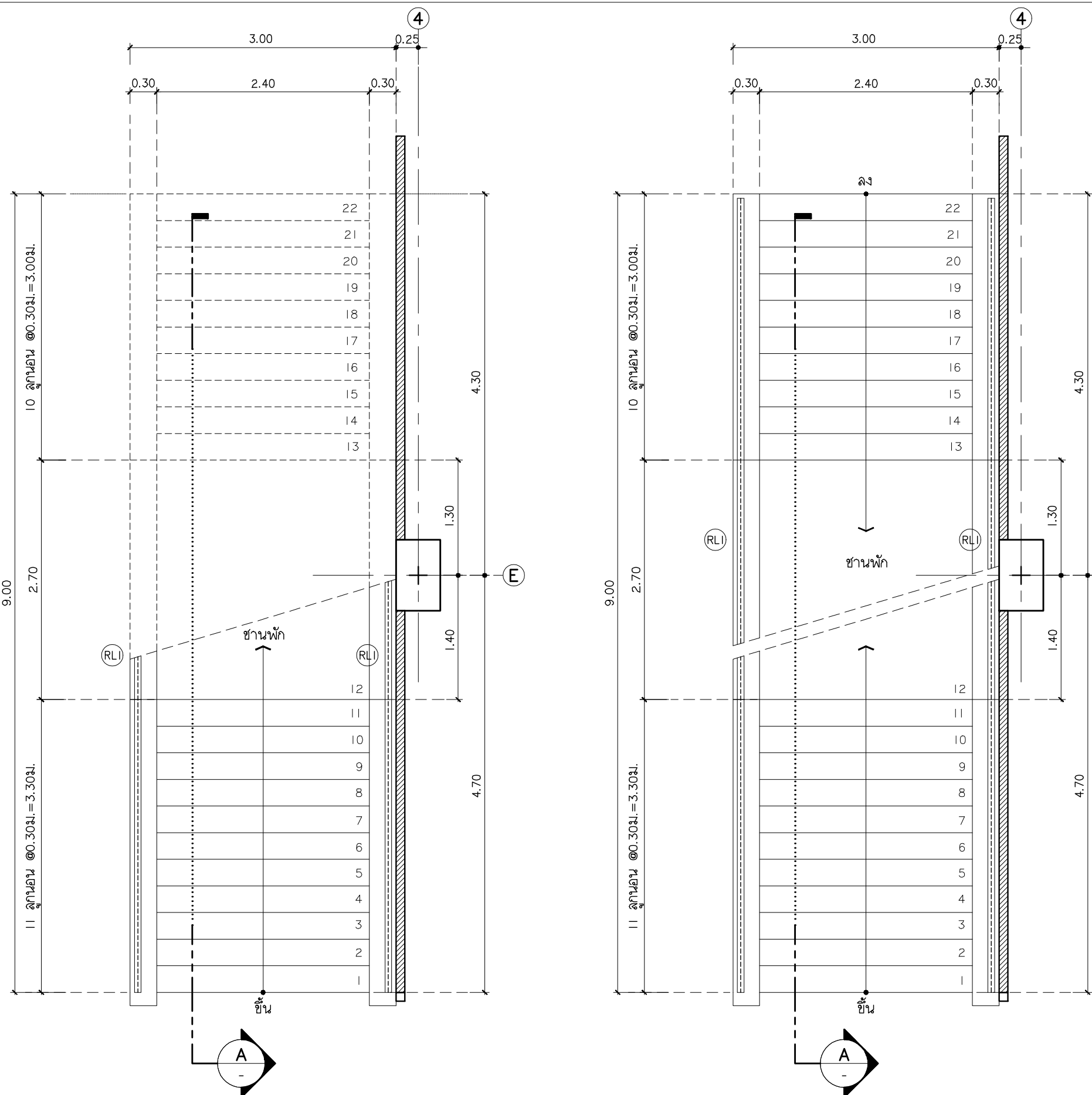
แบบขยายบันได ST-1 ชั้นพื้นดิน มาตราส่วน 1:50
