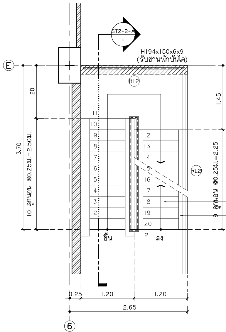
แบบขยายบันได ST2-2 แปลนพื้นที่ 1 - ชั้นที่ 3 มาตราส่วน 1:50
