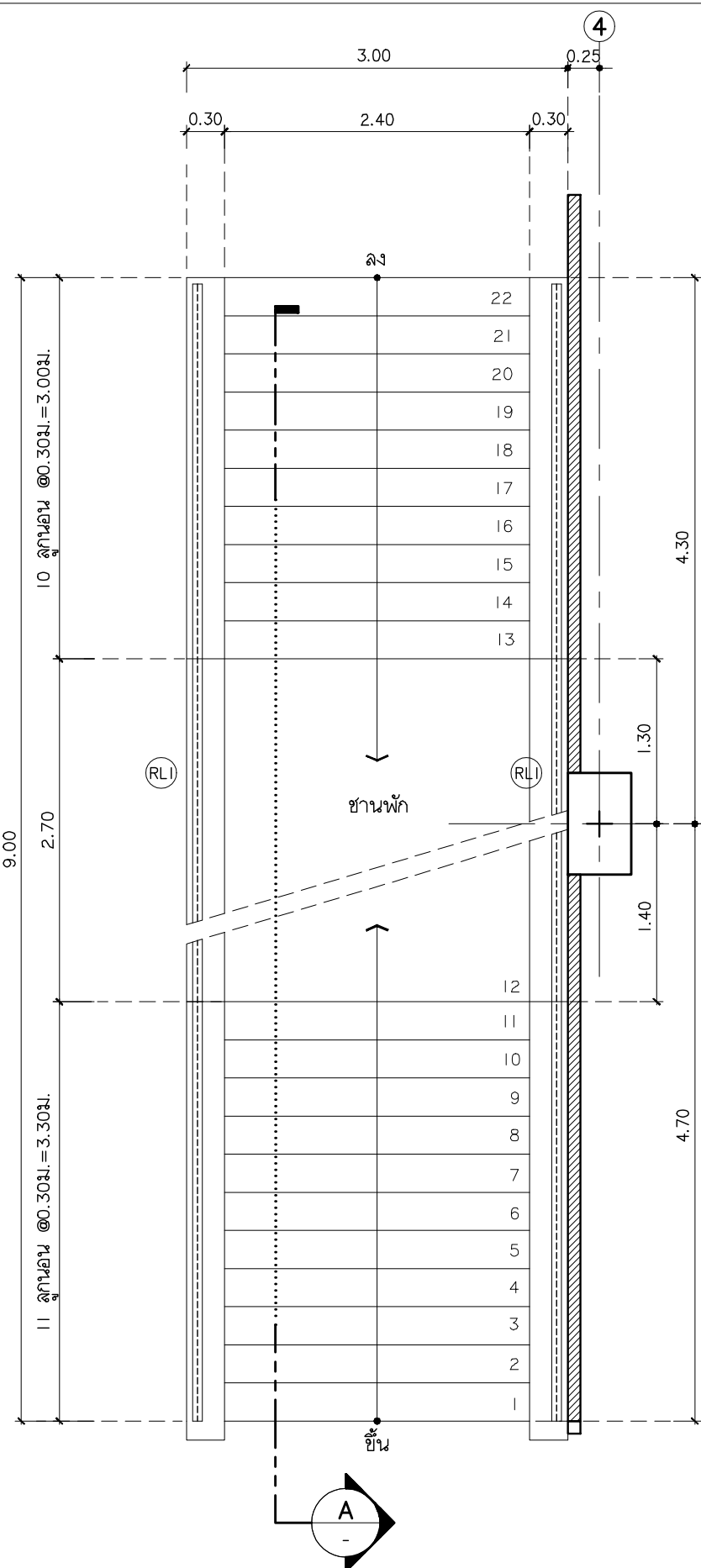
แบบขยายบันได ST-1 ชั้นที่ 1-3 มาตราส่วน 1:50
