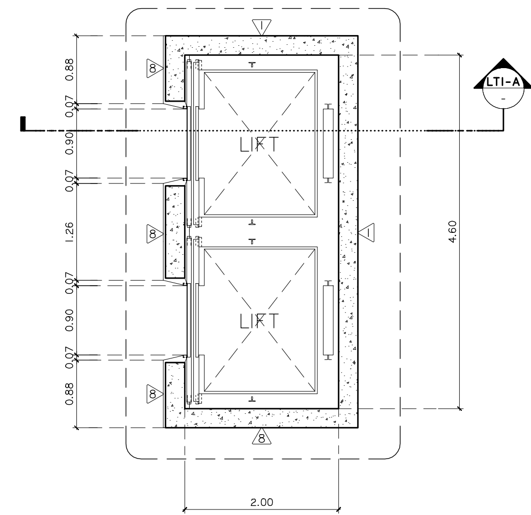
แบบขยายช่องลิฟท์ LTI แปลน มาตราส่วน 1:50
