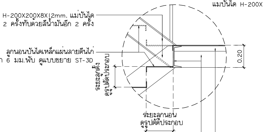
บันไดขึ้นลง จะระลอบ รูปตัดประกอบ
