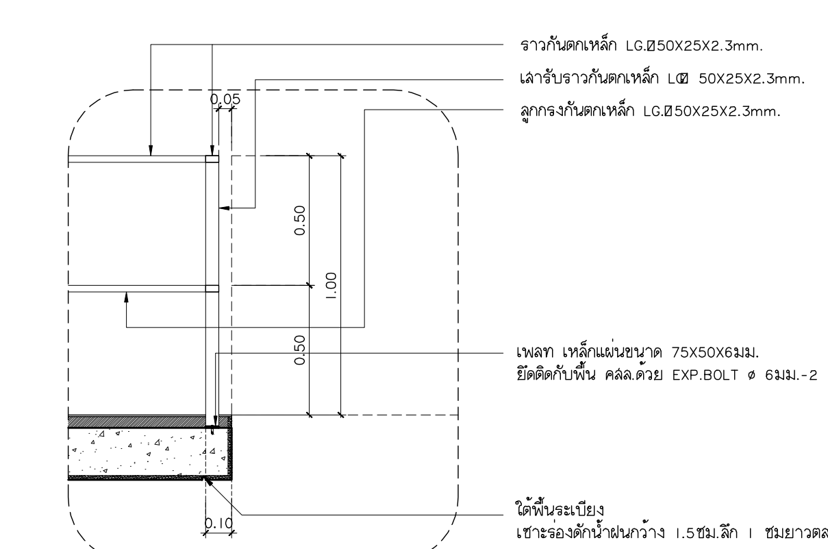
แบบขยาย RL2 มาตราส่วน 1:20
