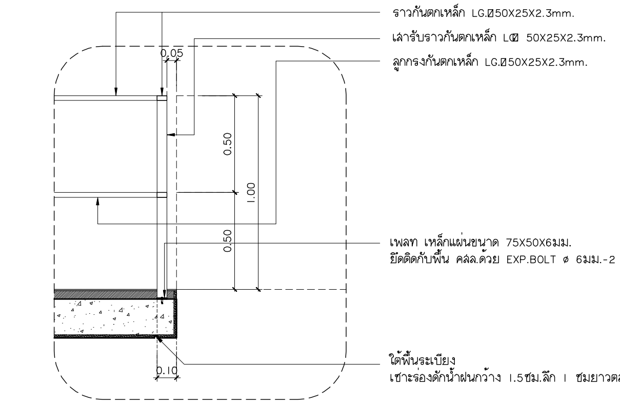
แบบขยาย RL2 มาตราส่วน 1:20
