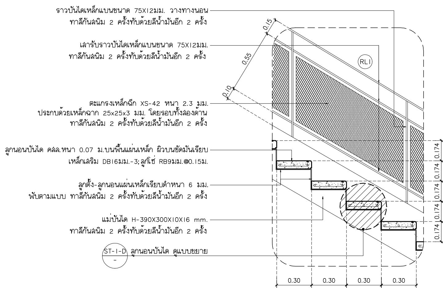
แบบขยายลูกนอนบันได ST-I-C มาตราส่วน 1:20
