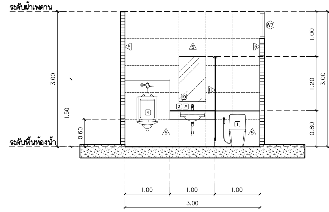
รูปตัด 2-A มาตราส่วน 1:50
