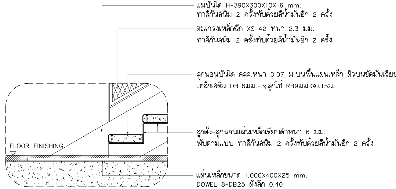
แบบขยาย ST-I-E มาตราส่วน 1:10
