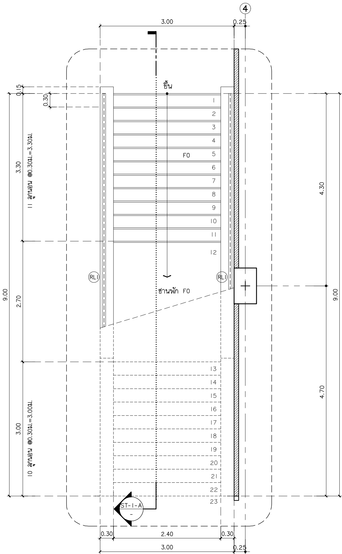
แบบขยายบันได ST-I ชั้นพื้นดิน มาตราส่วน 1:50
