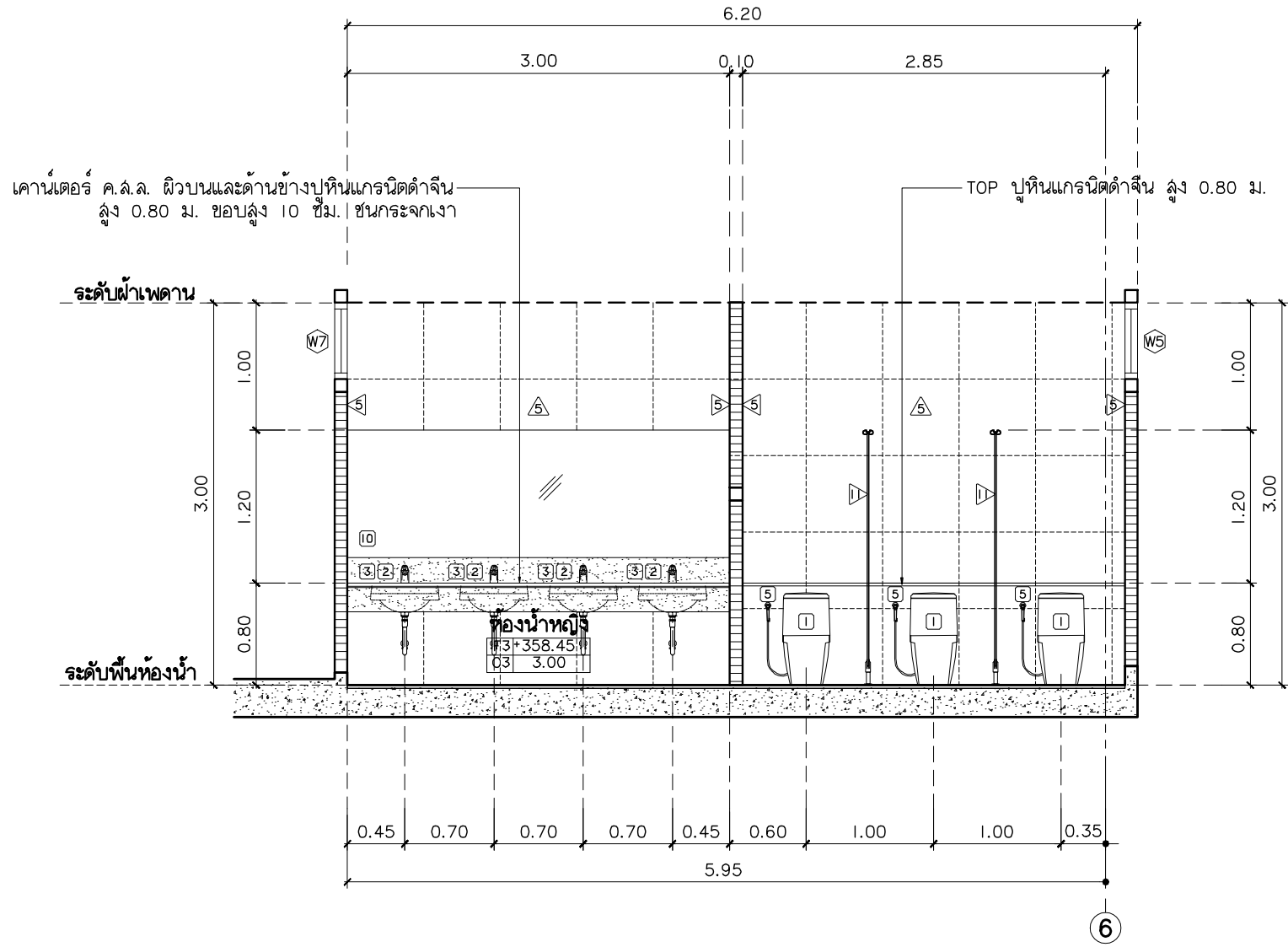
รูปตัด I-B มาตราส่วน 1:50
