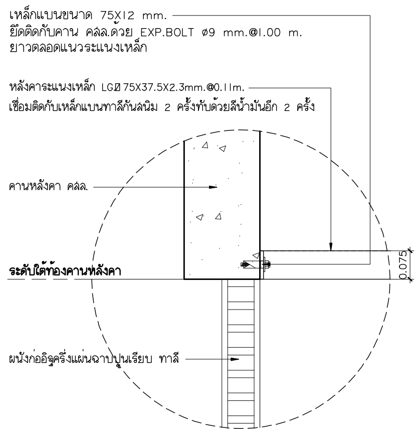
แบบขยาย SSI-3 มาตราส่วน 1:10
