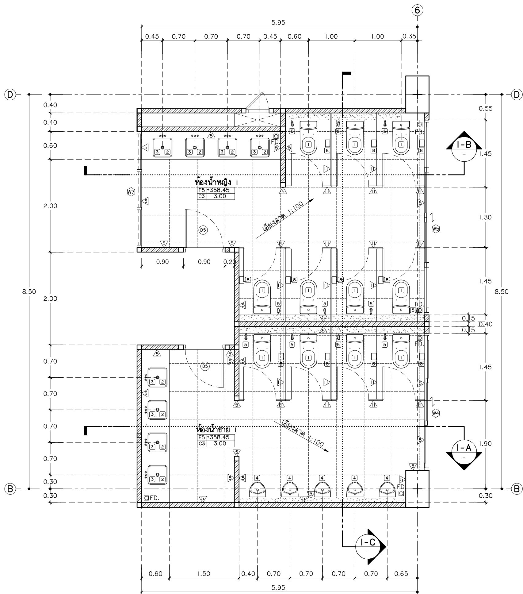
แบบขยายห้องน้ำ แปลน มาตราส่วน 1:50
