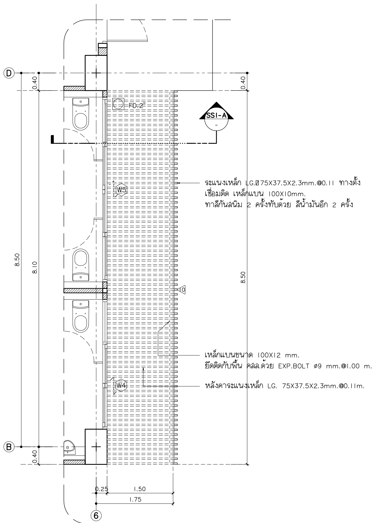
แบบขยาย SSI มาตราส่วน 1:50
