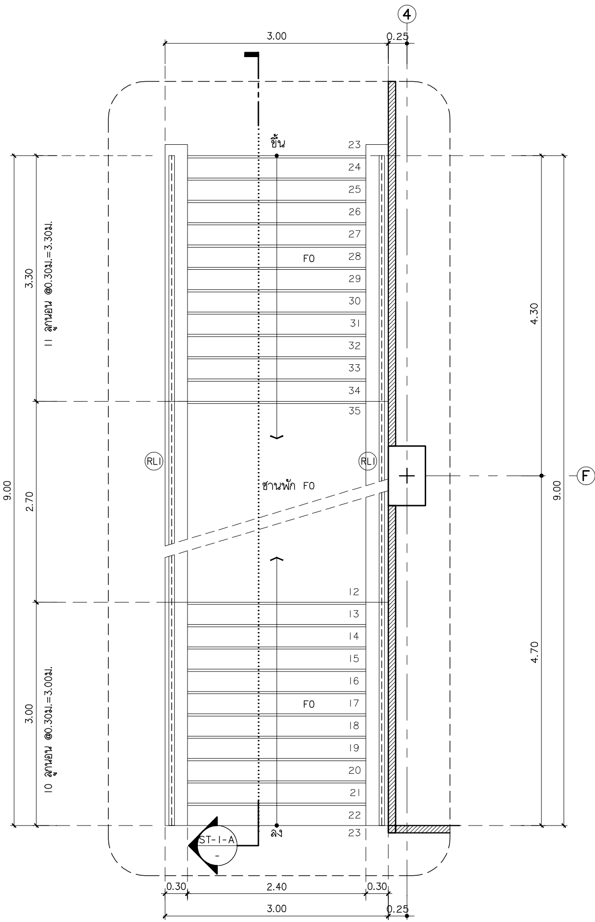
แบบขยายบันได ST-I ชั้นที่ 1 มาตราส่วน 1:50
