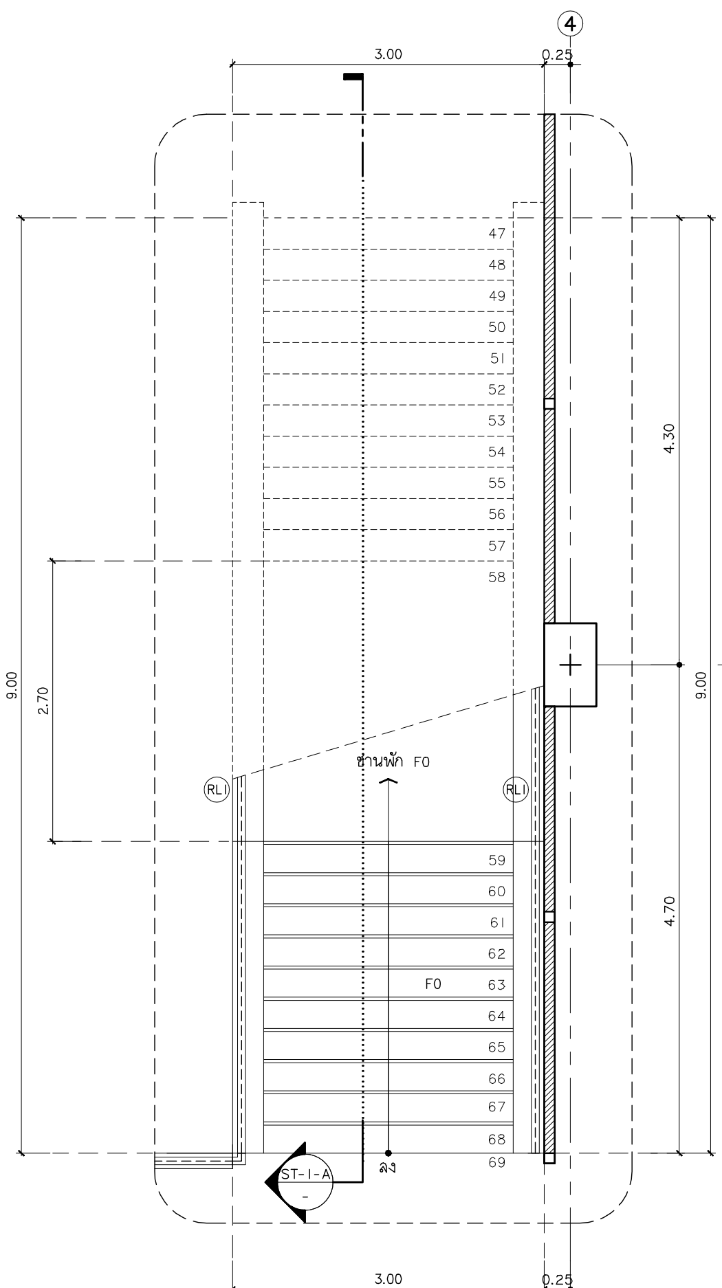
แบบขยายบันได ST-I ชั้นที่ 3 มาตราส่วน 1:50
