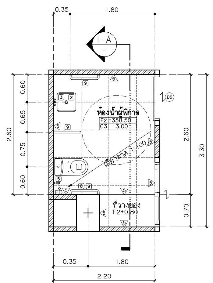
แบบขยายห้องน้ำคานพักการ มาตราส่วน 1:50
