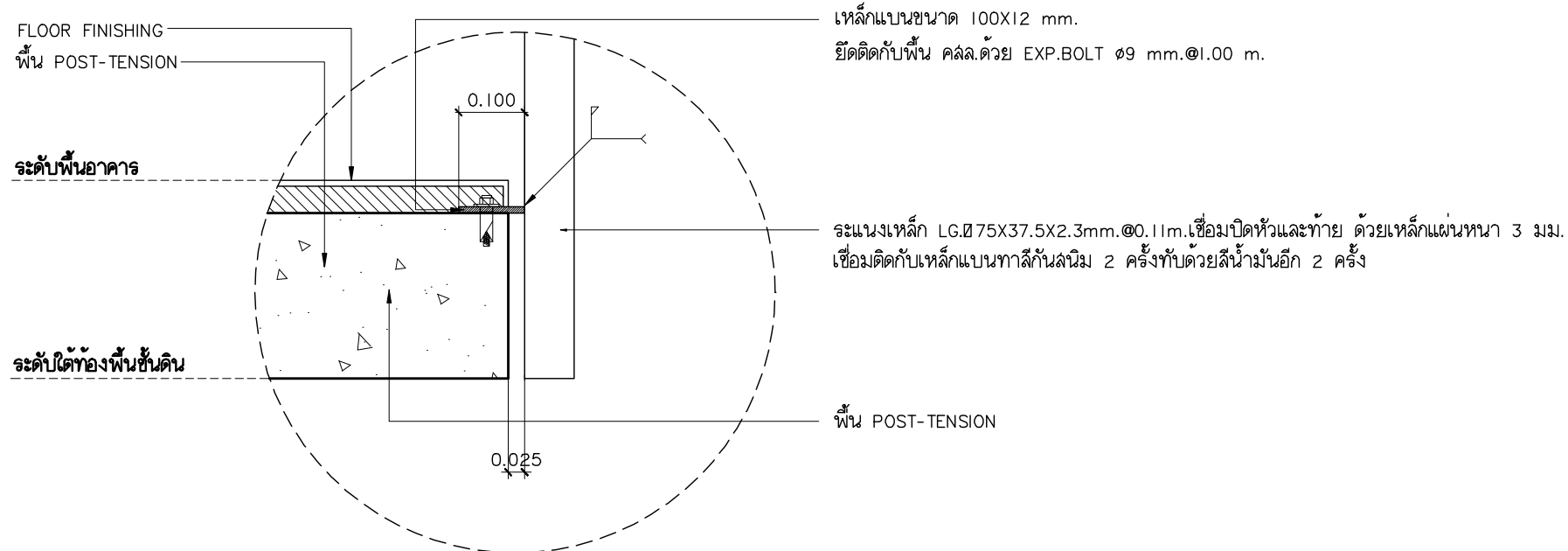
แบบขยาย SSI-1 มาตราส่วน 1:10
