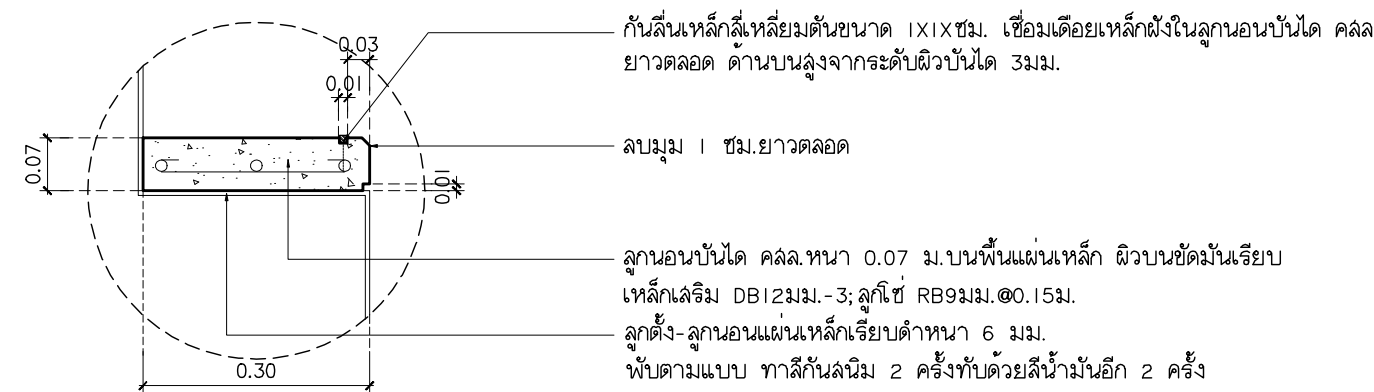
แบบขยาย ST-I-D มาตราส่วน 1:10
