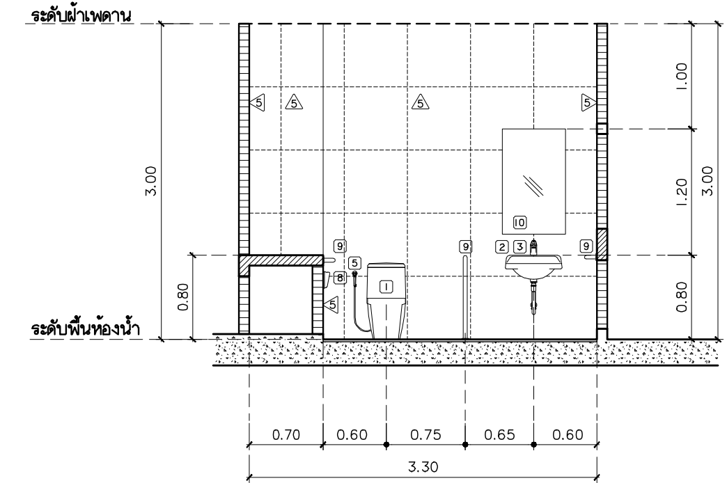
รูปตัด I-A มาตราส่วน 1:50
