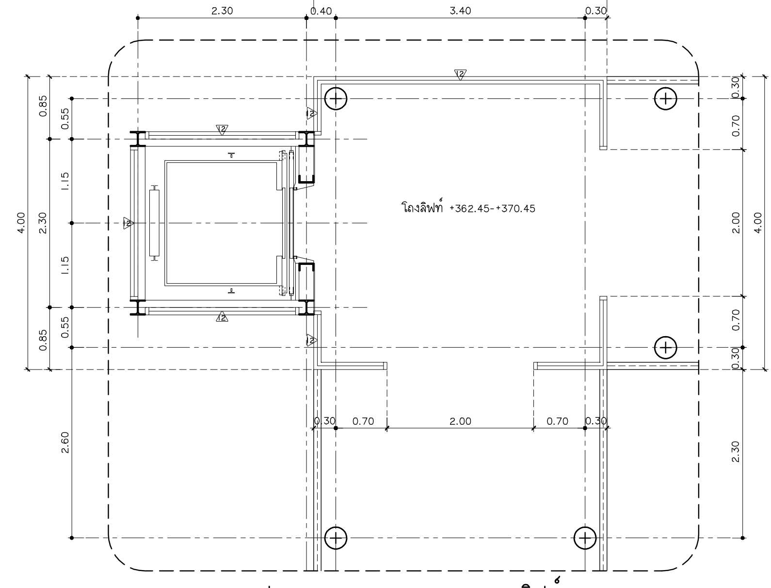
แผน +362.50-+370.50 ขยายลิฟท์ มาตราส่วน 1:50
