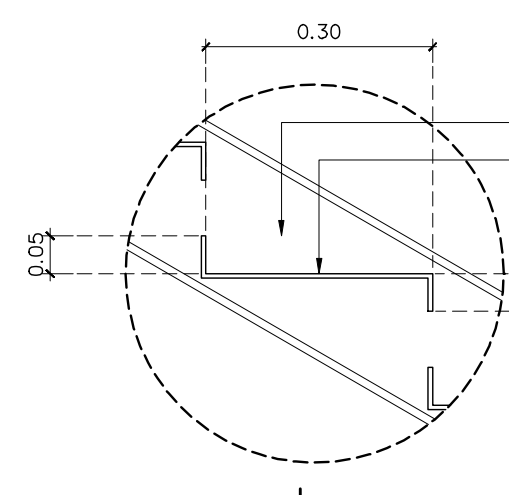
แบบขยายบันได ST-2-B มาตราส่วน 1:50
