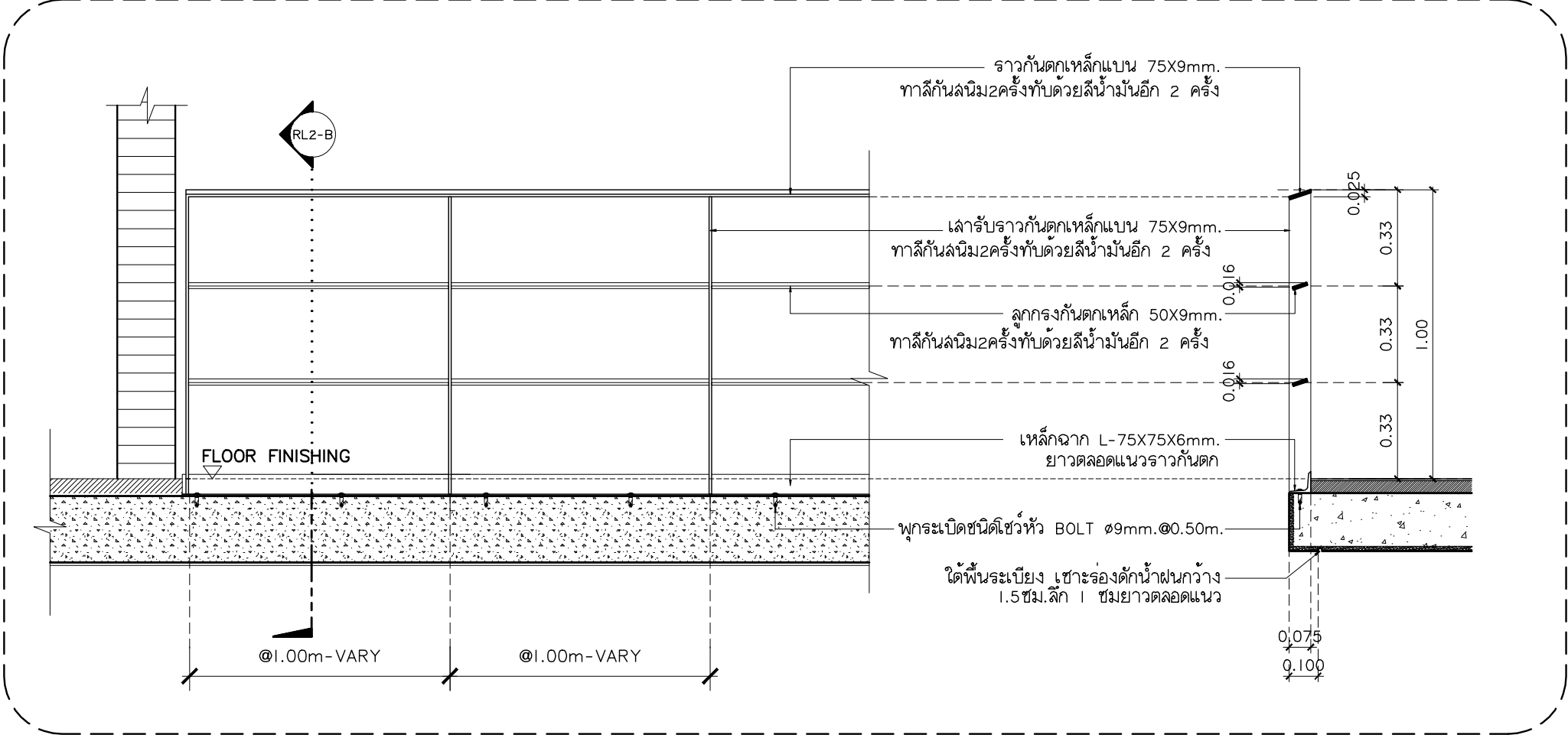
แบบขยายรากก้นตึก ภายนอกอาคาร มาตราส่วน 1:20
