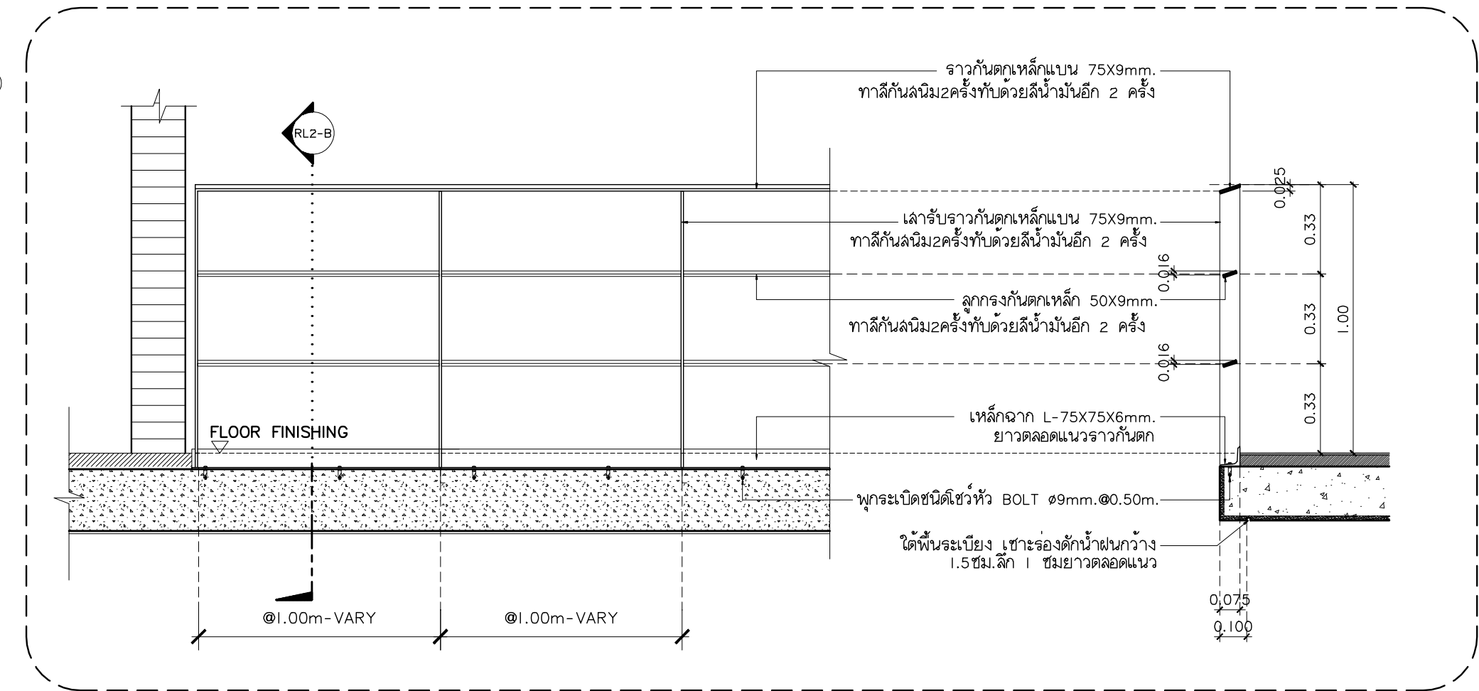
RL 1 แบบขยายจากรากันคก ภายนอกอาคาร มาตราส่วน 1:20
