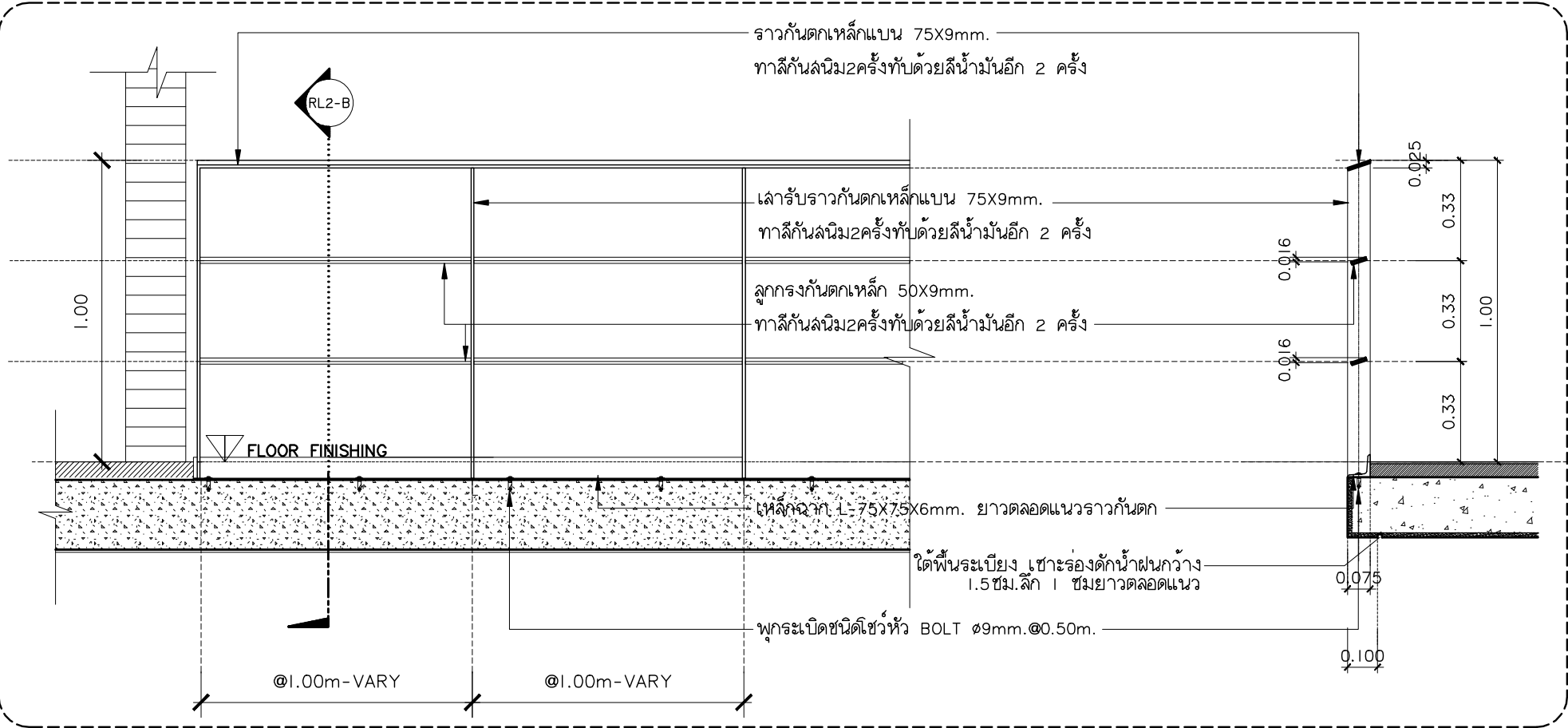
แบบขยายจากรั้วกันตก ภายนอกอาคาร มาตราส่วน 1:20
