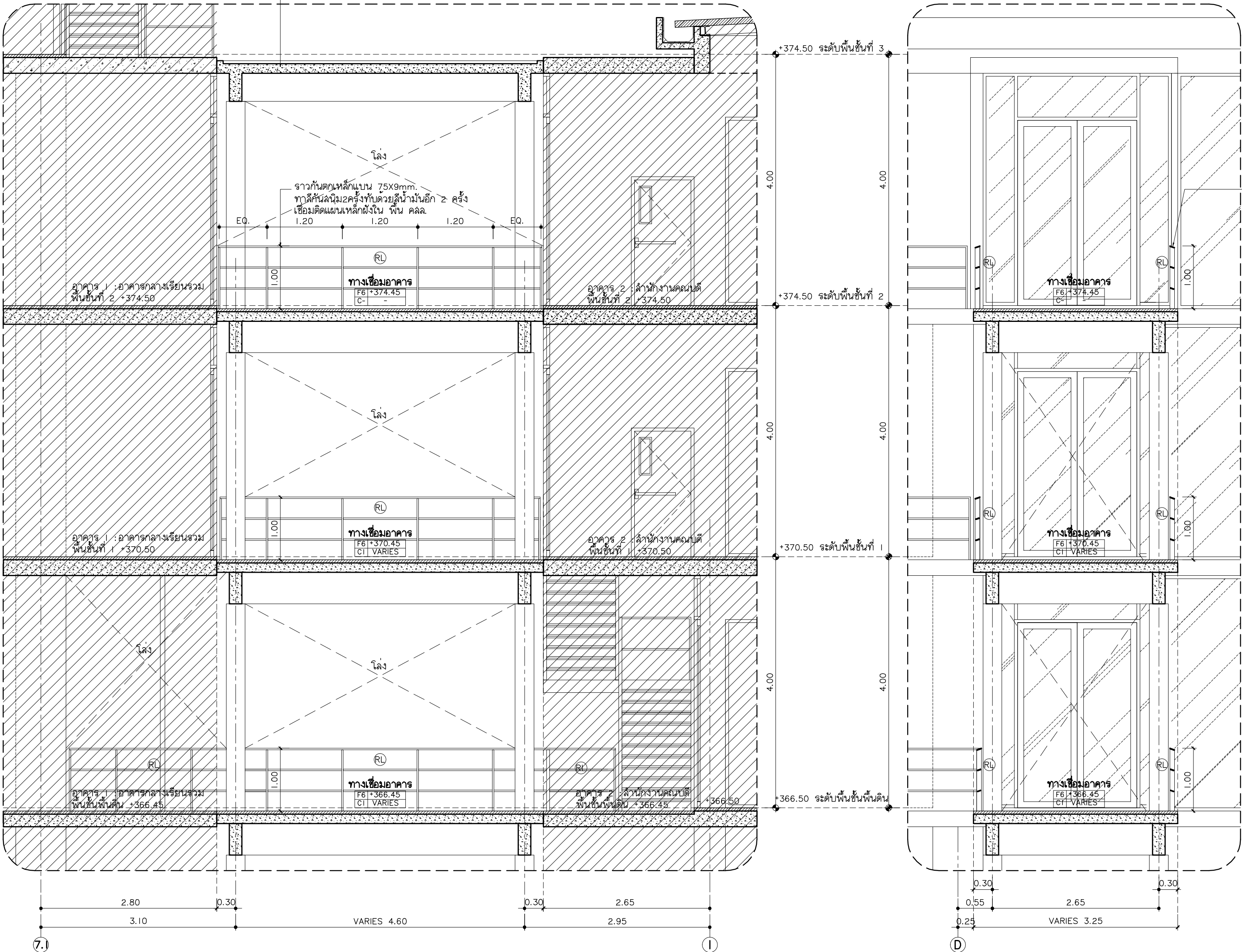
รูปตัด A ขยายทางเชื่อม 4 มาตราส่วน 1:50
