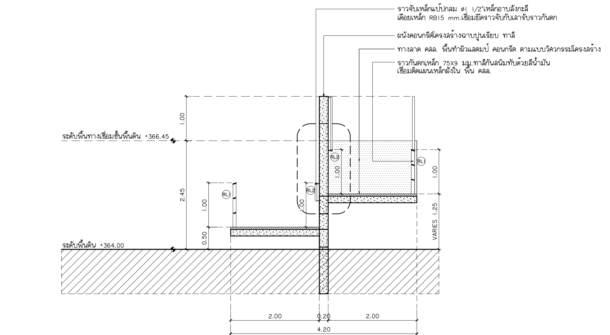
รูปตัด C ขยายทางเชื่อม 7 มาตราส่วน 1:50
