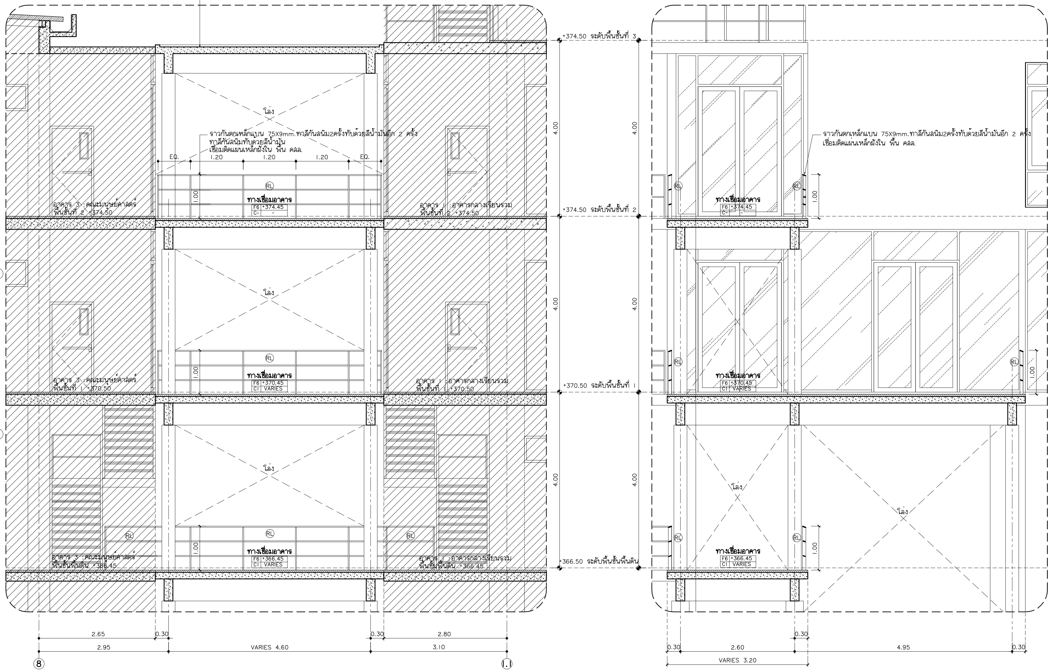
รูปตัด A ขยายทางเชื่อม 3 มาตราส่วน 1:50
