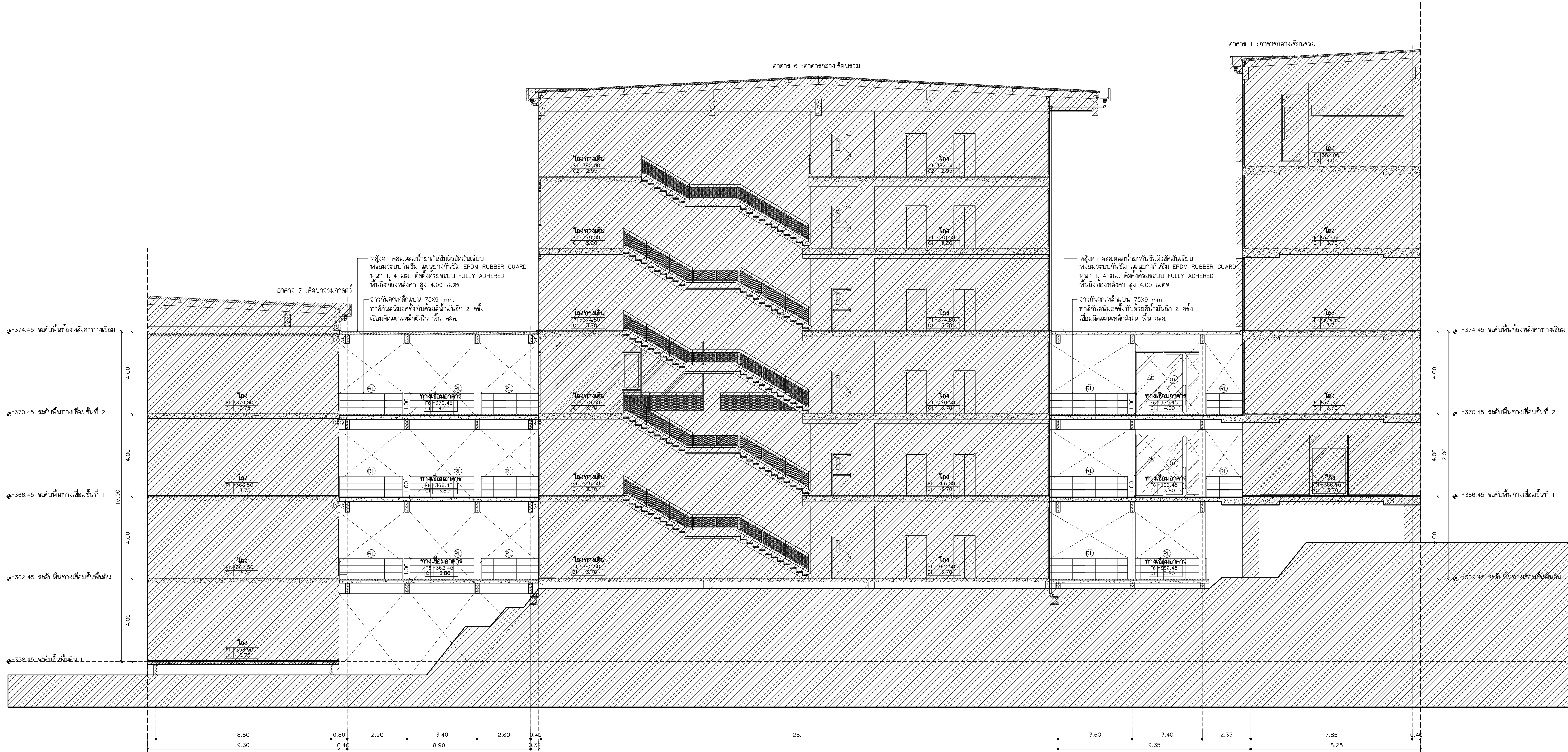
รูปตัด D ขยายทางเชื่อม 5 มาตราส่วน 1:100
