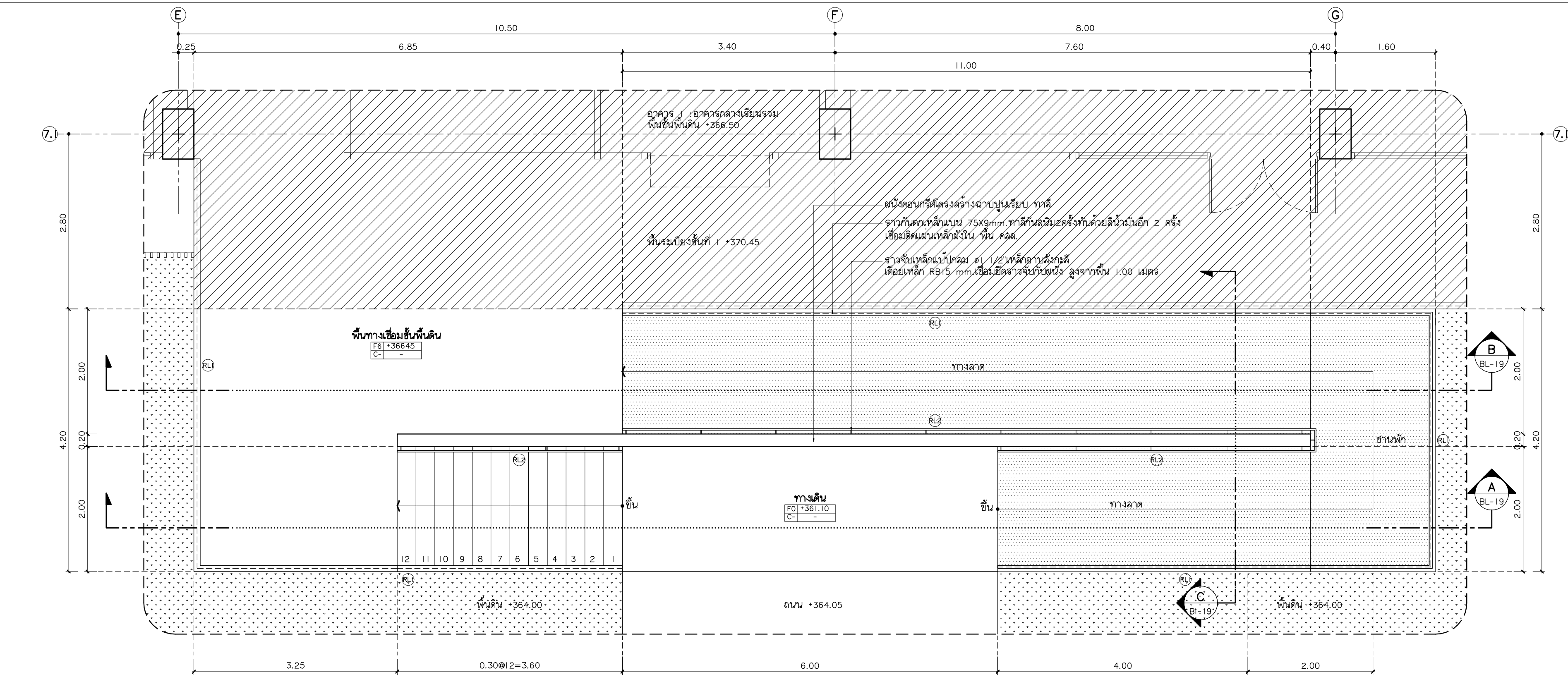
แปลน ขยายทางเชื่อม 7 มาตราส่วน 1:50
