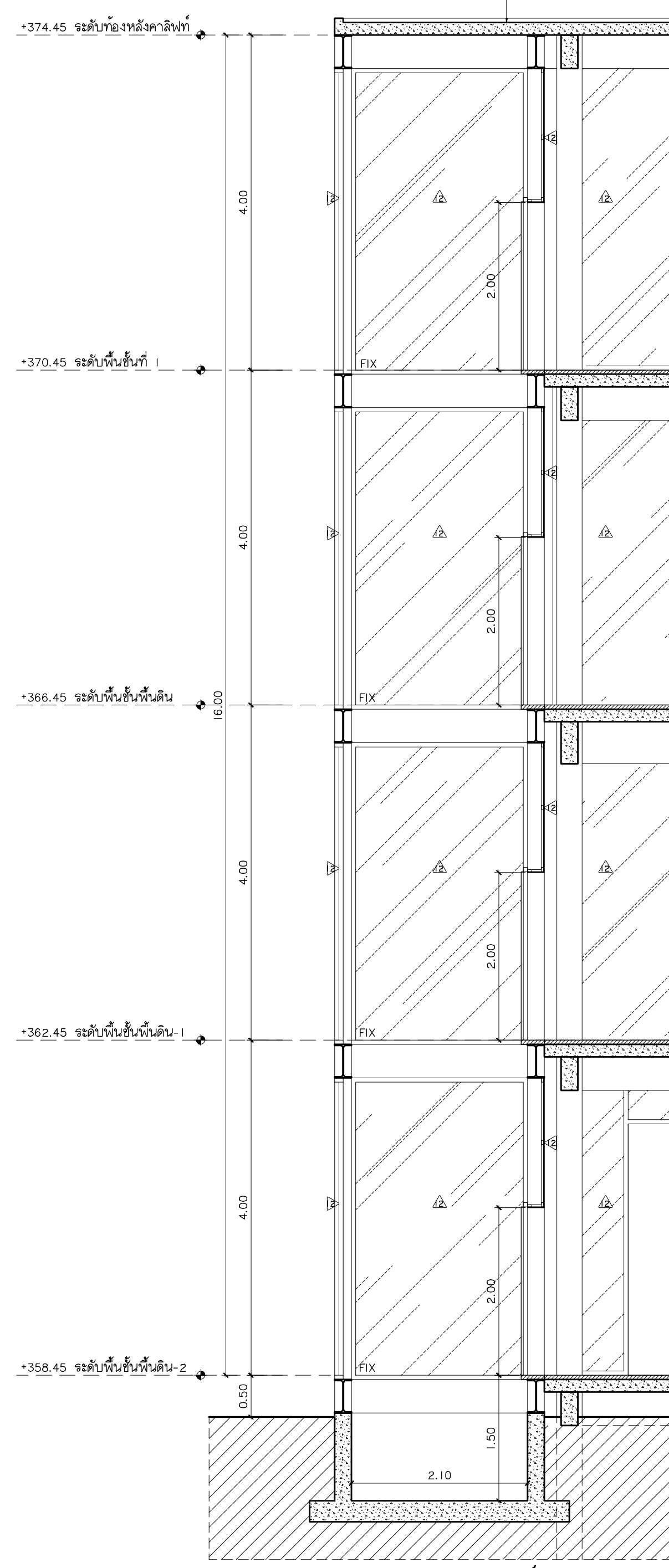
รูปตัด A ขยายลิฟท์ มาตราส่วน 1:50
