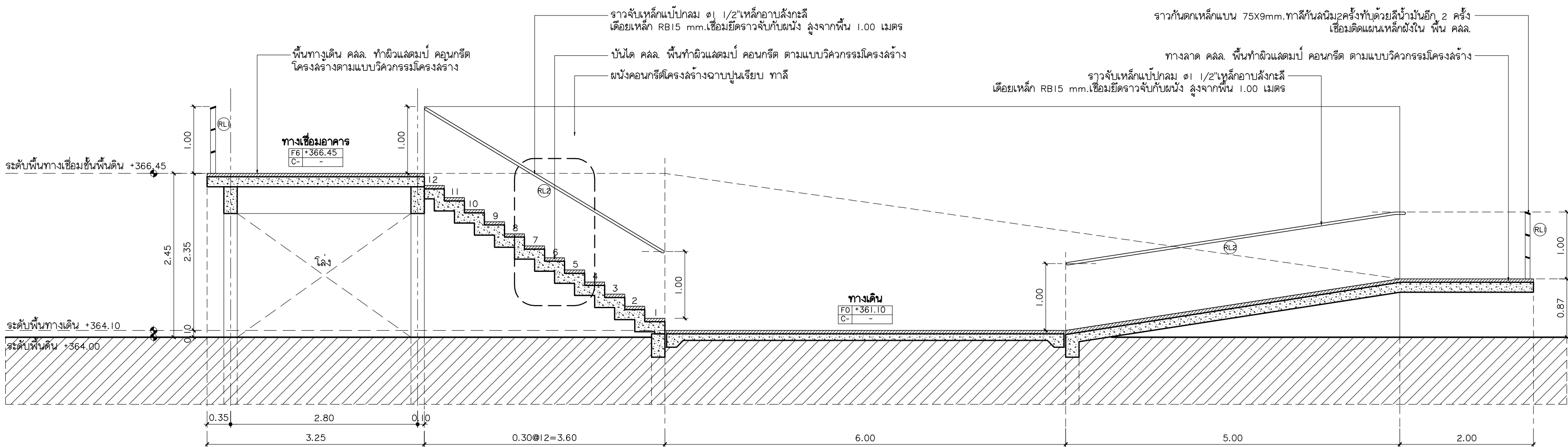
รูปตัด A ขยายทางเชื่อม 7 มาตราส่วน 1:50
