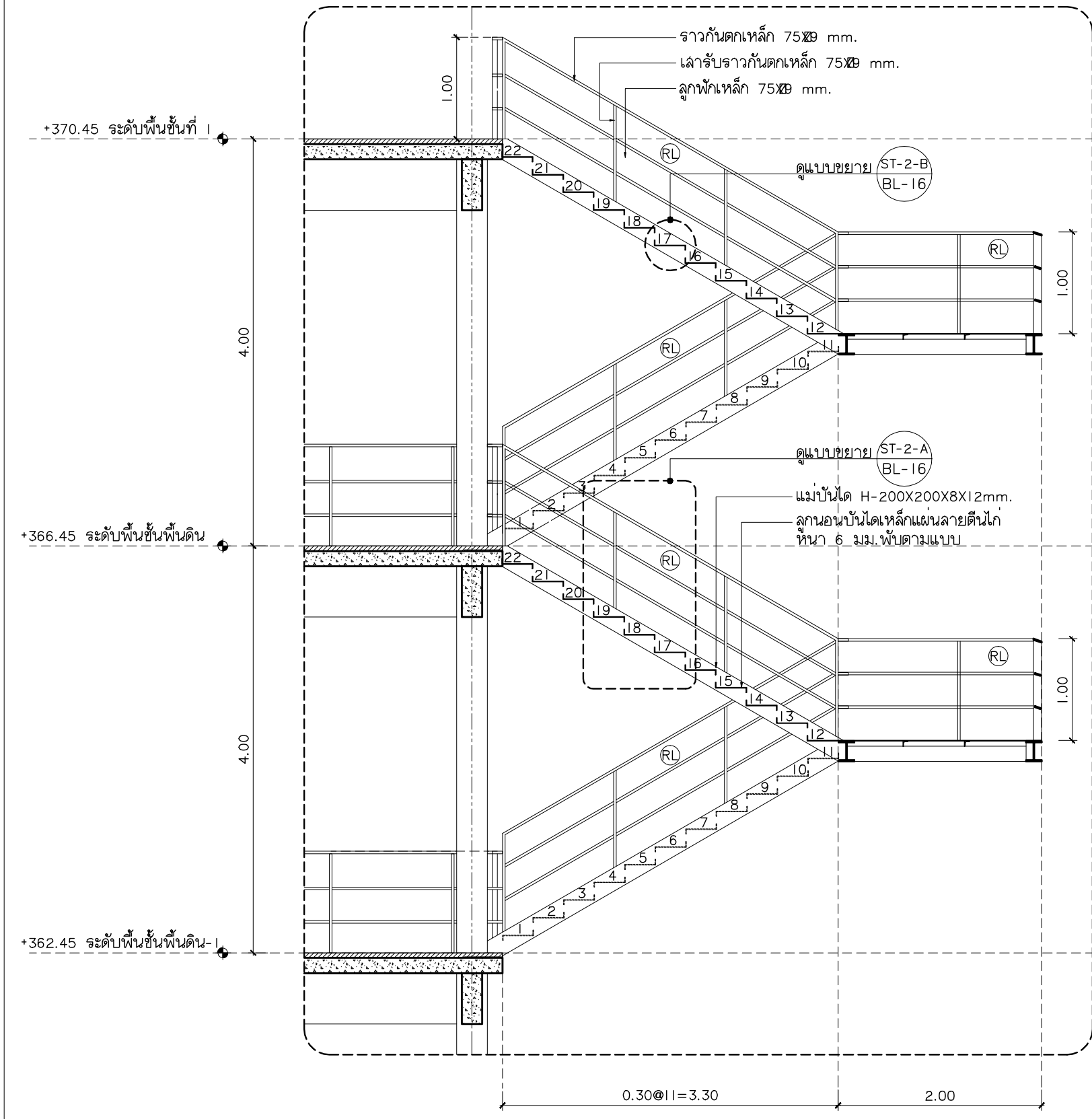
รูปตัด A ขยายบันไดทางเชื่อม มาตราส่วน 1:50
