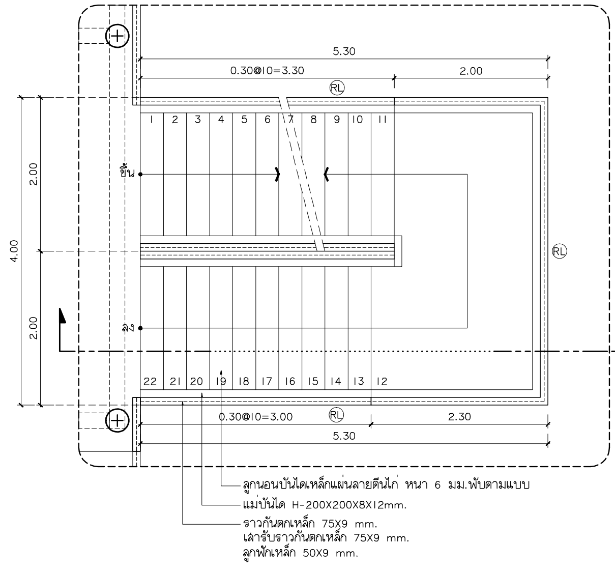
แบบขยายบันไดทางเชื่อม มาตราส่วน 1:50
