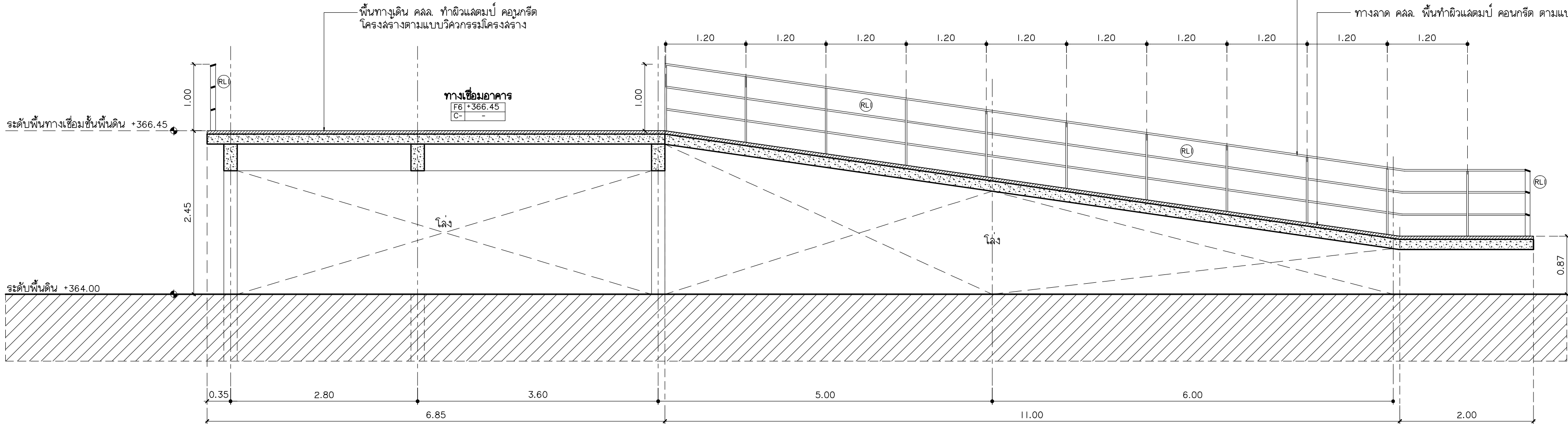
รูปตัด B ขยายทางเชื่อม 7 มาตราส่วน 1:50
