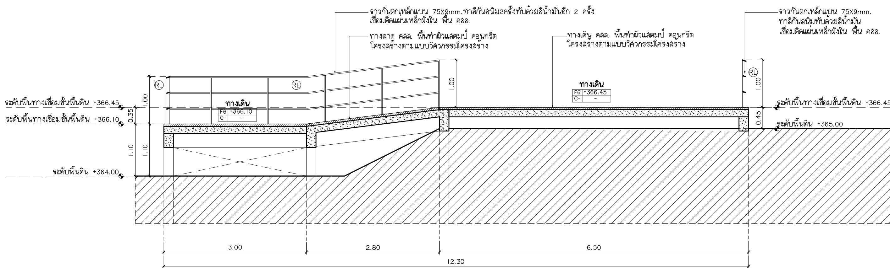
รูปตัด A ขยายทางเชื่อม 9 มาตราส่วน 1:50
