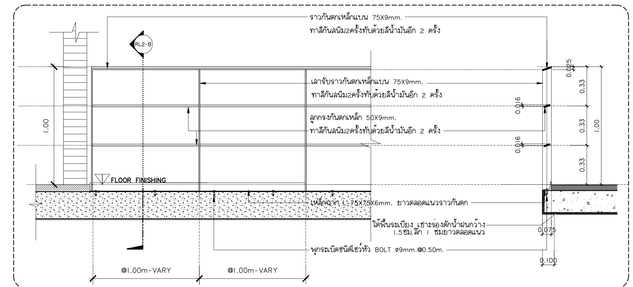
แบบขยายรากันตค ภายนอกอาคาร มาตราล้นน 1: 20
