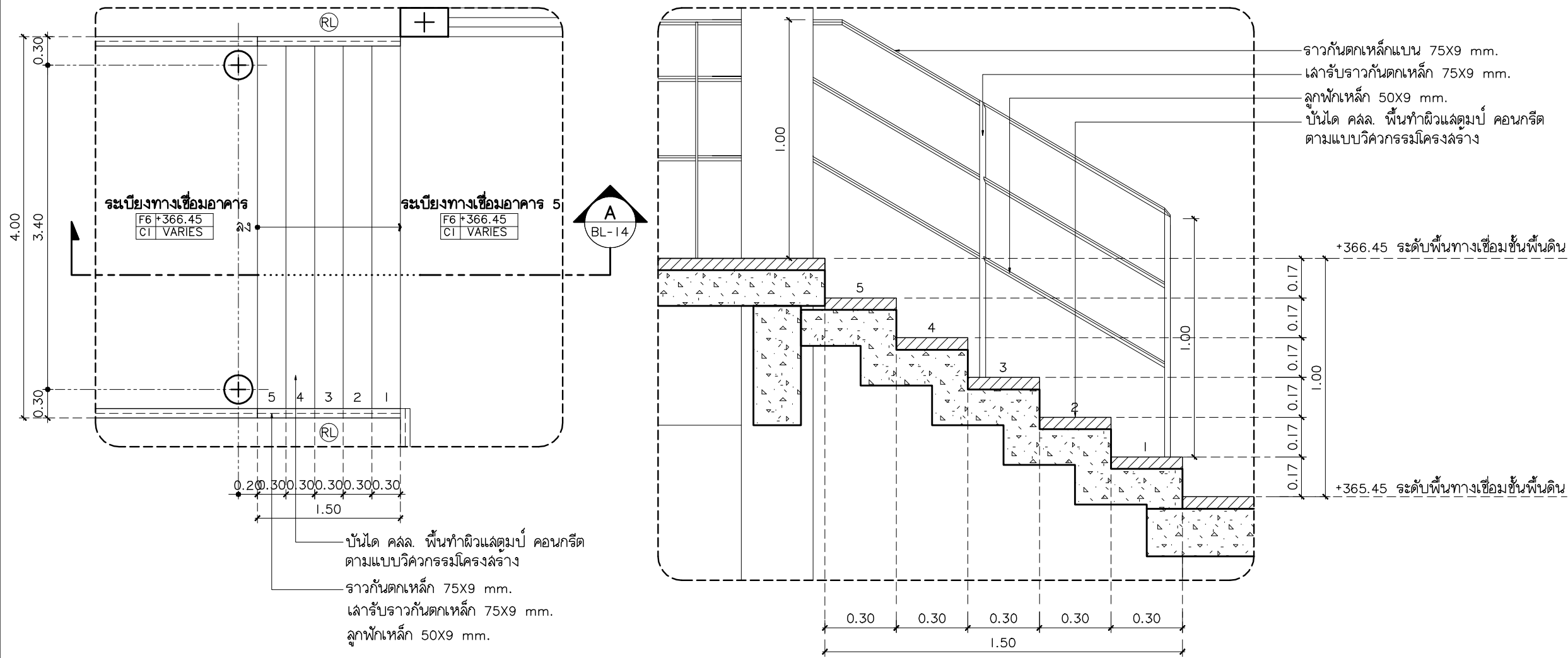
แปลน ST-1 บันไดทางเชื่อม มาตราส่วน 1:50
