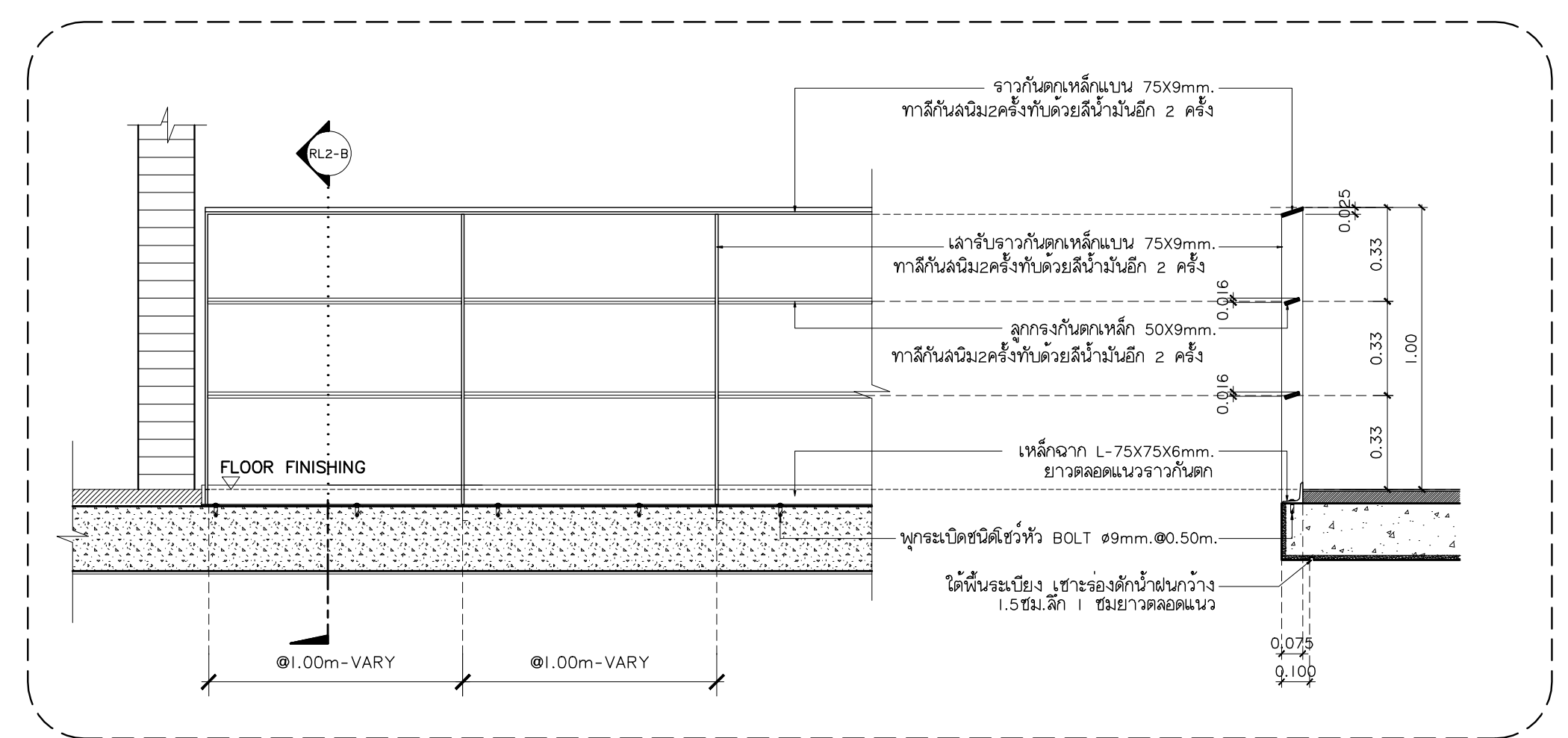
แบบขยายราวกันตก ภายนอกอาคาร มาตราส่วน 1:20
