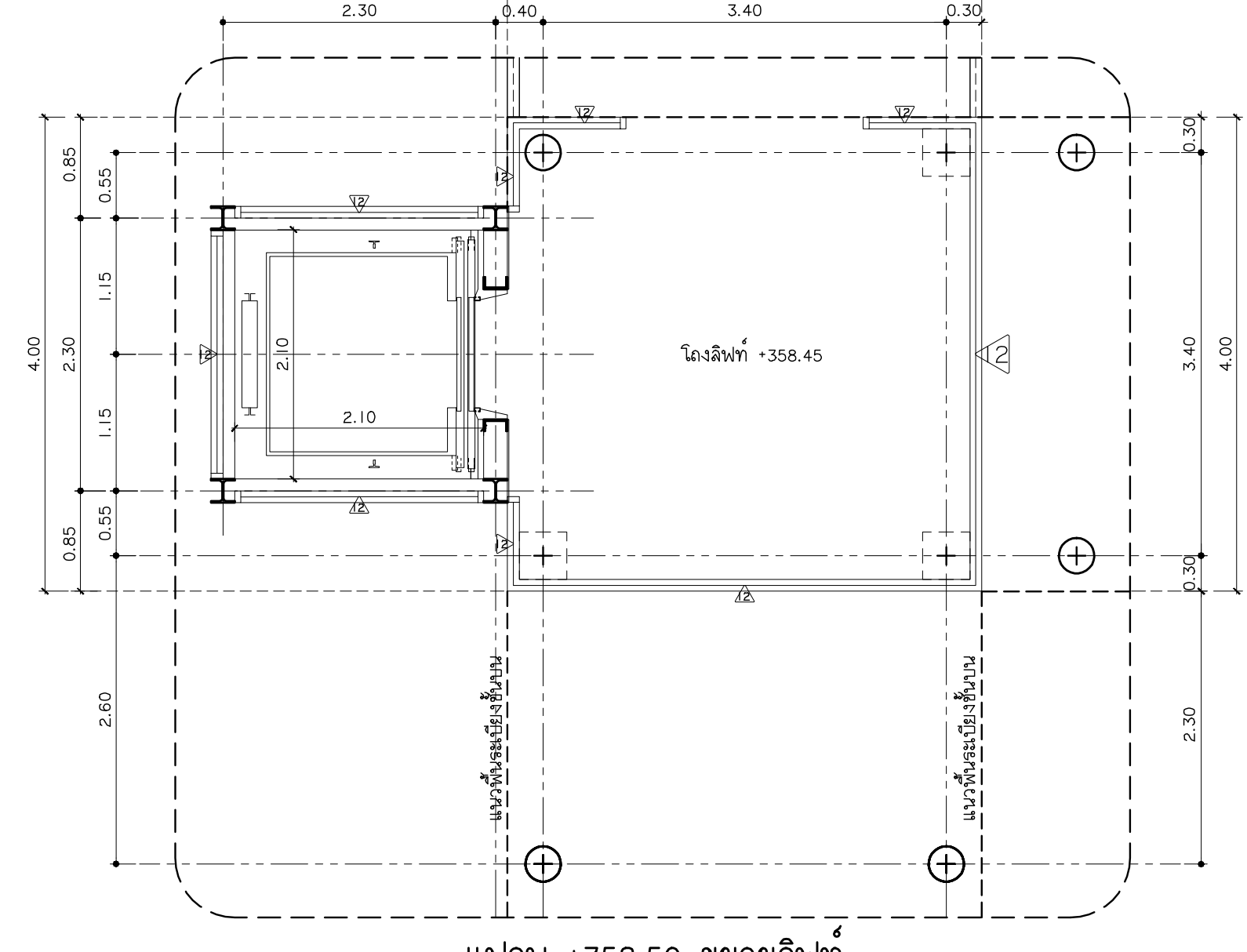
แผน +358.50 ขยายลิฟท์ มาตราส่วน 1:50
