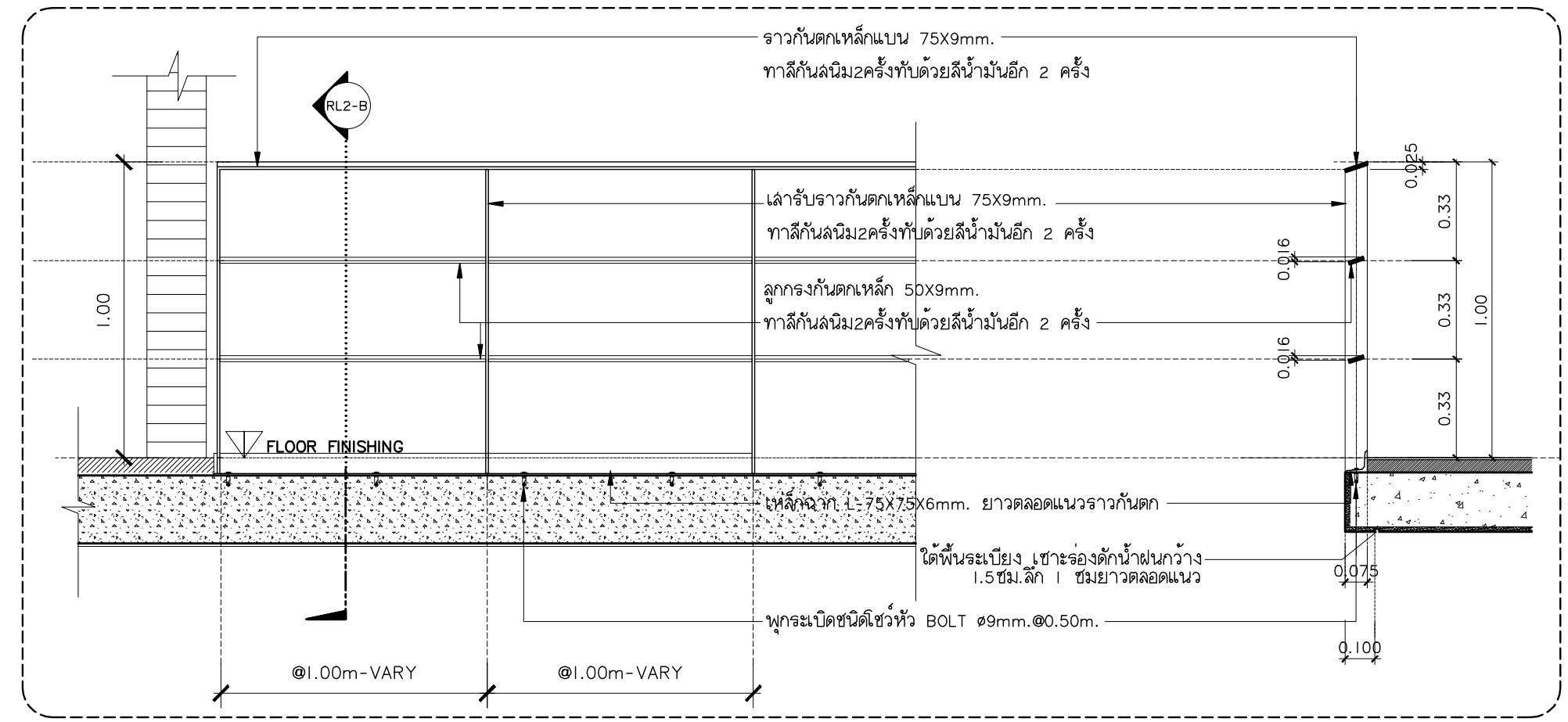
แบบขยายราวกันตก ภายนอกอาคาร มาตราส่วน 1:20
