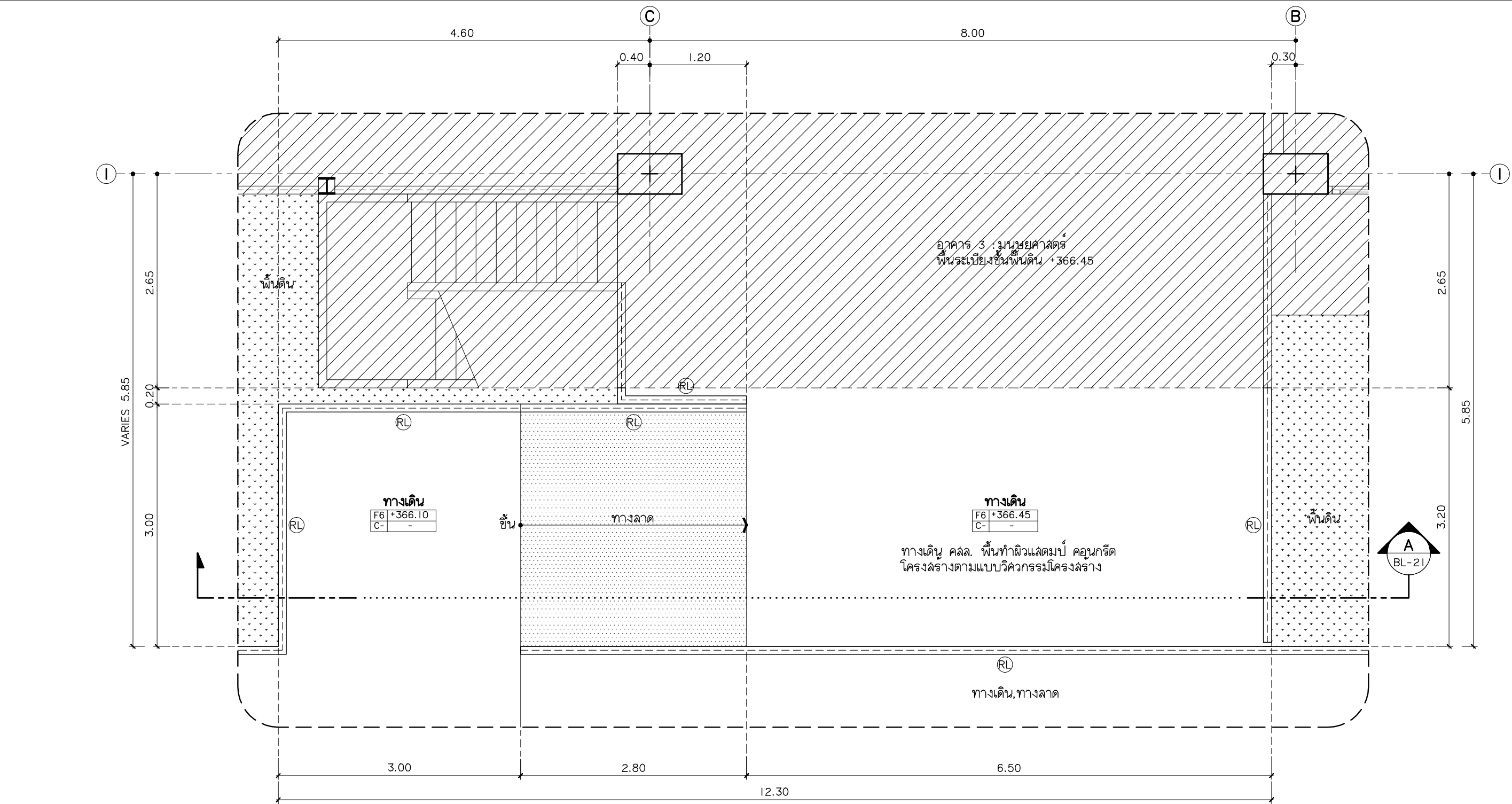
แผน ขยายทางเชื่อม 9 มาตราส่วน 1:50
