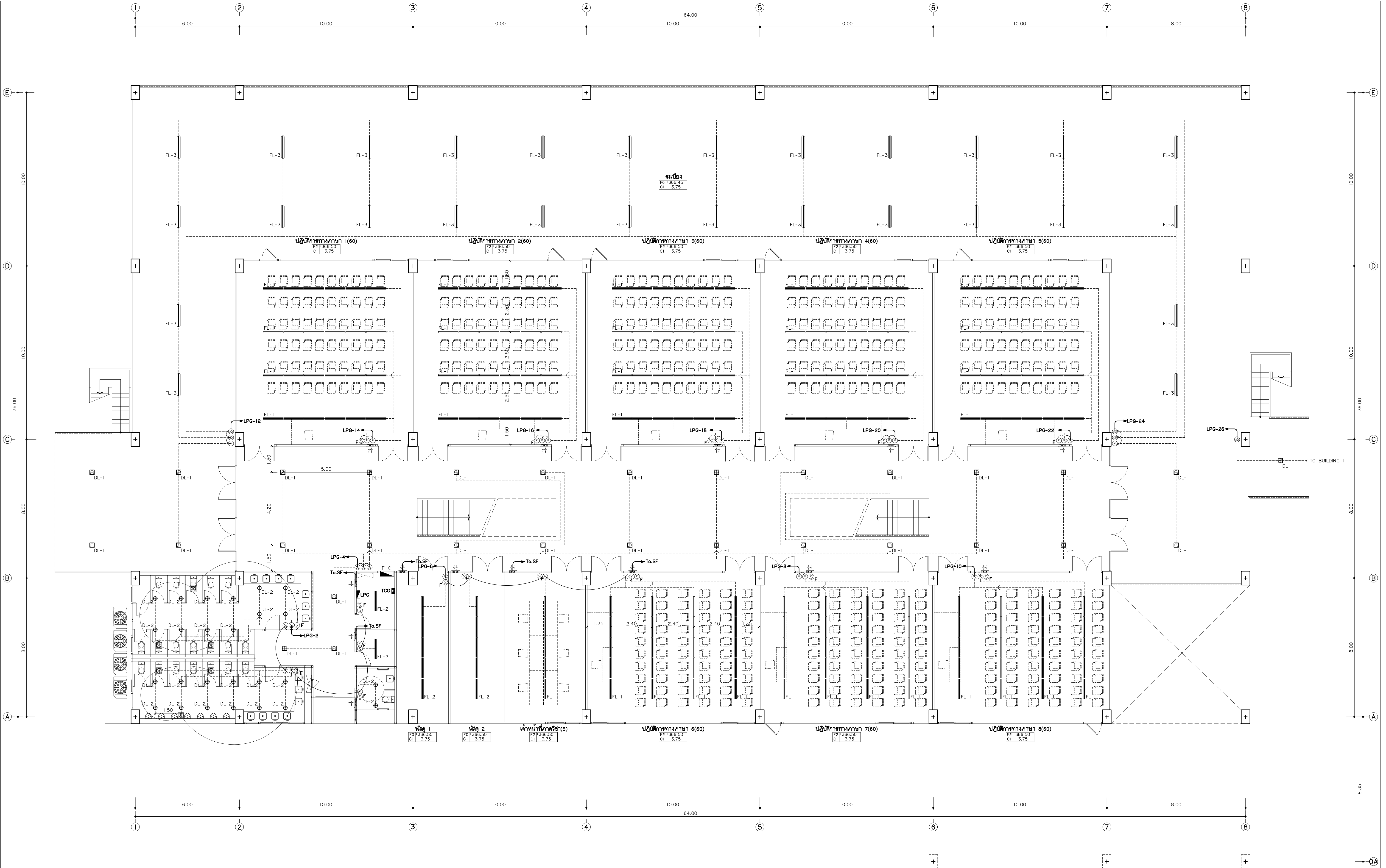
แปลนไฟฟ้าแสงสว่าง ชั้นพื้นดิน มาตราส่วน 1:100
