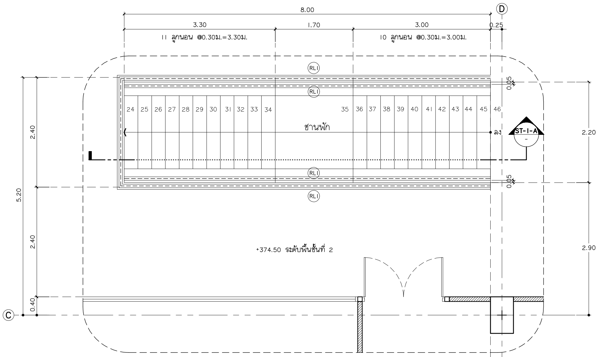
แบบขยายบันได ST-I ชั้นที่ 2 มาตราส่วน 1:50
