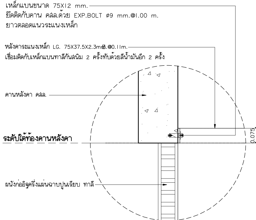
แบบขยาย SSI-3 มาตราส่วน 1:10
