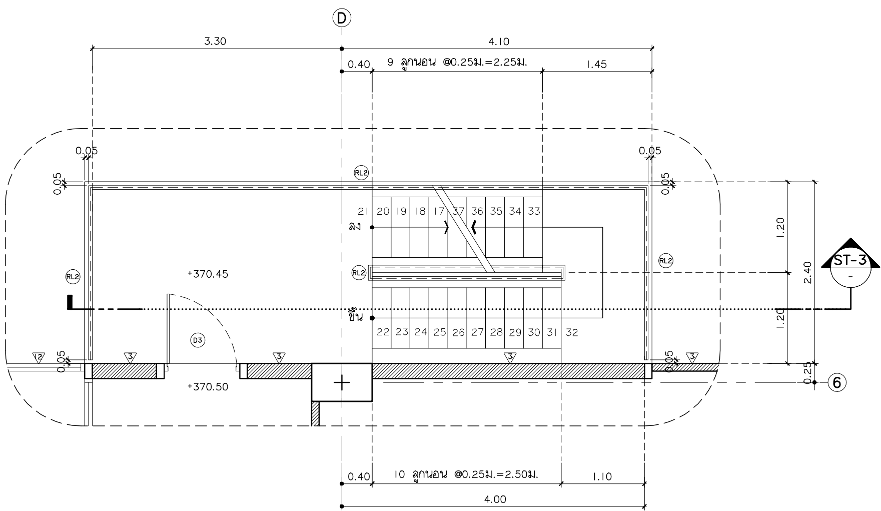
แบบขยายบันได ST-3,4 ชั้นที่ 1 มาตราส่วน 1:50
