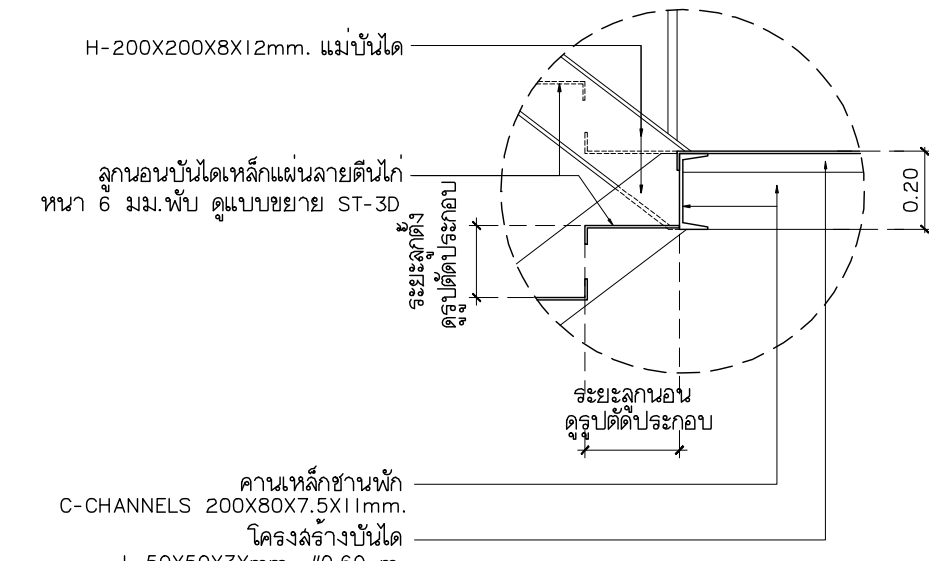
แบบขยาย ST-C มาตราส่วน 1:20
