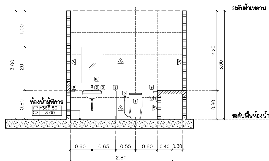
รูปตัด I-A มาตราส่วน 1:50
