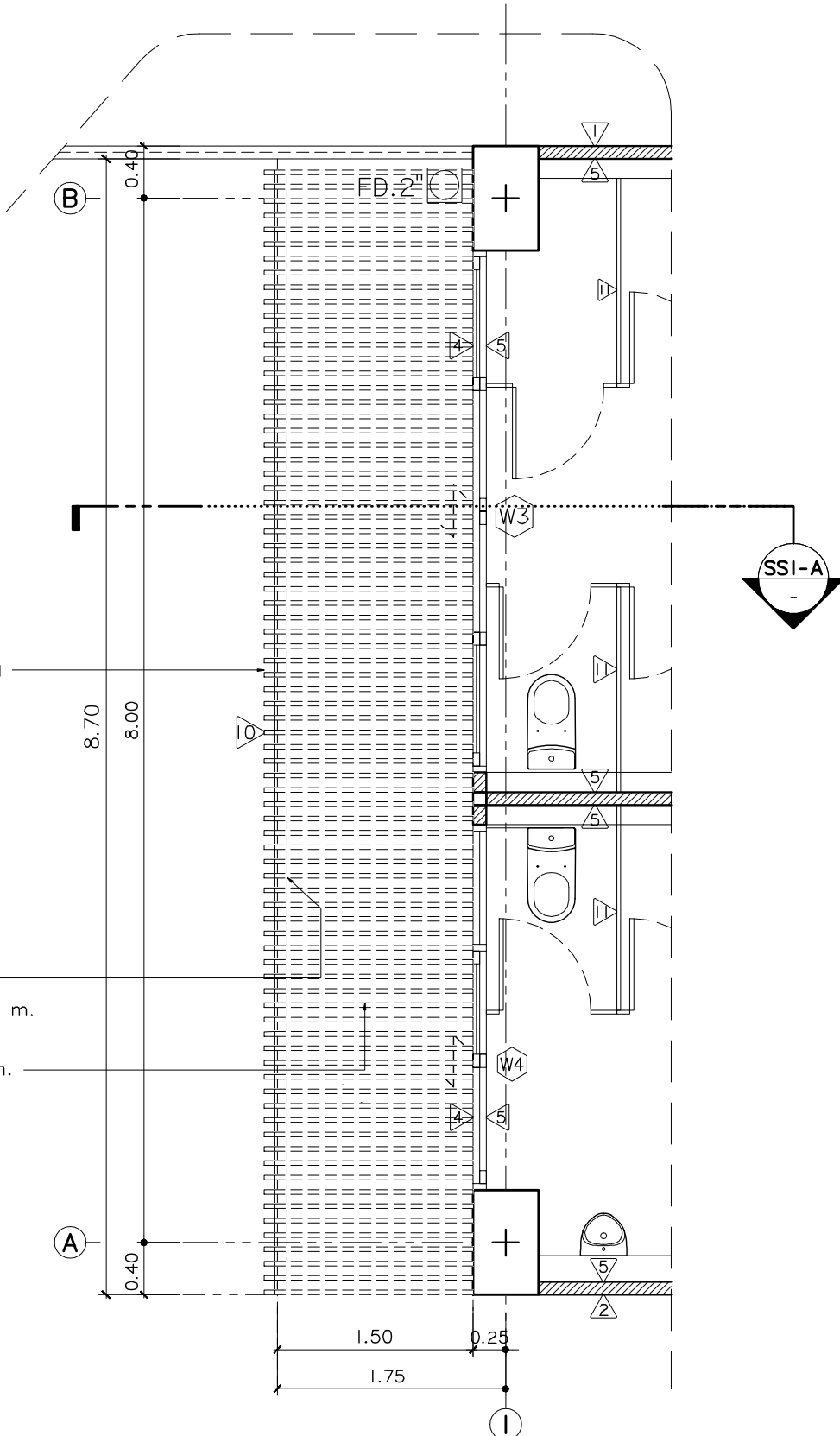
แบบขยายผนัง SSI แปลน มาตราส่วน 1:50
