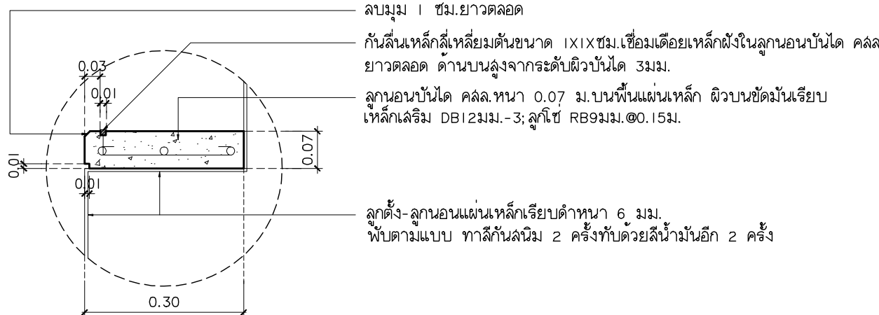
แบบขยาย ST-I-D มาตราส่วน 1:10
