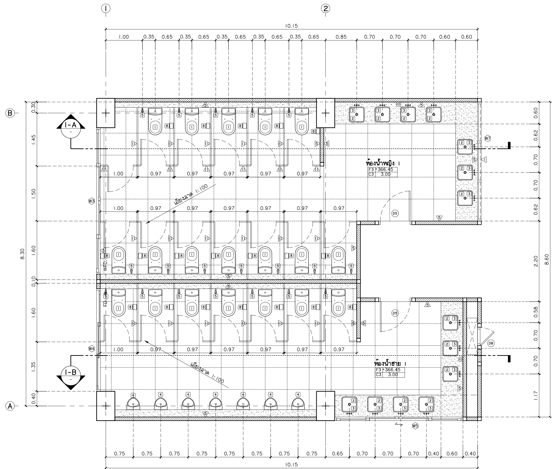
แบบขยายห้องน้ำ ชาย - หญิง มาตราส่วน 1:50
