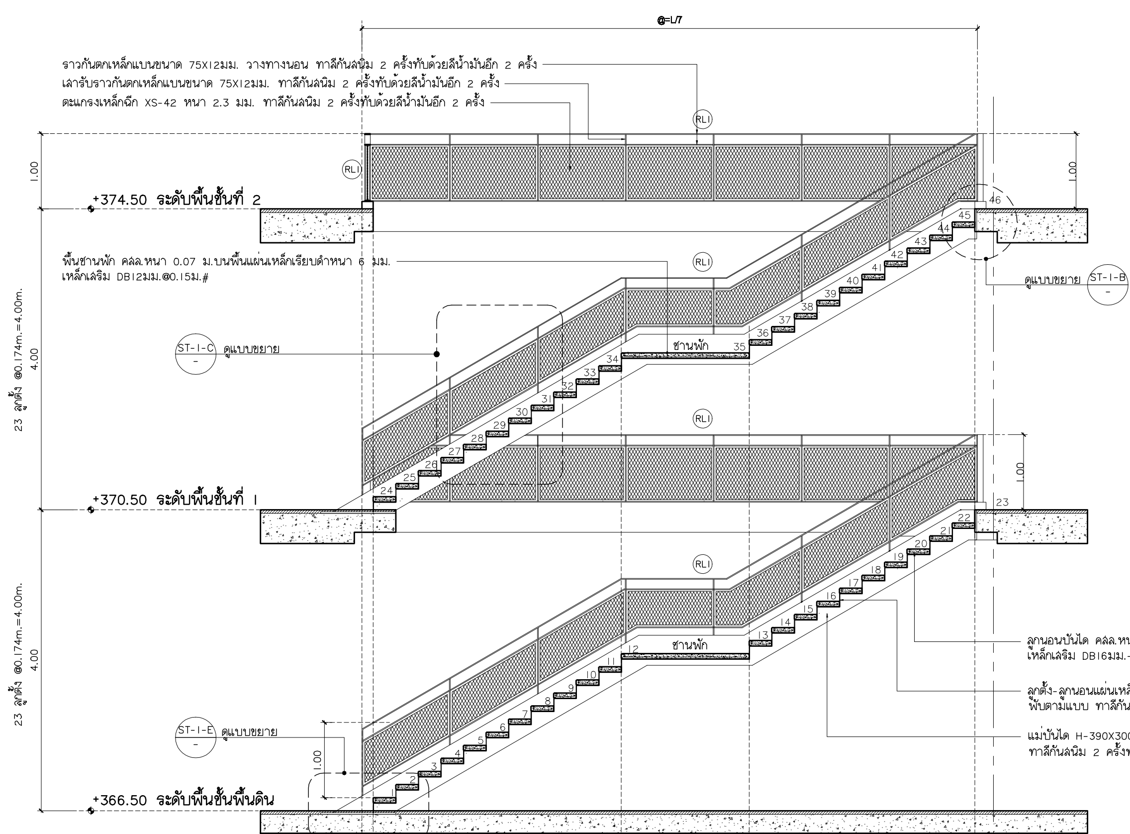
รูปตัด ST-I-A มาตราส่วน 1:50
