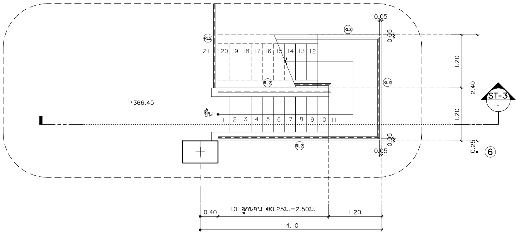
แบบขยายบันได ST-3,4 ชั้นพื้นดิน มาตราส่วน 1:50
