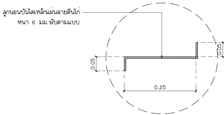
แบบขยาย ST-D มาตราส่วน 1:20
