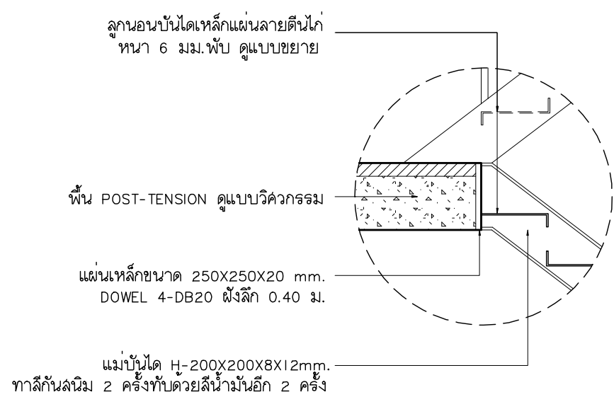
แบบขยาย ST-E มาตราส่วน 1:20
