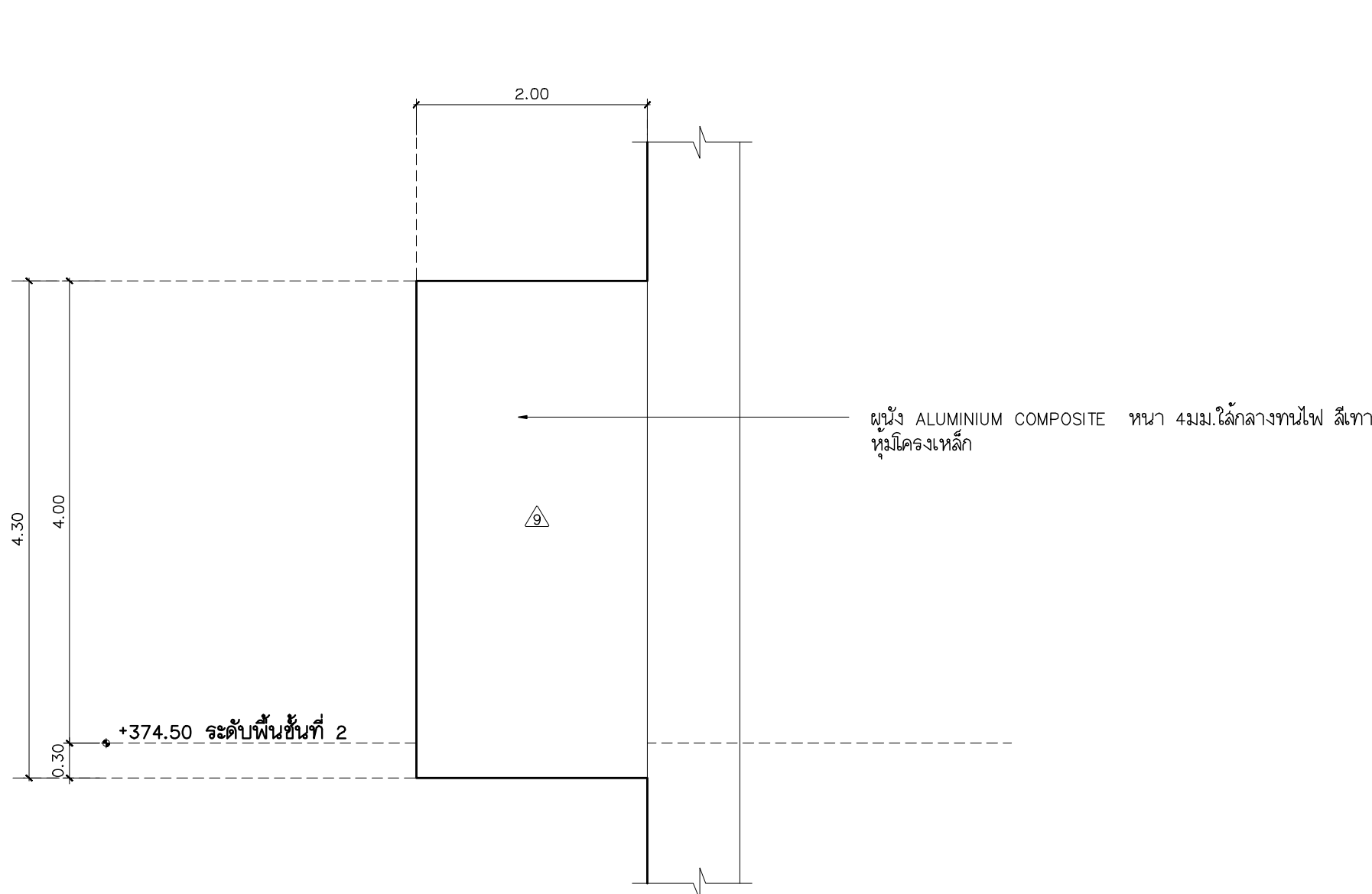
แบบขยาย FC-I รูปด้านหน้า มาตราส่วน 1:50
