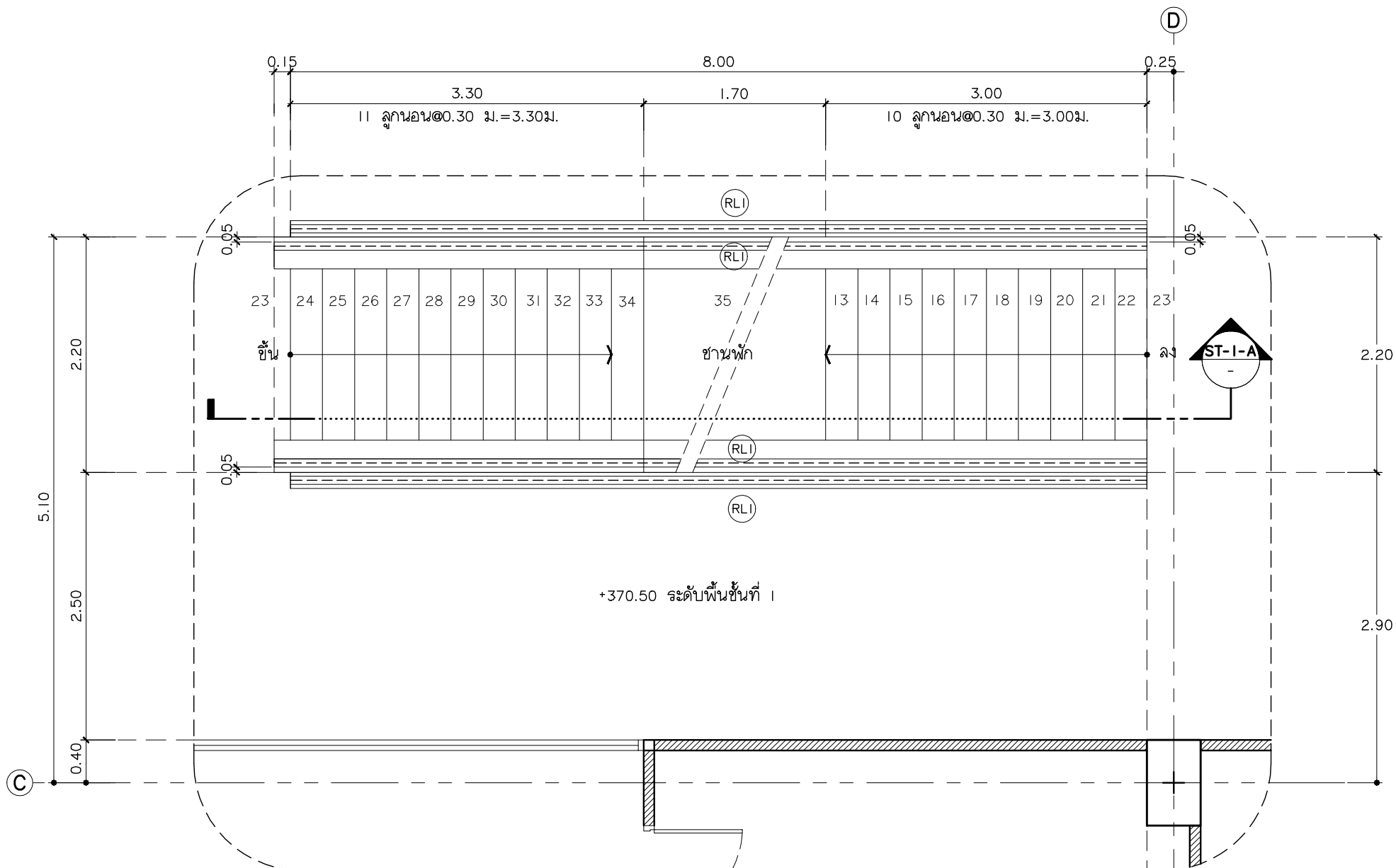
แบบขยายบันได ST-I ชั้นที่ 1 มาตราส่วน 1:50
