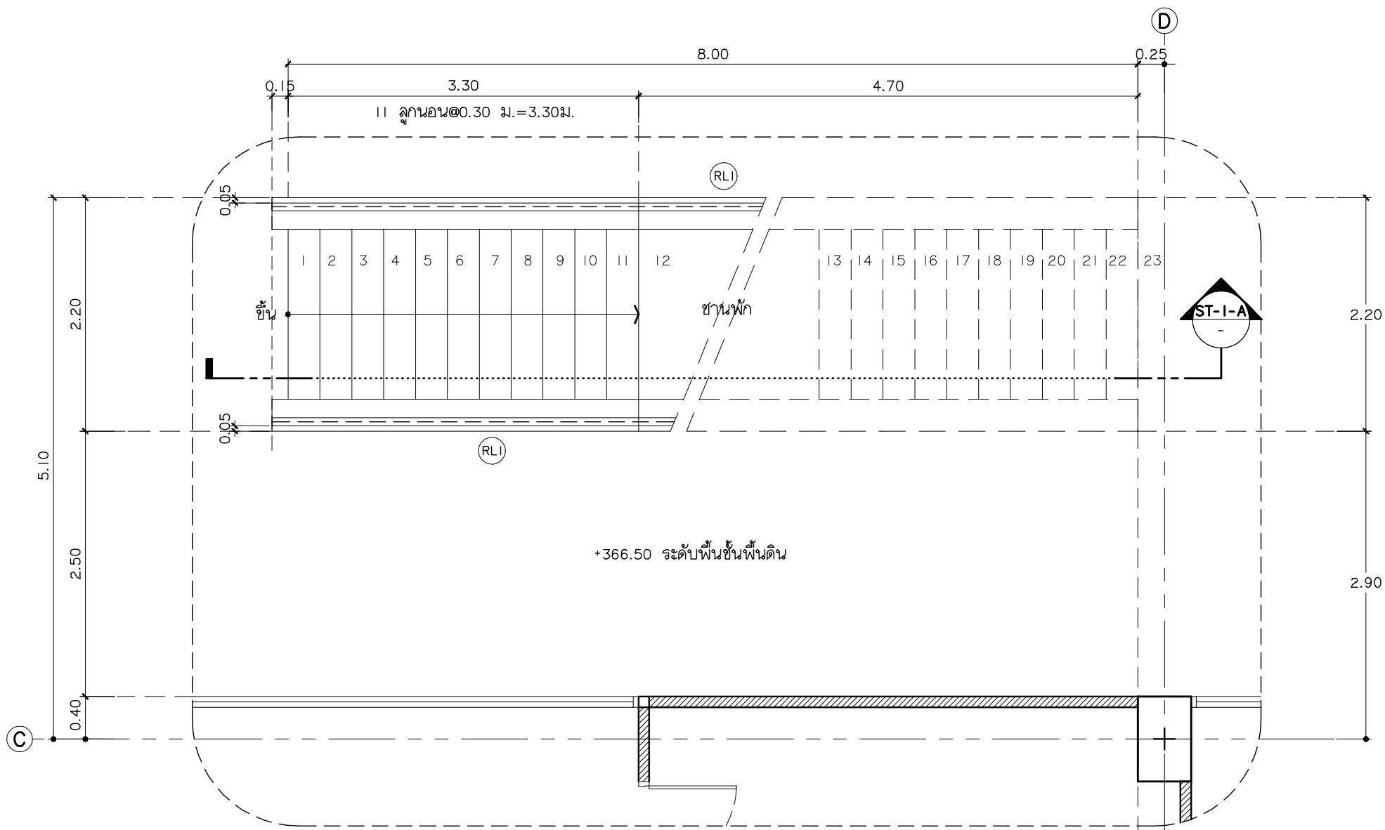
แบบขยายบันได ST-I ชั้นพื้นดิน มาตราส่วน 1:50
