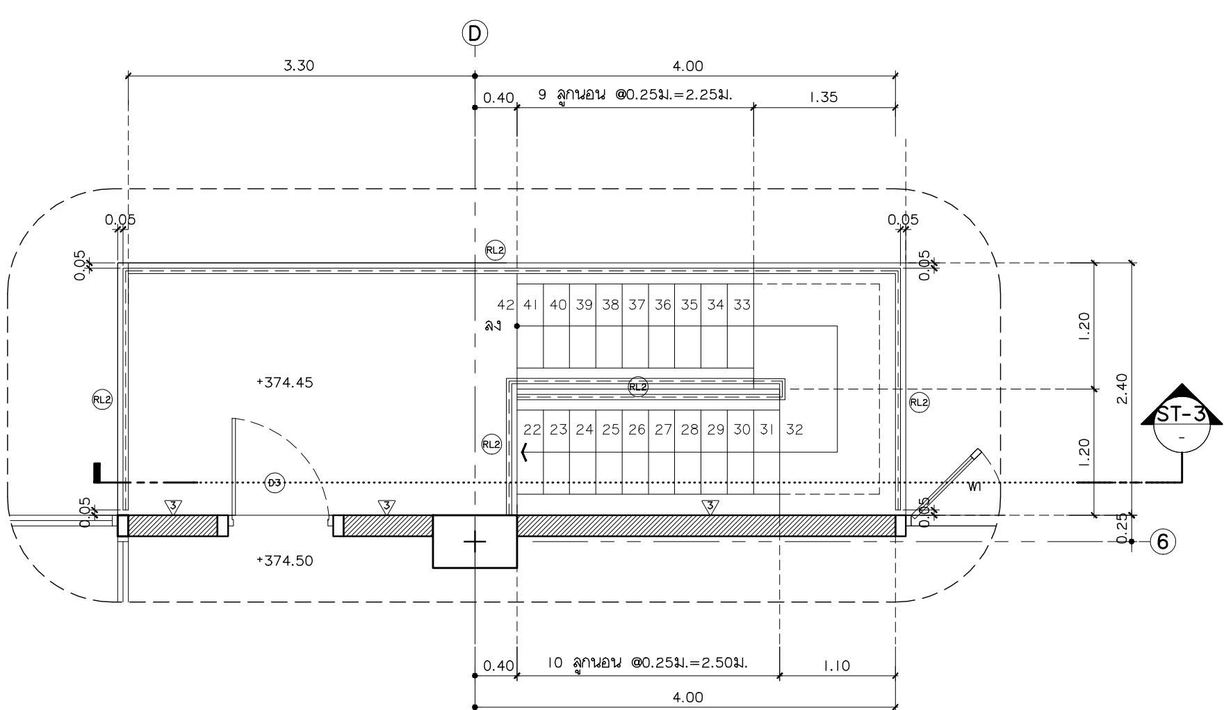
แบบขยายบันได ST-3,4 ชั้นที่ 2 มาตราส่วน 1:50
