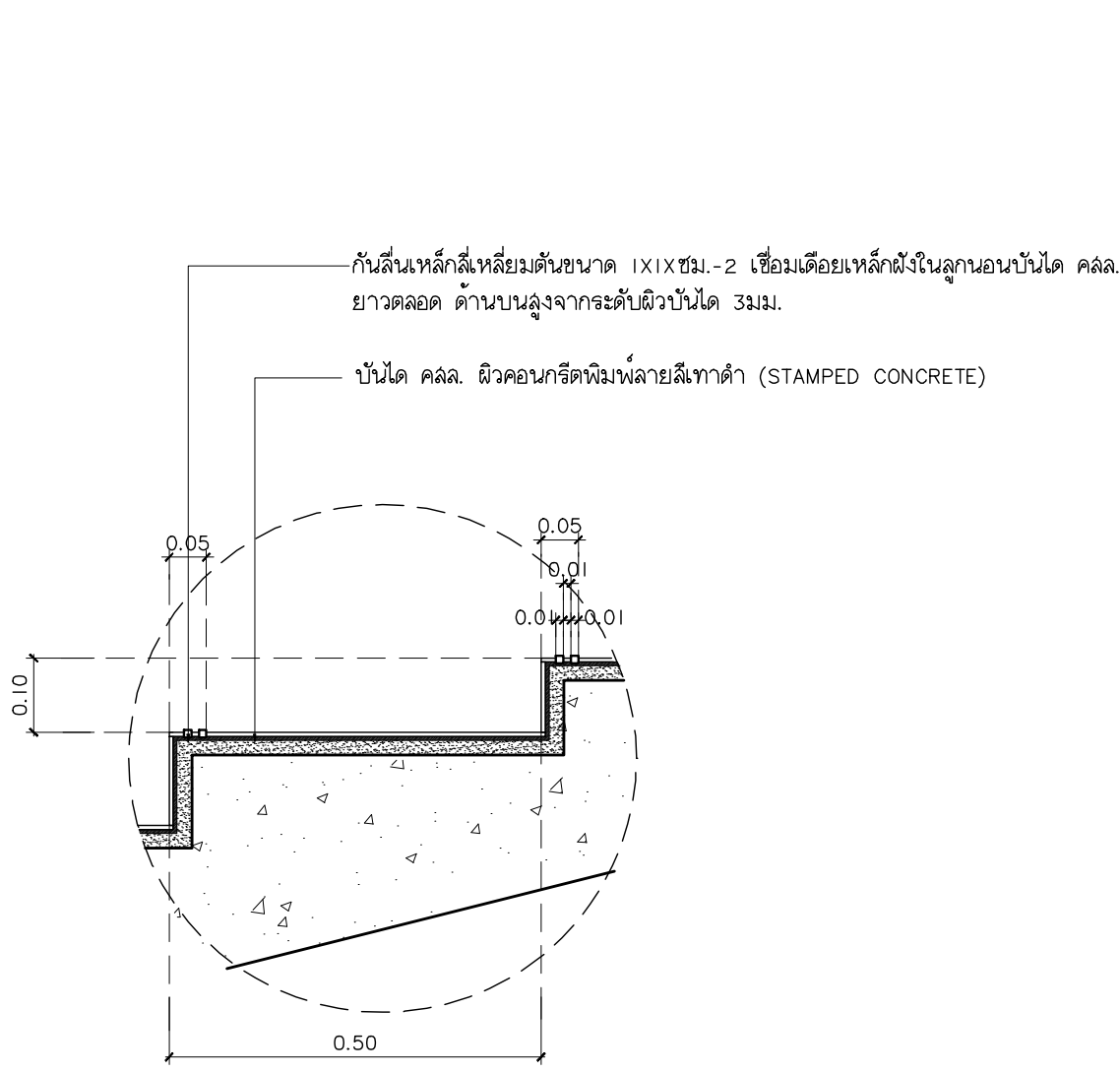
แบบขยายบันได ST5-I มาตราส่วน 1:10
