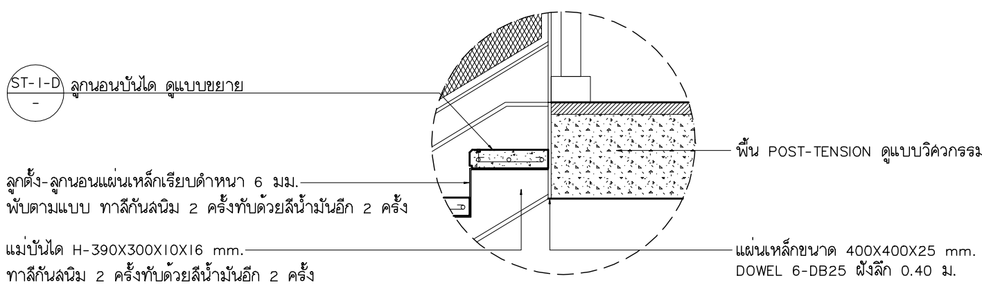
แบบขยาย ST-I-B มาตราส่วน 1:20
