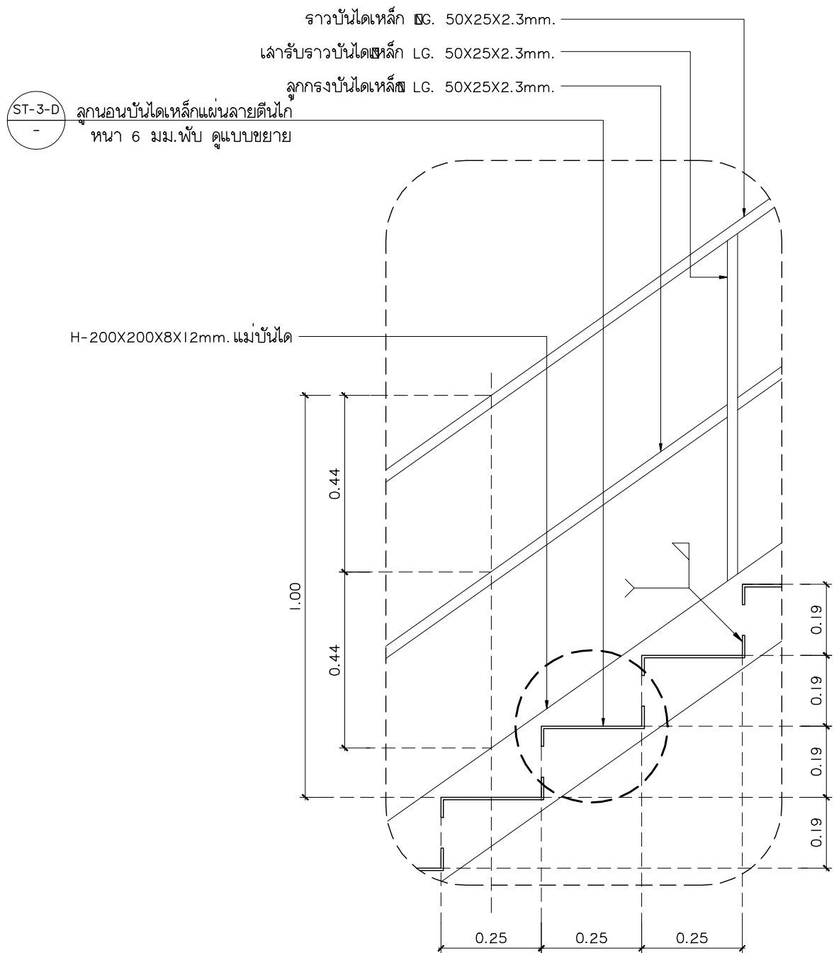
แบบขยาย ST-B มาตราส่วน 1:50
