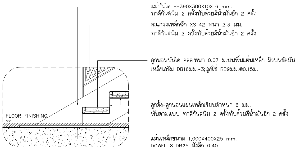
แบบขยาย ST-I-E มาตราส่วน 1:20
