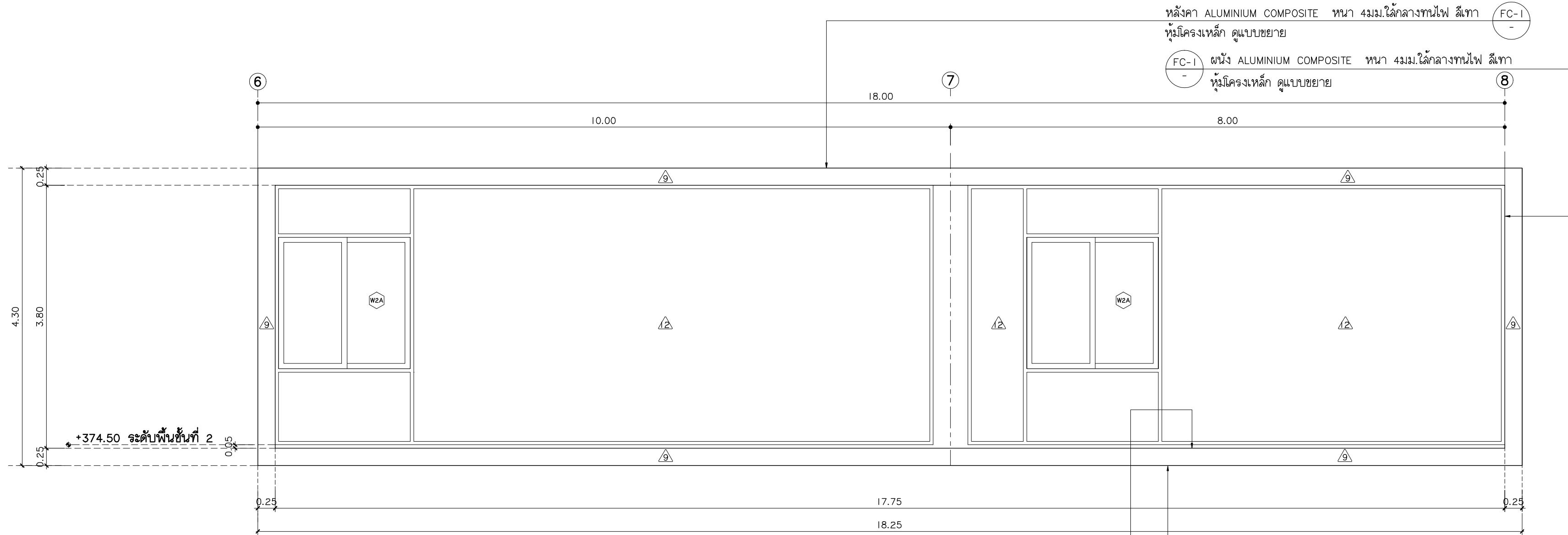
แบบขยาย FC-I รูปด้านหน้า มาตราส่วน 1:50
