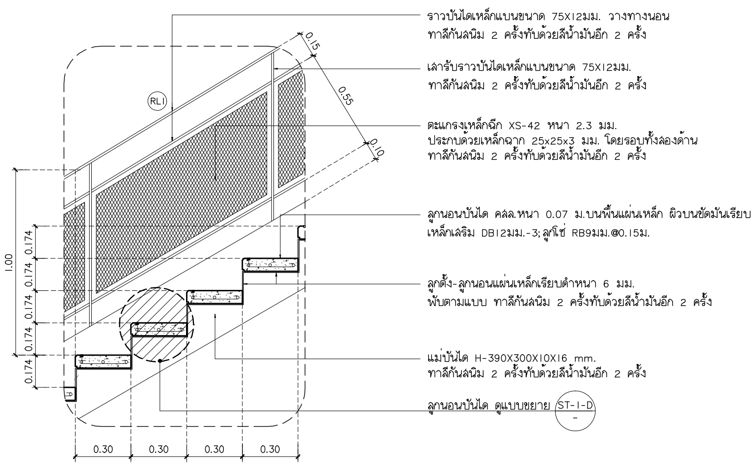
แบบขยายลูกนอนบันได ST-I-C มาตราส่วน 1:20
