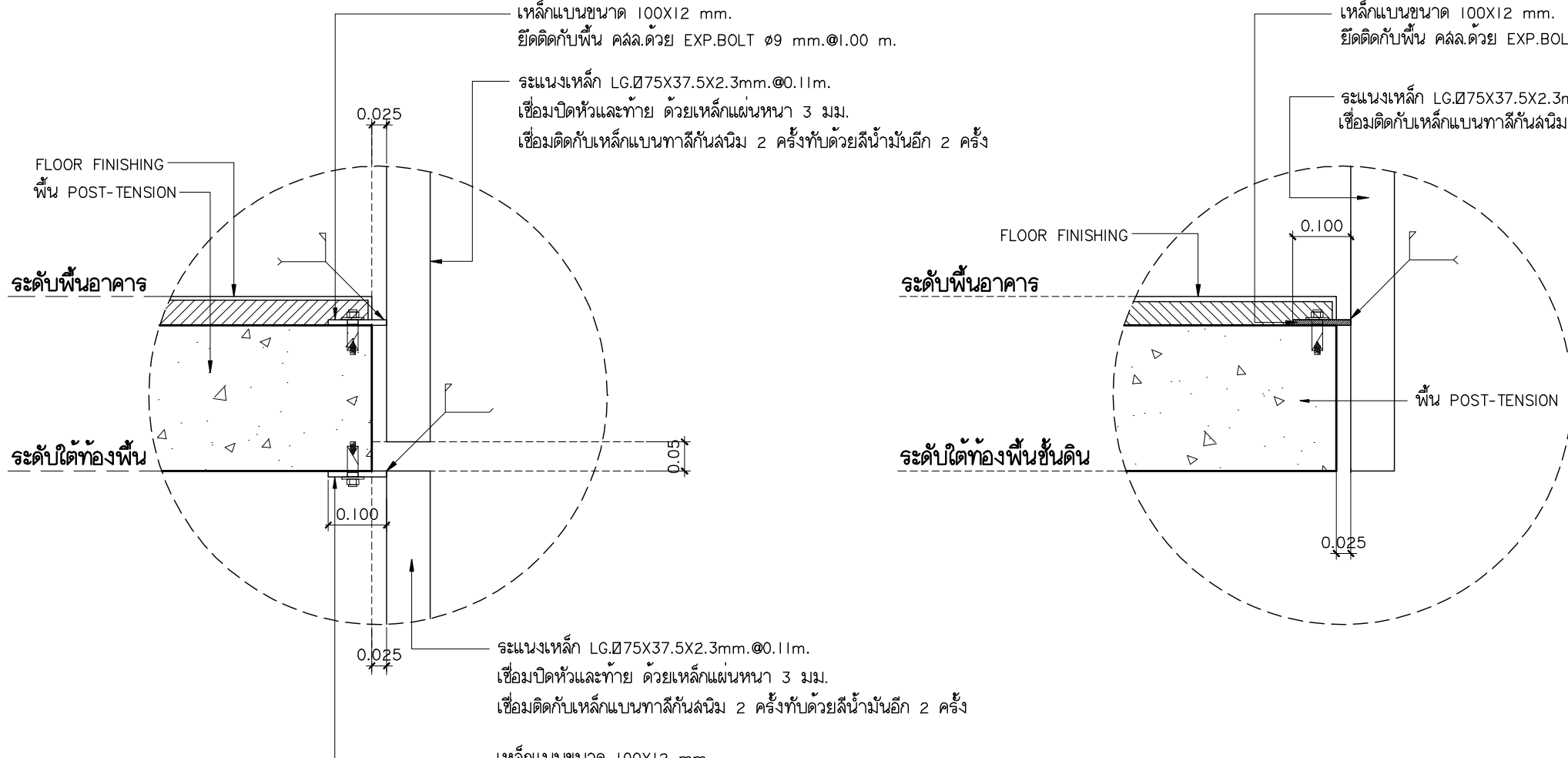
แบบขยาย SSI-2 มาตราส่วน 1:10
