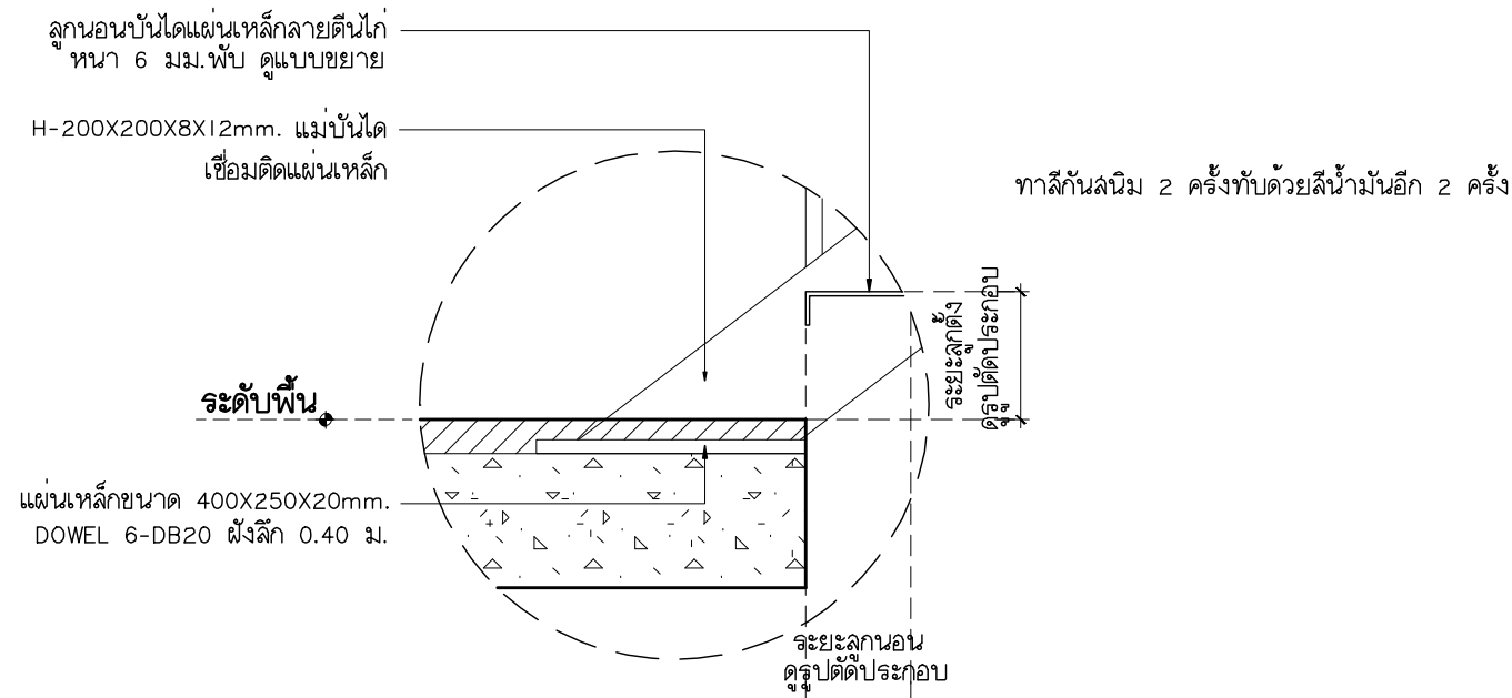
แบบขยาย ST-A มาตราส่วน 1:20
