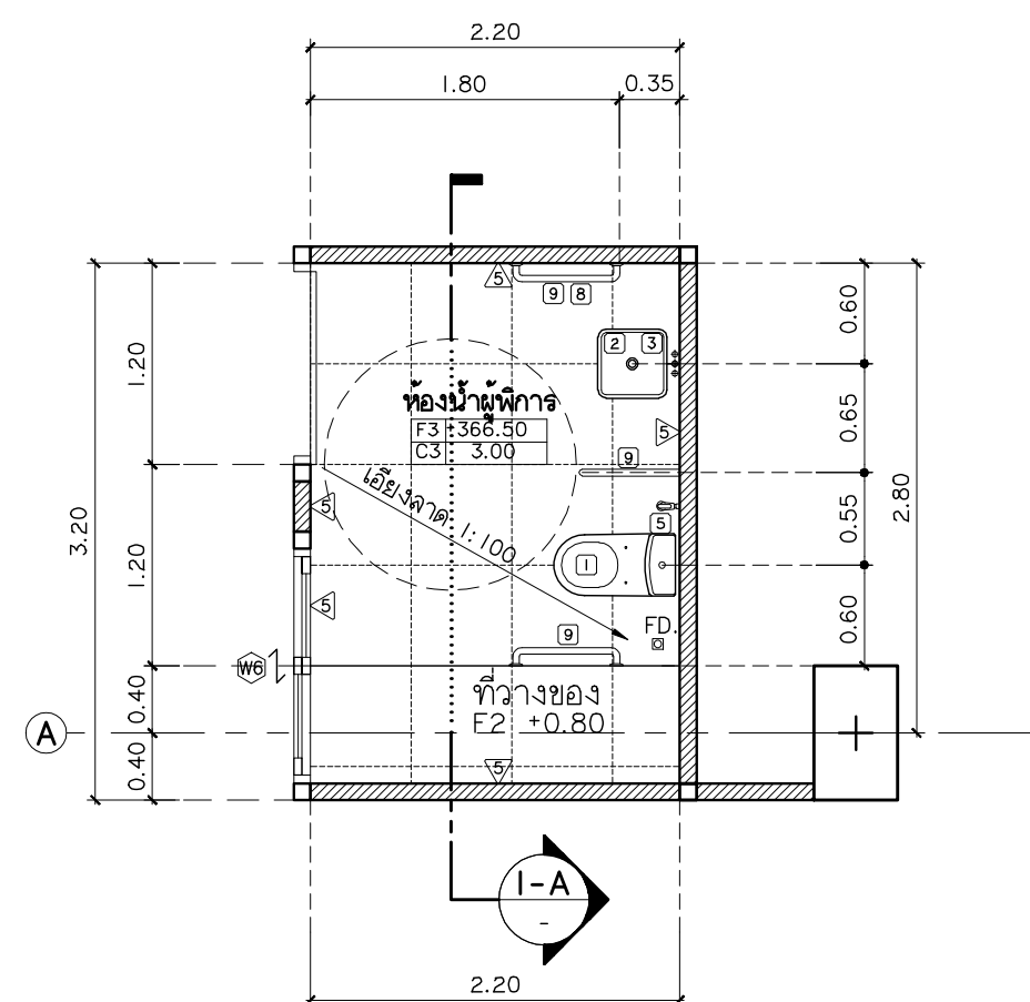
แบบขยายห้องน้ำคนพิการ มาตราส่วน 1:50
