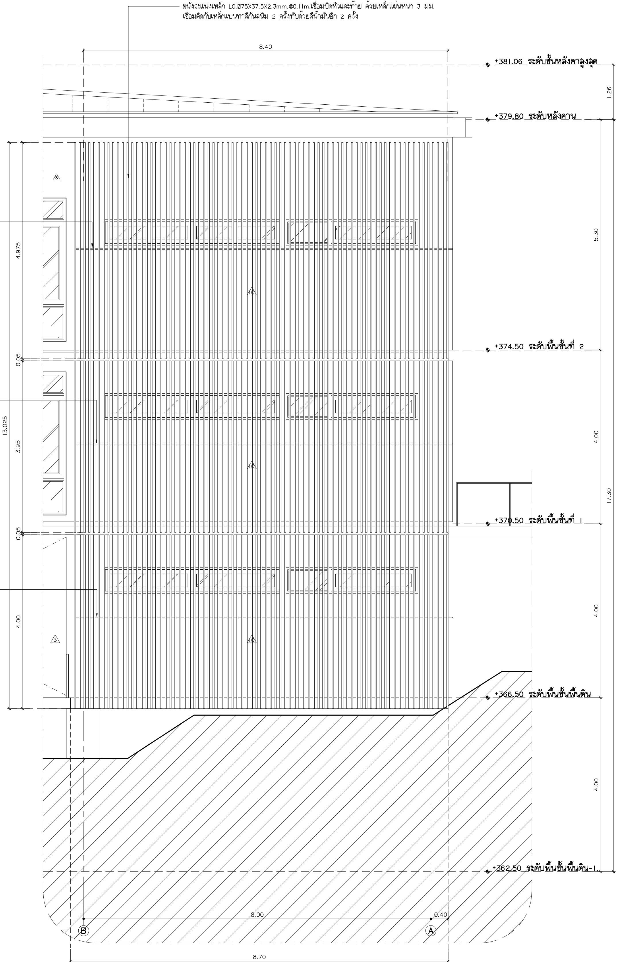
รูปด้านหน้า SSI มาตราส่วน 1:50
