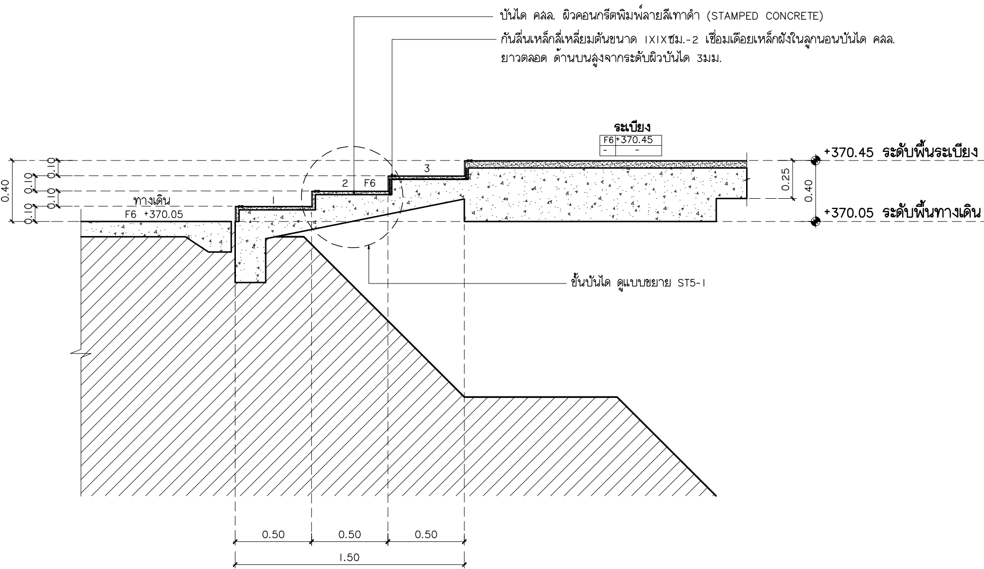
แบบขยายบันได ST5 รูปตัด A มาตราส่วน 1:25
