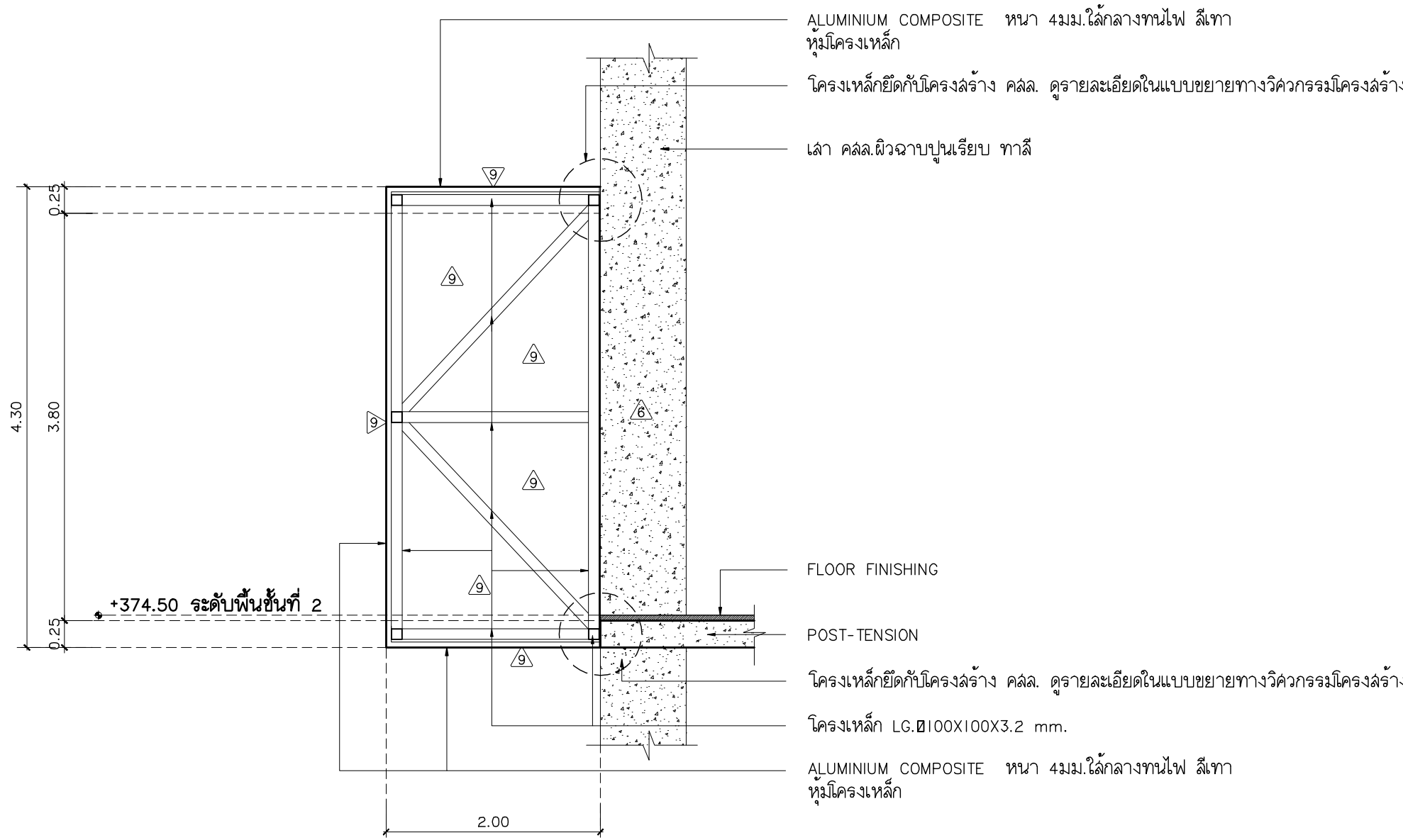
รูปตัด FC-I-A มาตราส่วน 1:50
