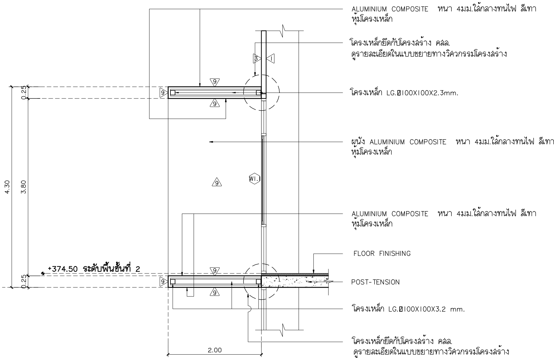
รูปตัด FC-I-B มาตราส่วน 1:50
