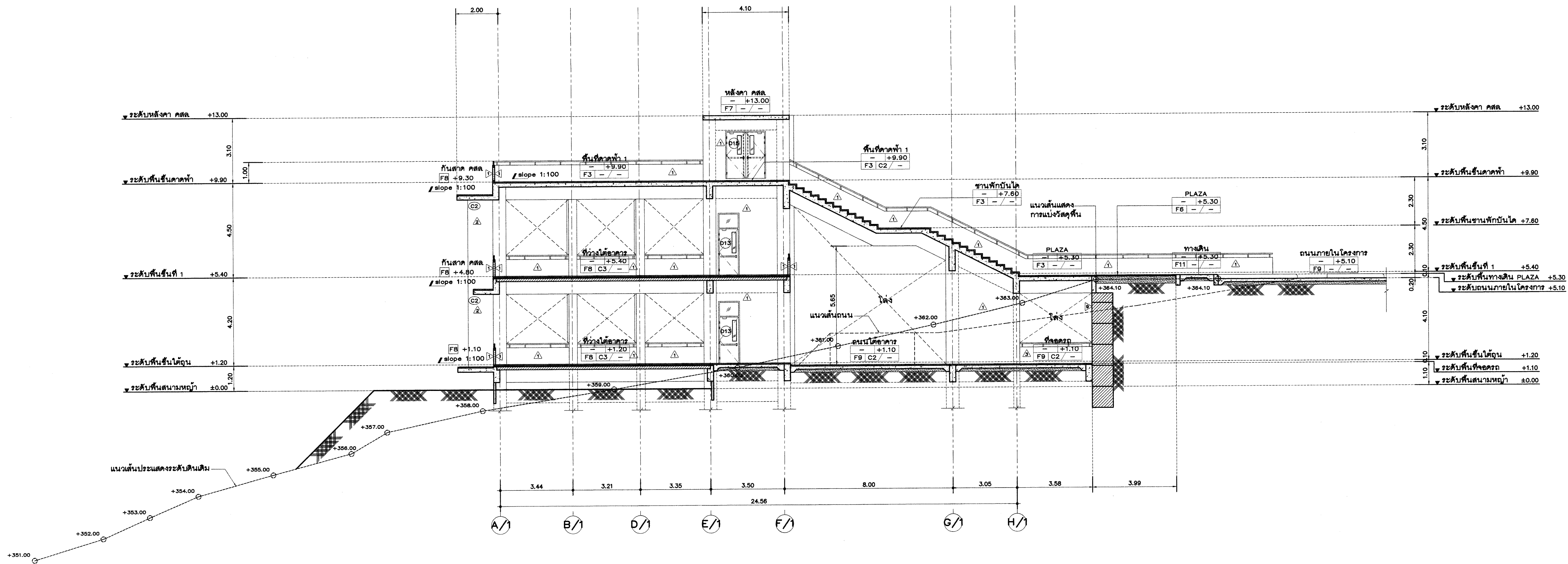
รูปตัด F-F
