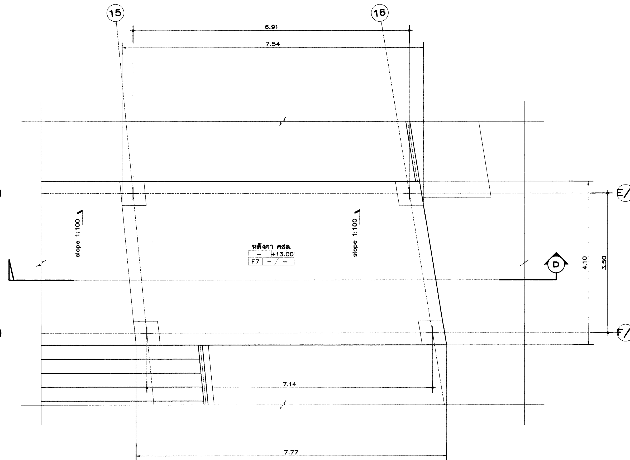
แปลนขยายบันได 3 ชั้นหลังคา คสล. (บันไดหนีไฟ)
