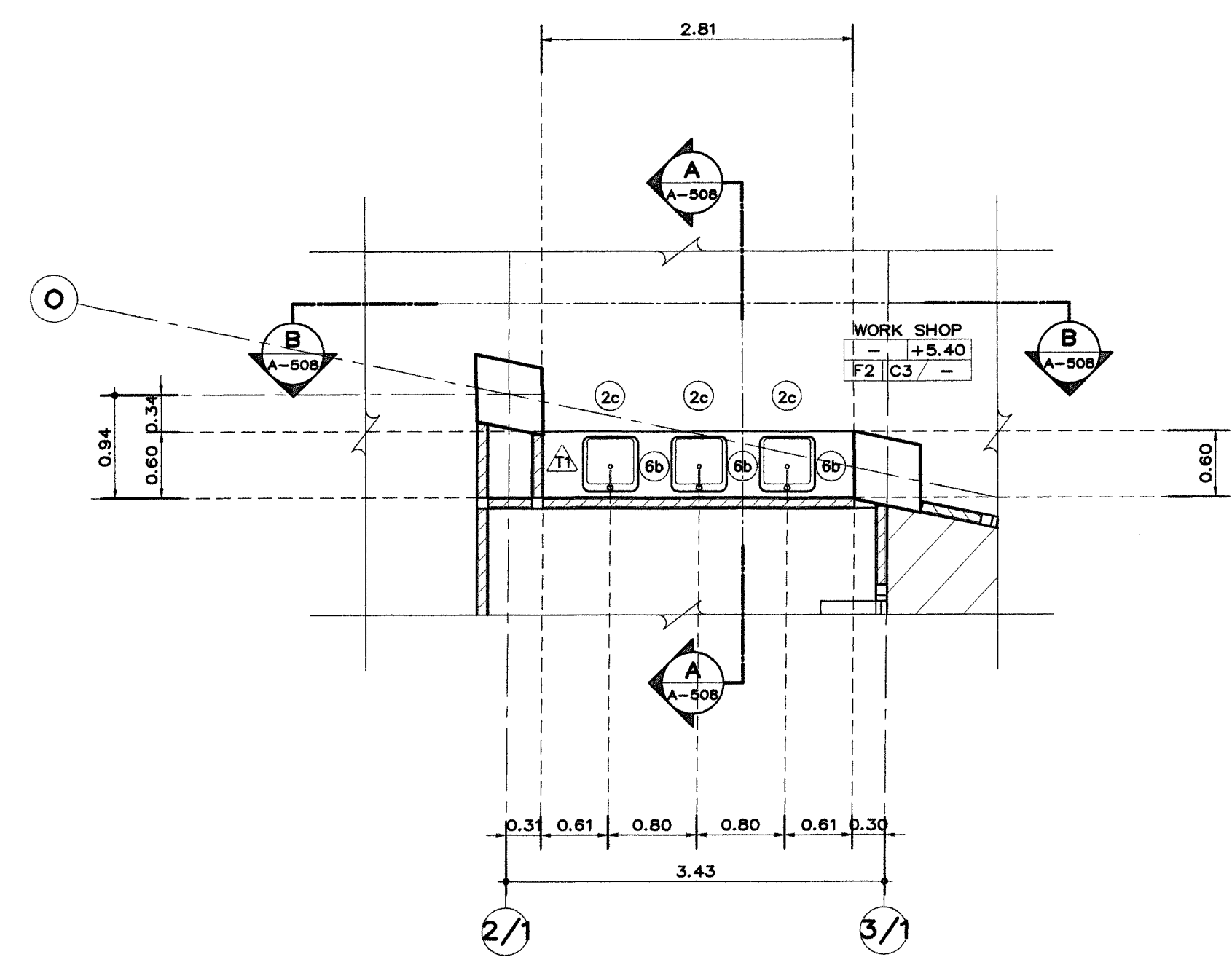
แปลนพื้นแสดงอ่างล้างมือ ห้อง WORK SHOP
