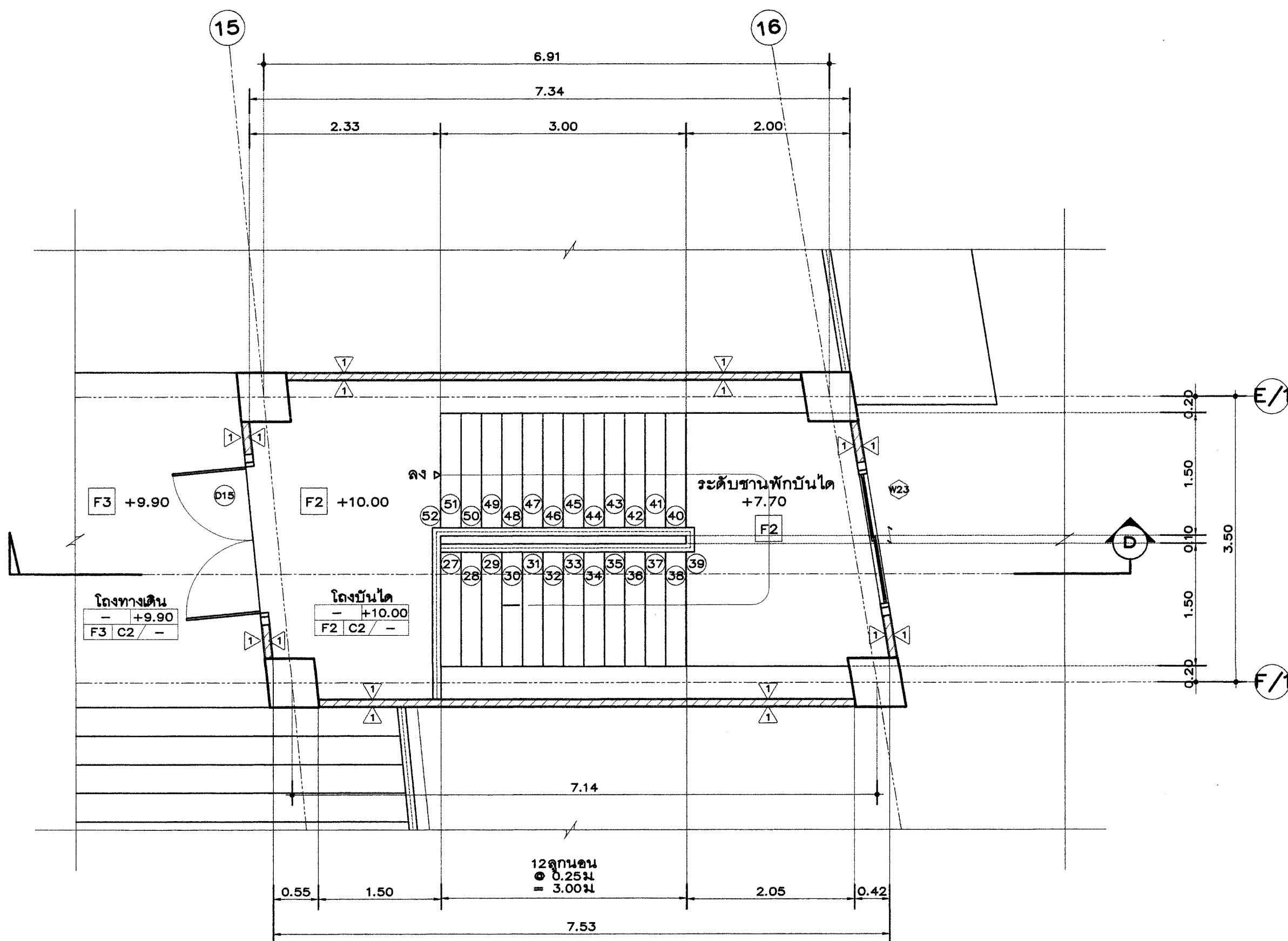
แปลนขยายบันได 3 ชั้นคาดฟ้า (บันไดหนีไฟ)
