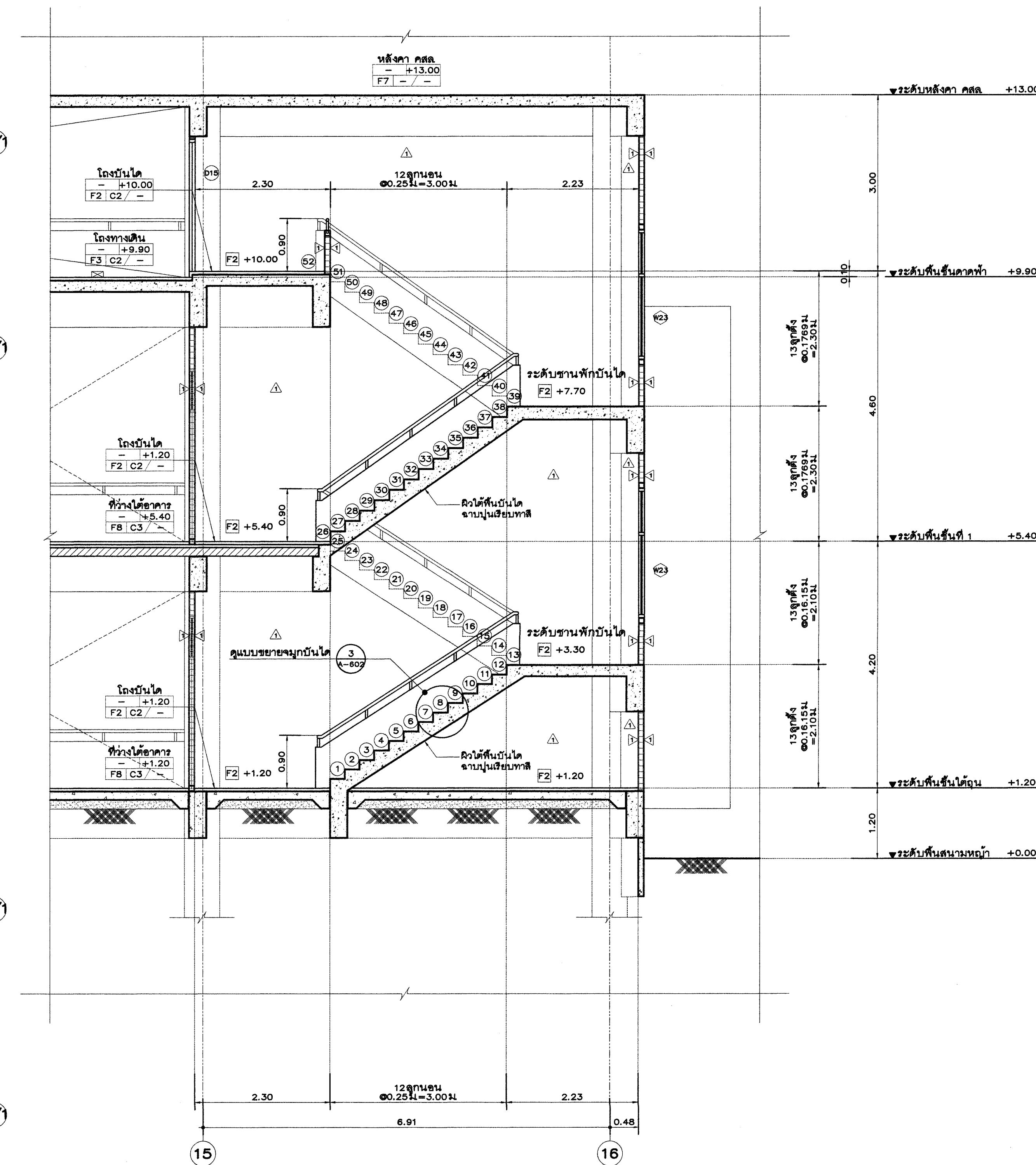
รูปตัด D-D
