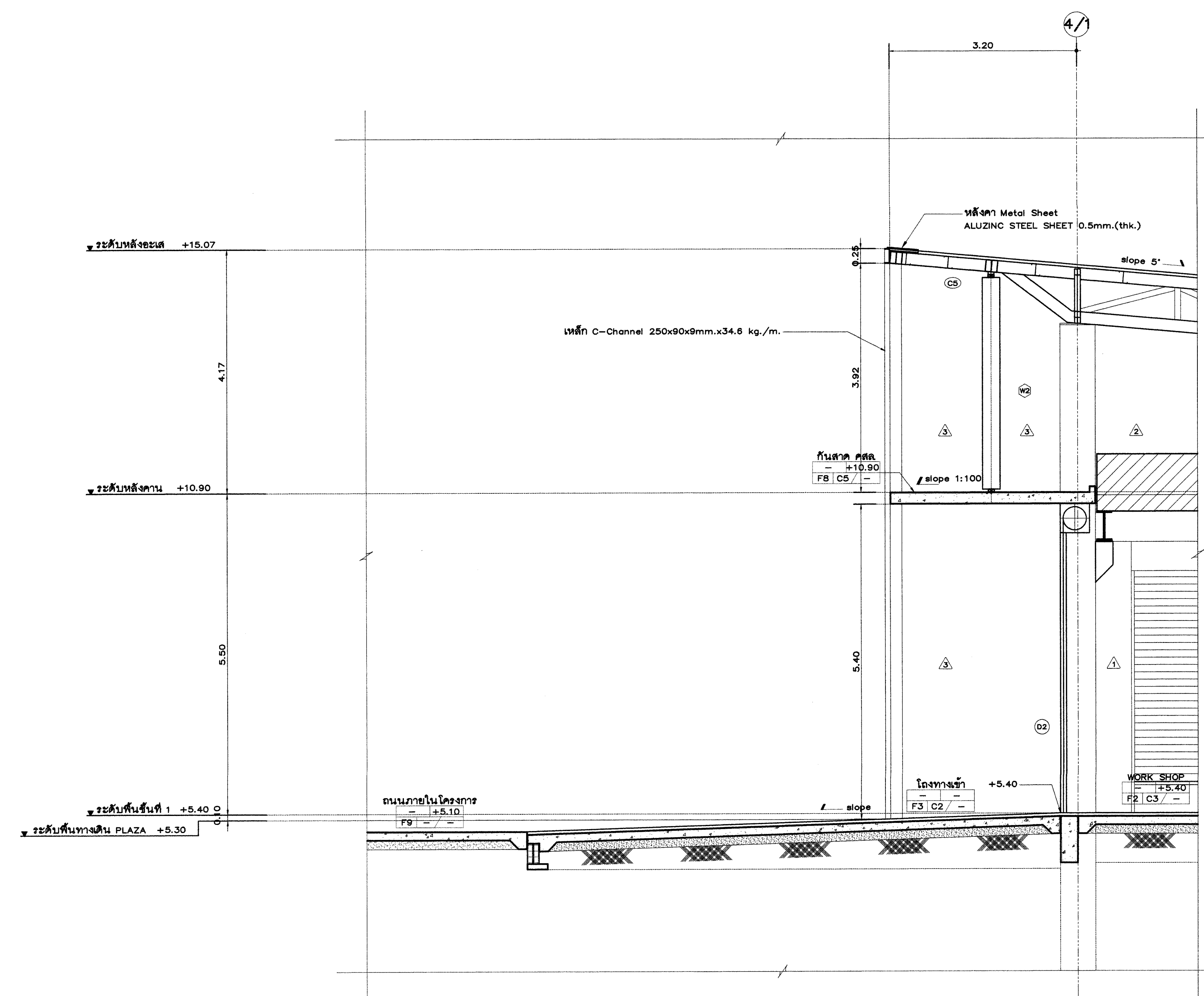
รูปตัด A-A ขนาดส่วน 1:50
