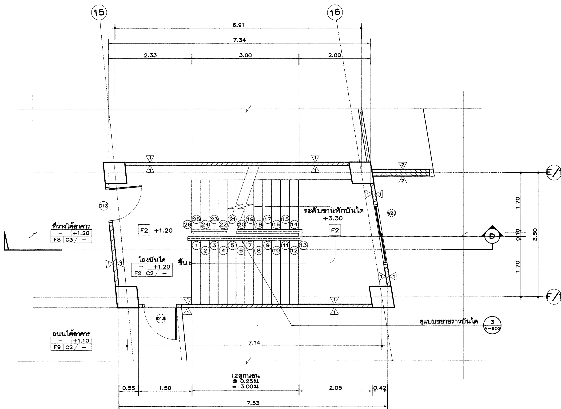
แปลนขยายบันได 3 ชั้นใต้ถุน (บันไดหนีไฟ)
