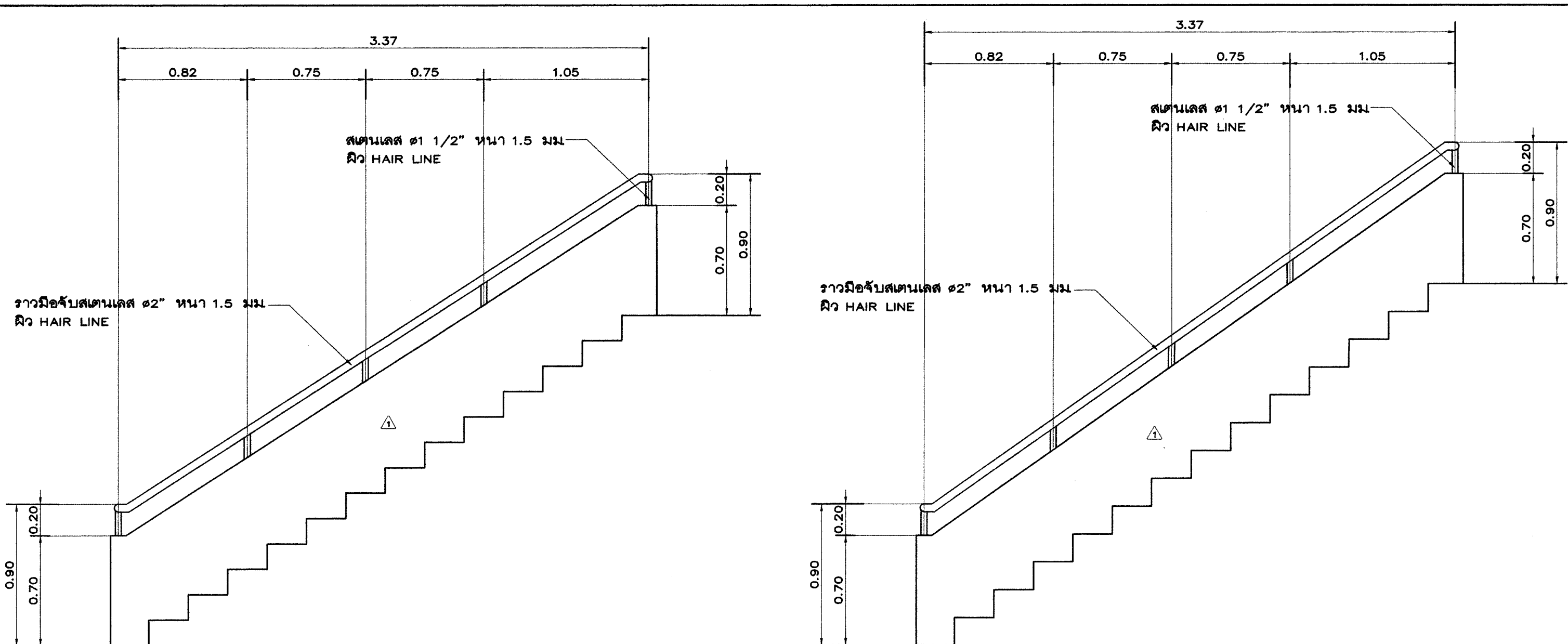
แบบขยายราวบันได 3
