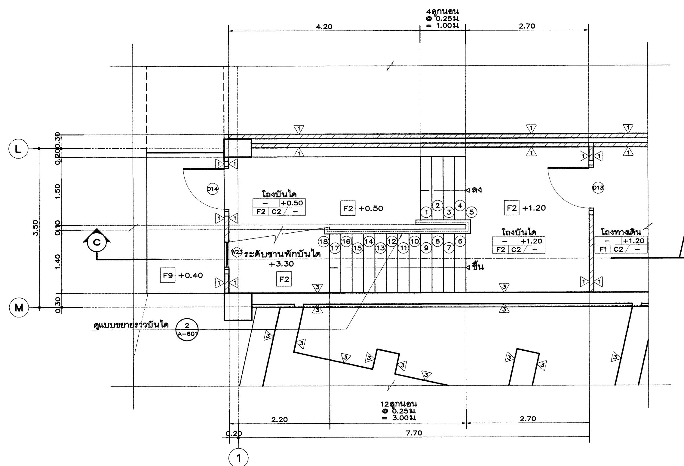
แปลนขยายบันได 2 ชั้นใต้ถุน (บันไดหนีไฟ) SCALE 1:50
