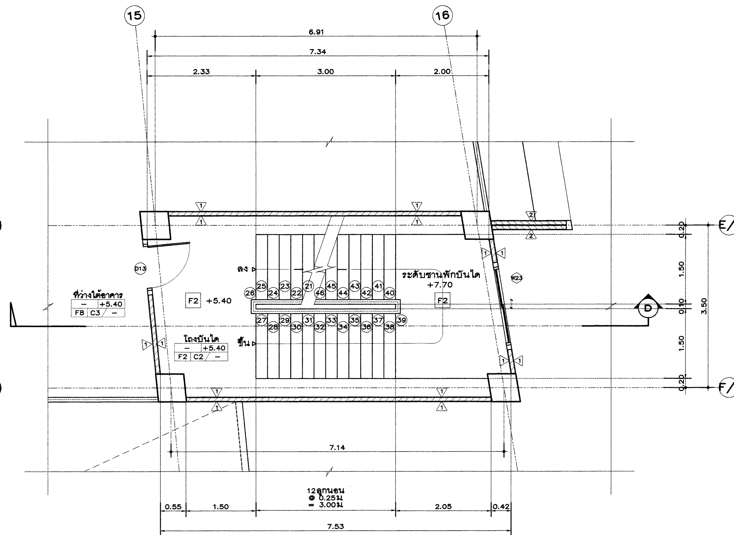
แปลนขยายบันได 3 ชั้นที่ 1 (บันไดหนีไฟ)
