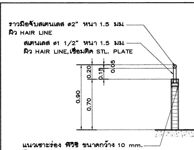
แบบขยายราวบันได
