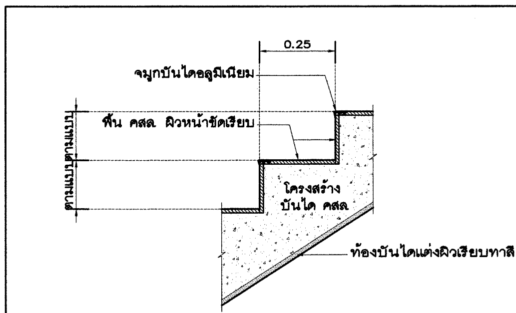
แบบขยายจุกบันได 3
