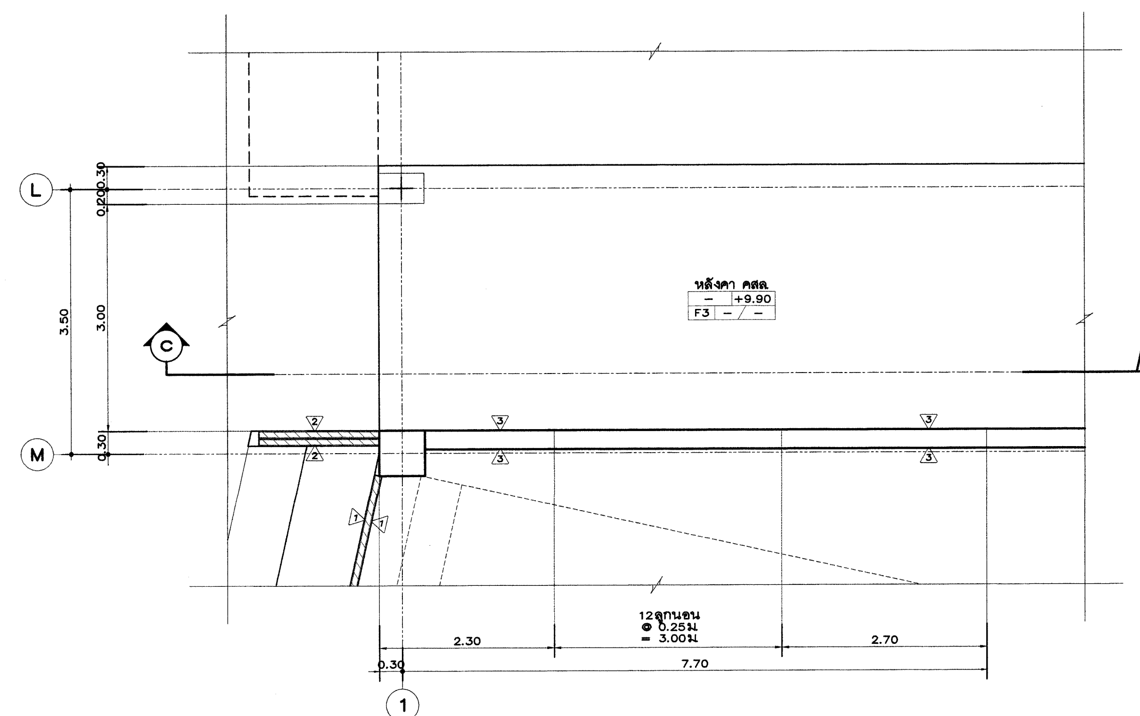
แปลนขยายบันได 2 ชั้นคดฟ้า (บันไดหนีไฟ) SCALE 1:50
