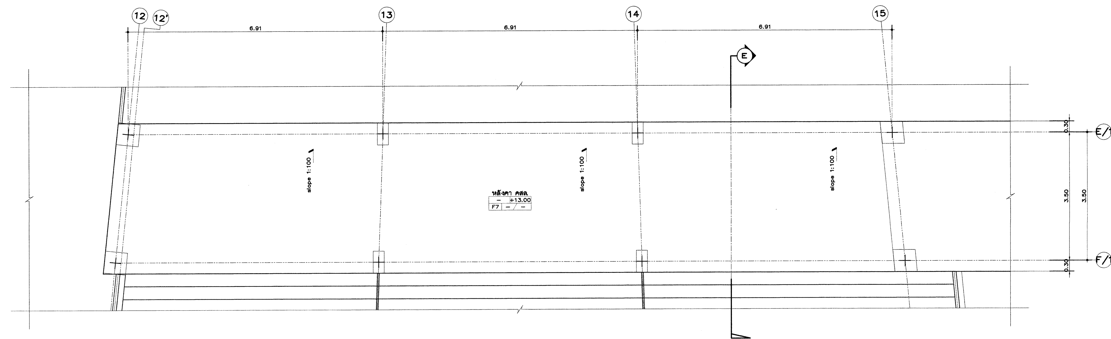
แปลนขยายบันได 4 ชั้นหลังคา คสล. SCALE 1:50
