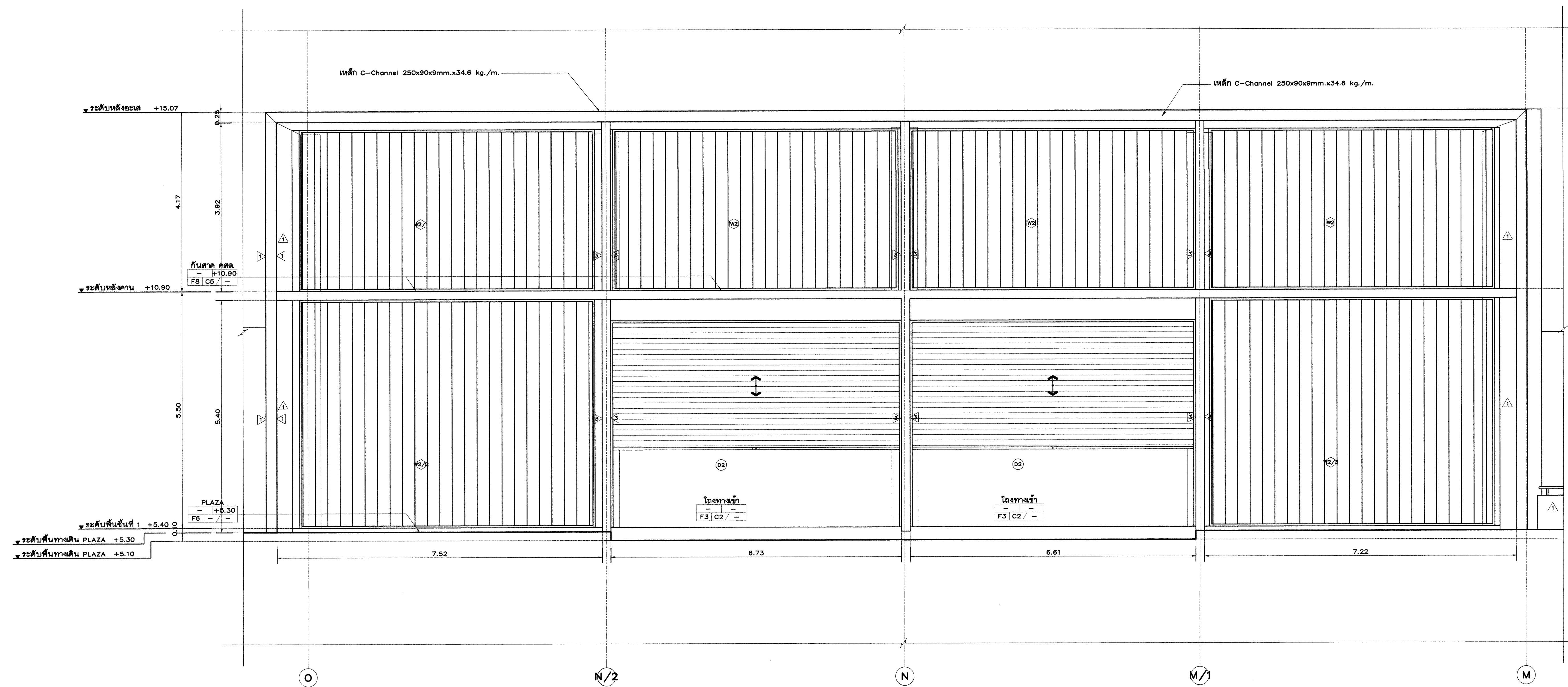
รูปด้าน 1 ขนาดส่วน 1:50
