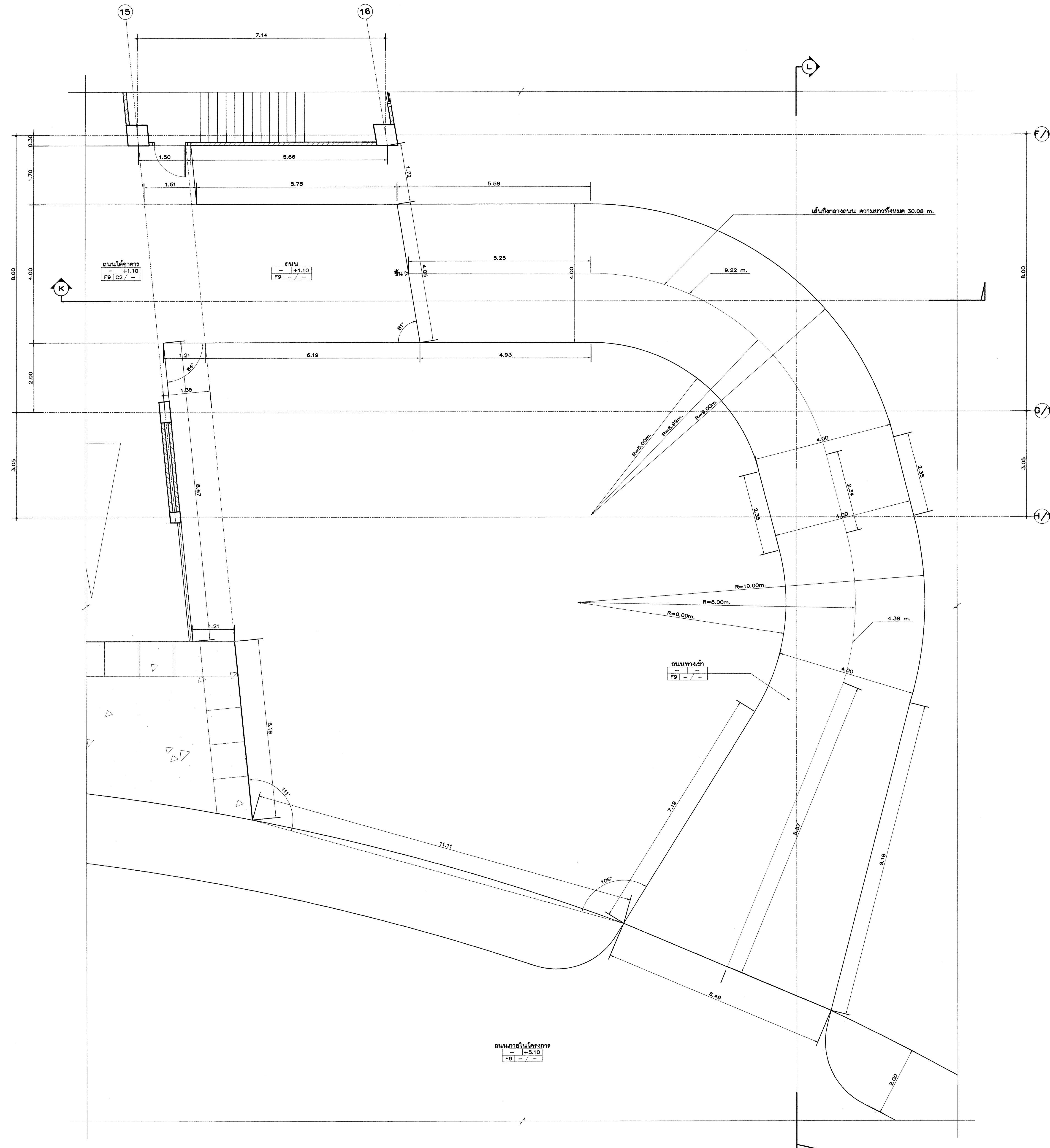
แผนขยายถนนทางเข้าติดต่ออาคาร ชั้นใต้ถุน SCALE 1:50
