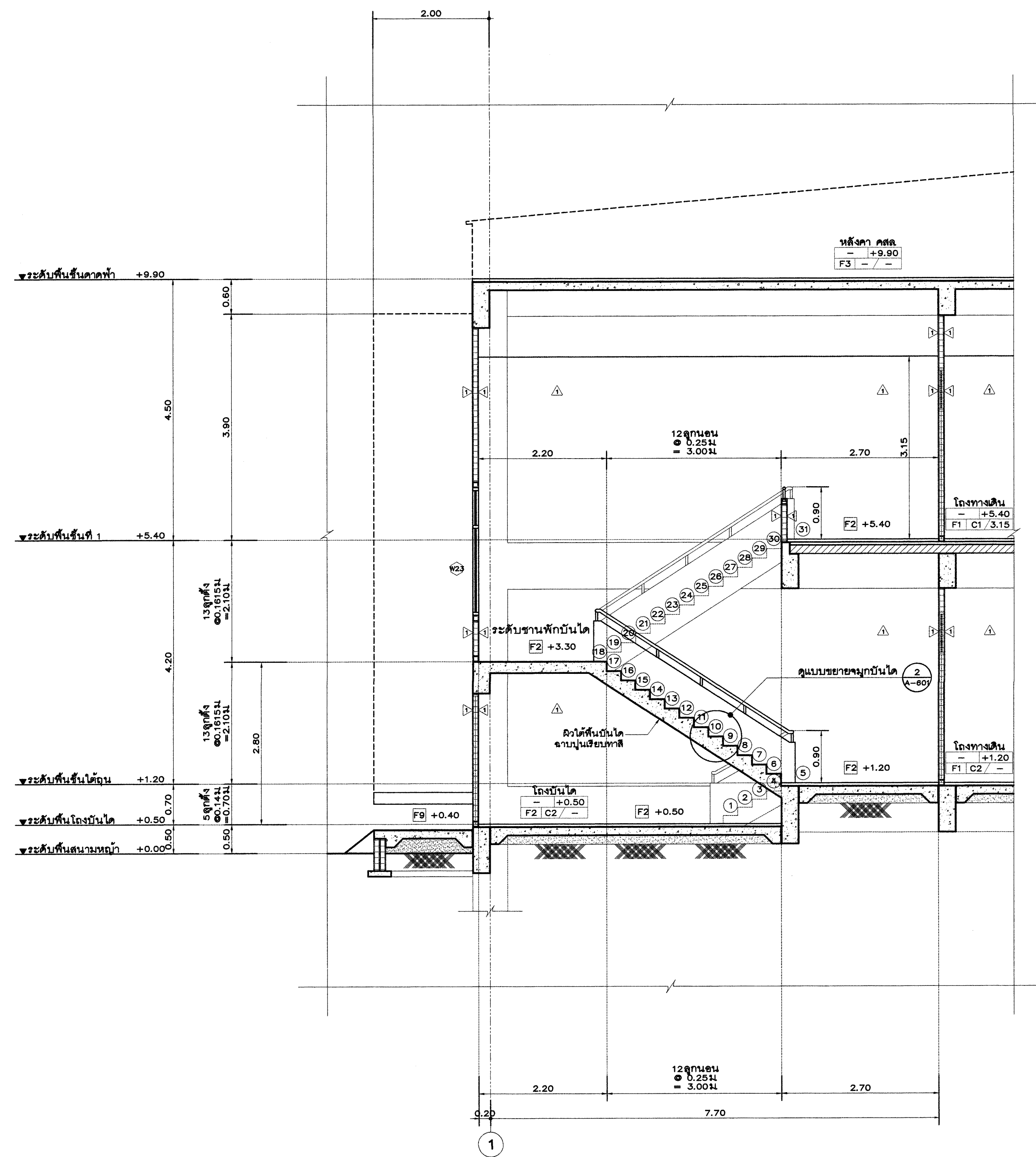
รูปตัด C-C ขนาดส่วน 1:50
