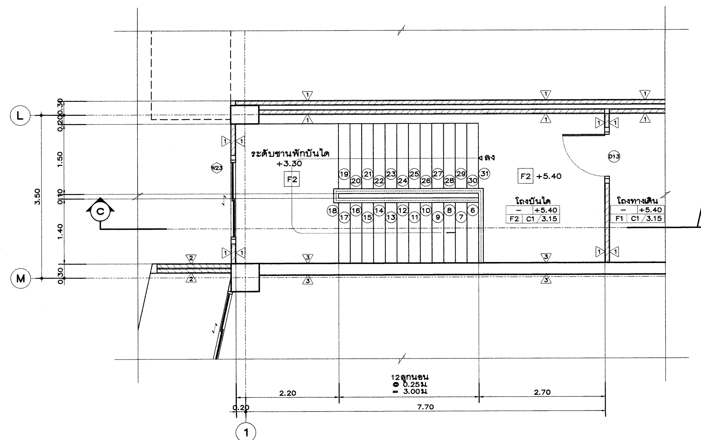
แปลนขยายบันได 2 ชั้นที่ 1 (บันไดหนีไฟ) SCALE 1:50
