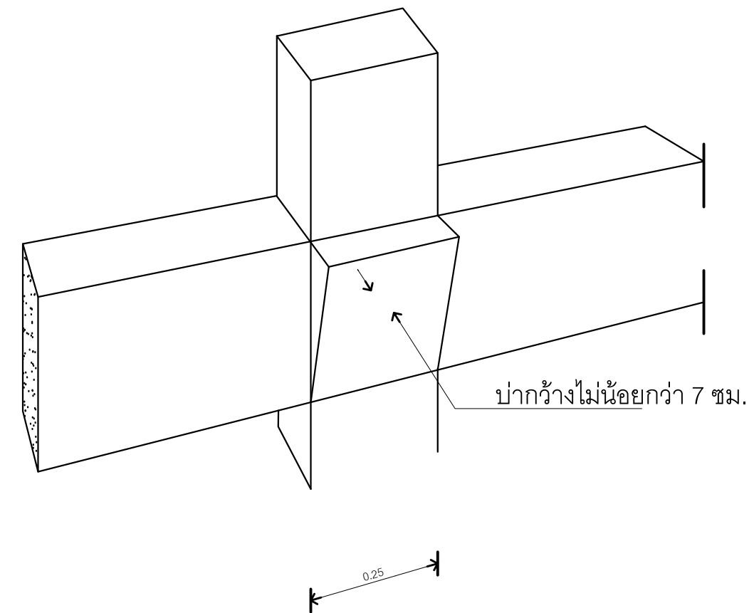
การทำปาดูข้างเสาเพื่อรองรับแผ่น Hollow Core Slab
