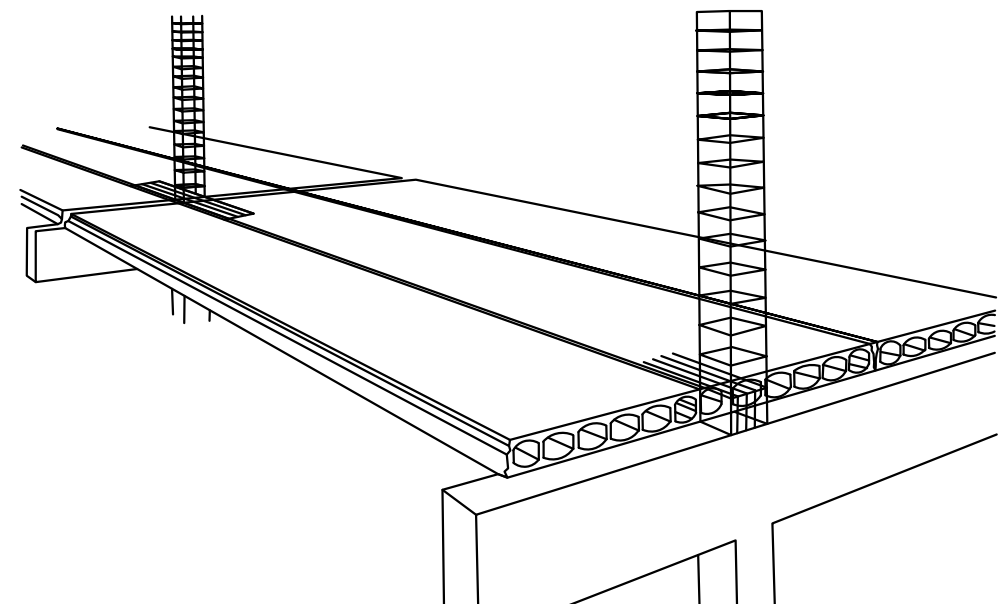
การเสริมเหล็กตามรางพิเศษบริเวณหัวเสา
