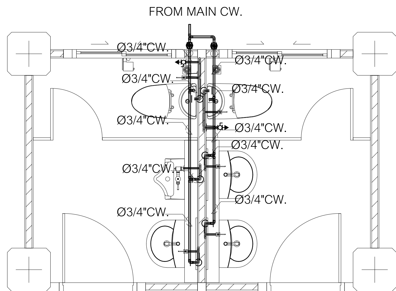
แบบขยายการเดินท่อ CW,HW ภายในห้องน้ำ 02 ชาย,หญิง SCALE 1 : 25
