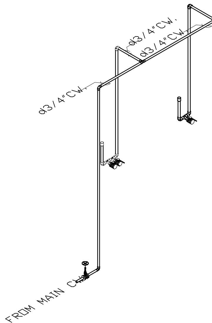
ISOMETRICการเดินท่อ CW,HW ภายในห้องน้ำ 03 วิทยากร
