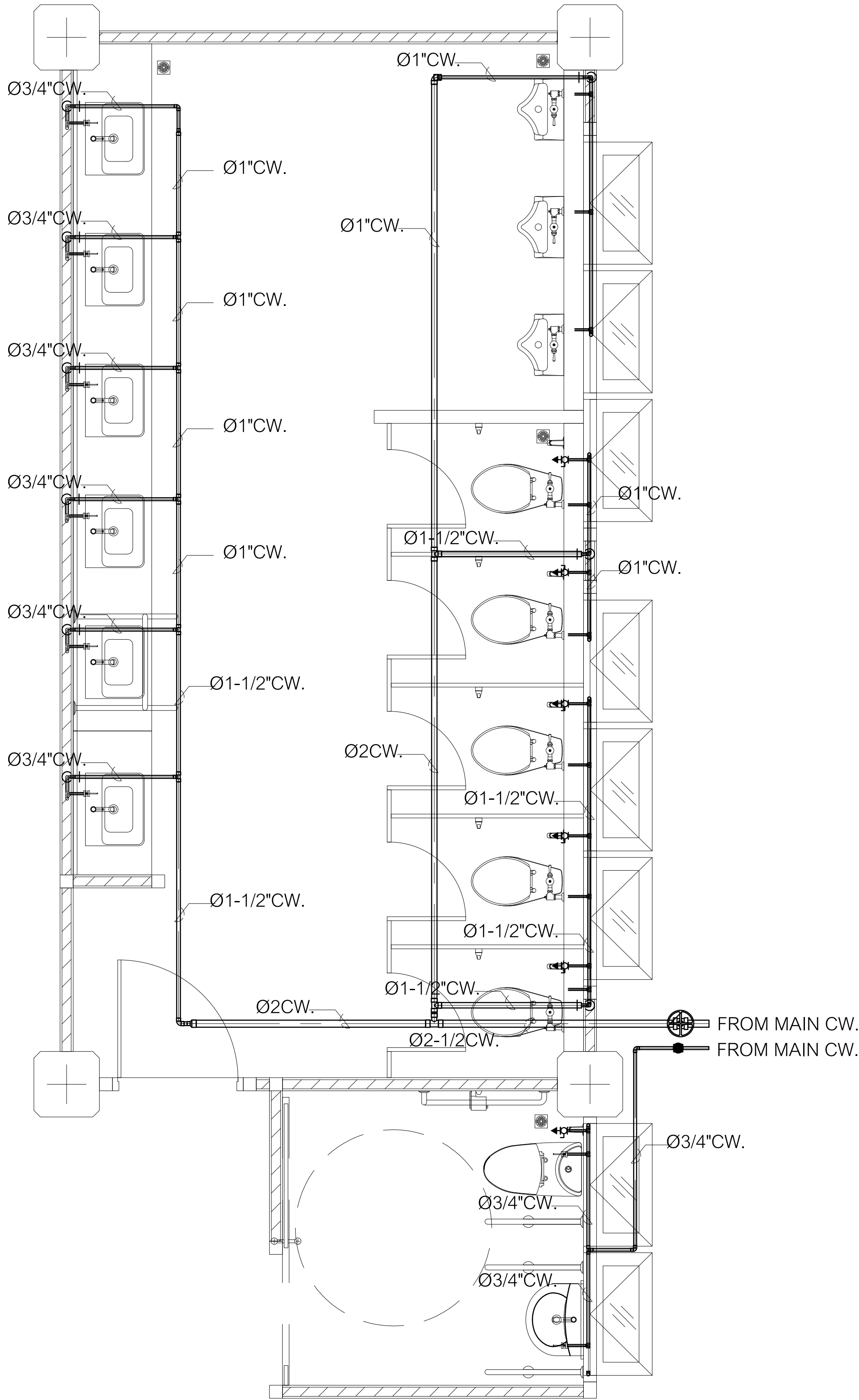
แบบขยายการเดินท่อ CW,HW ภายในห้องน้ำ 01 ชาย, ผู้พิการชาย SCALE 1 : 25
