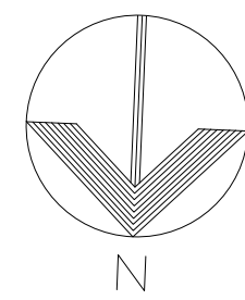
แปลนระบบระบายน้ำหลังคา มาตราส่วน 1:100
