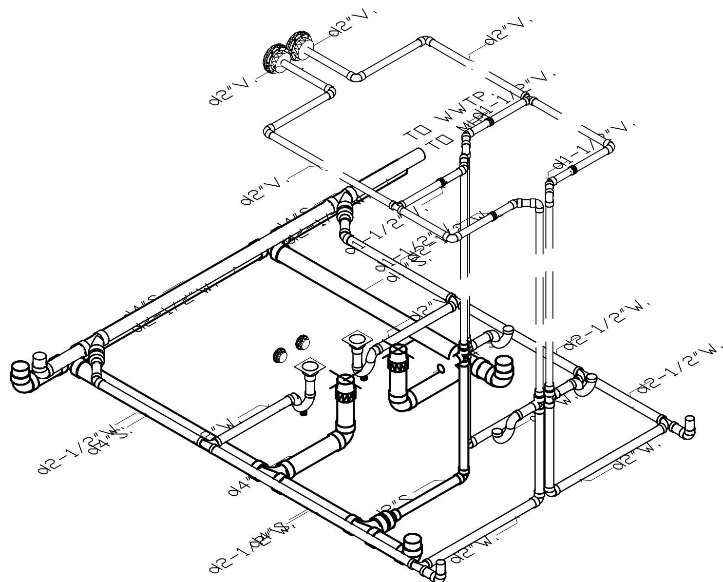
ISOMETRICการเดินท่อ S,W,V ภายในห้องน้ำ 02 ชาย,หญิง
