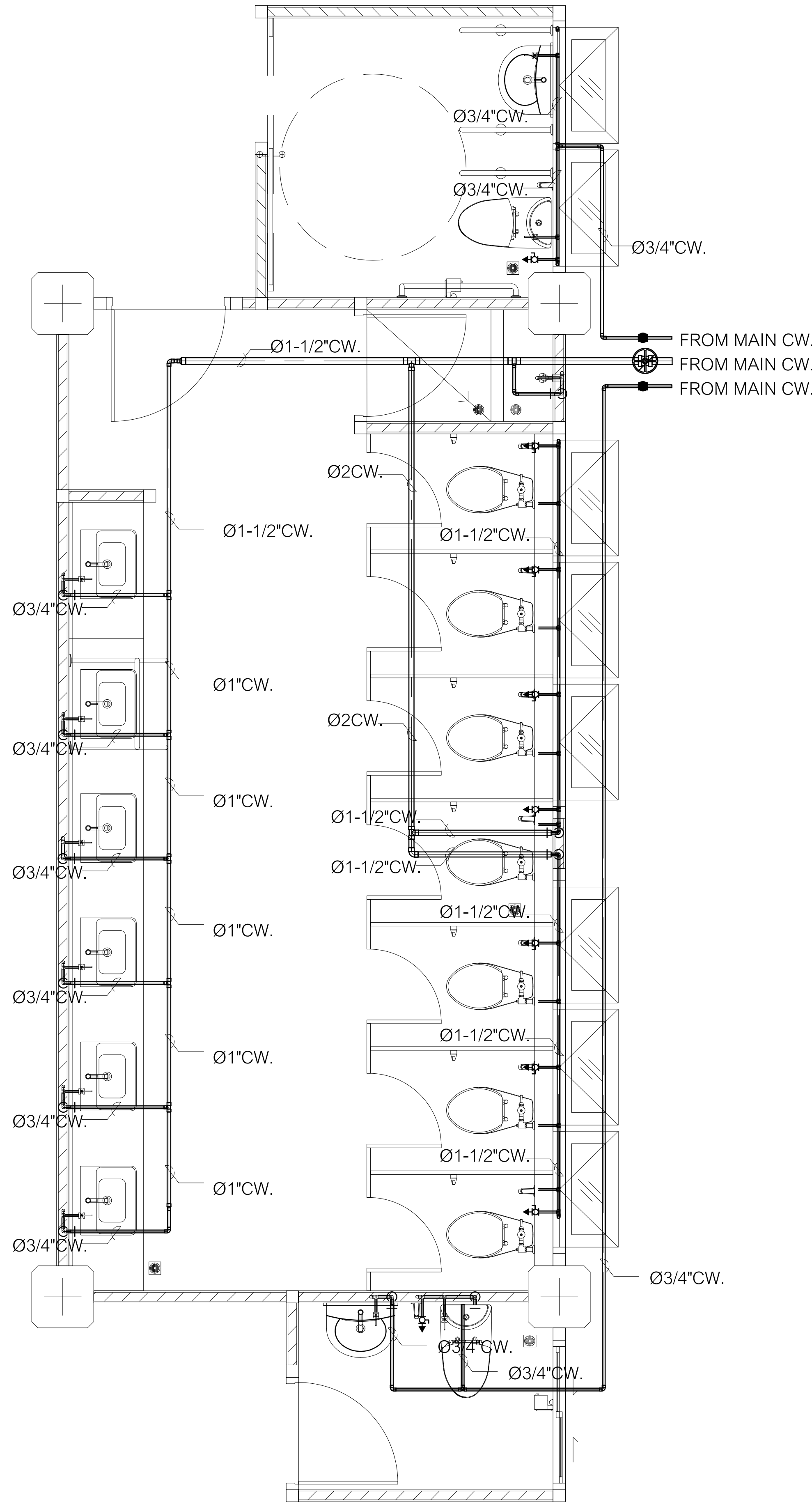
แบบขยายการเดินท่อ CW,HW ภายในห้องน้ำ 01 หญิง , ผู้พิการหญิง,04 พยาบาล
