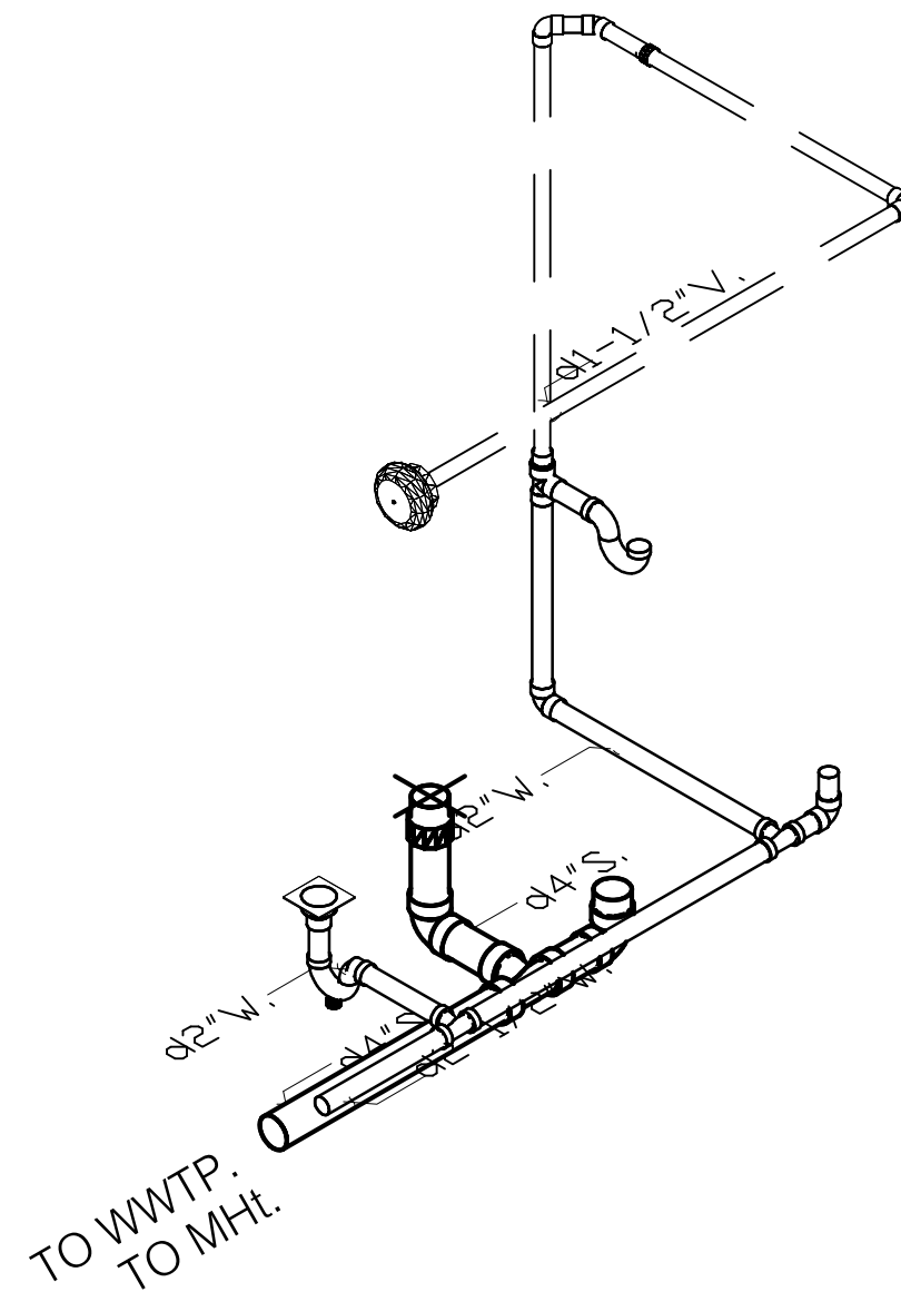
ISOMETRICการเดินท่อ S,W,V ภายในห้องน้ำ 03 วิทยากร
