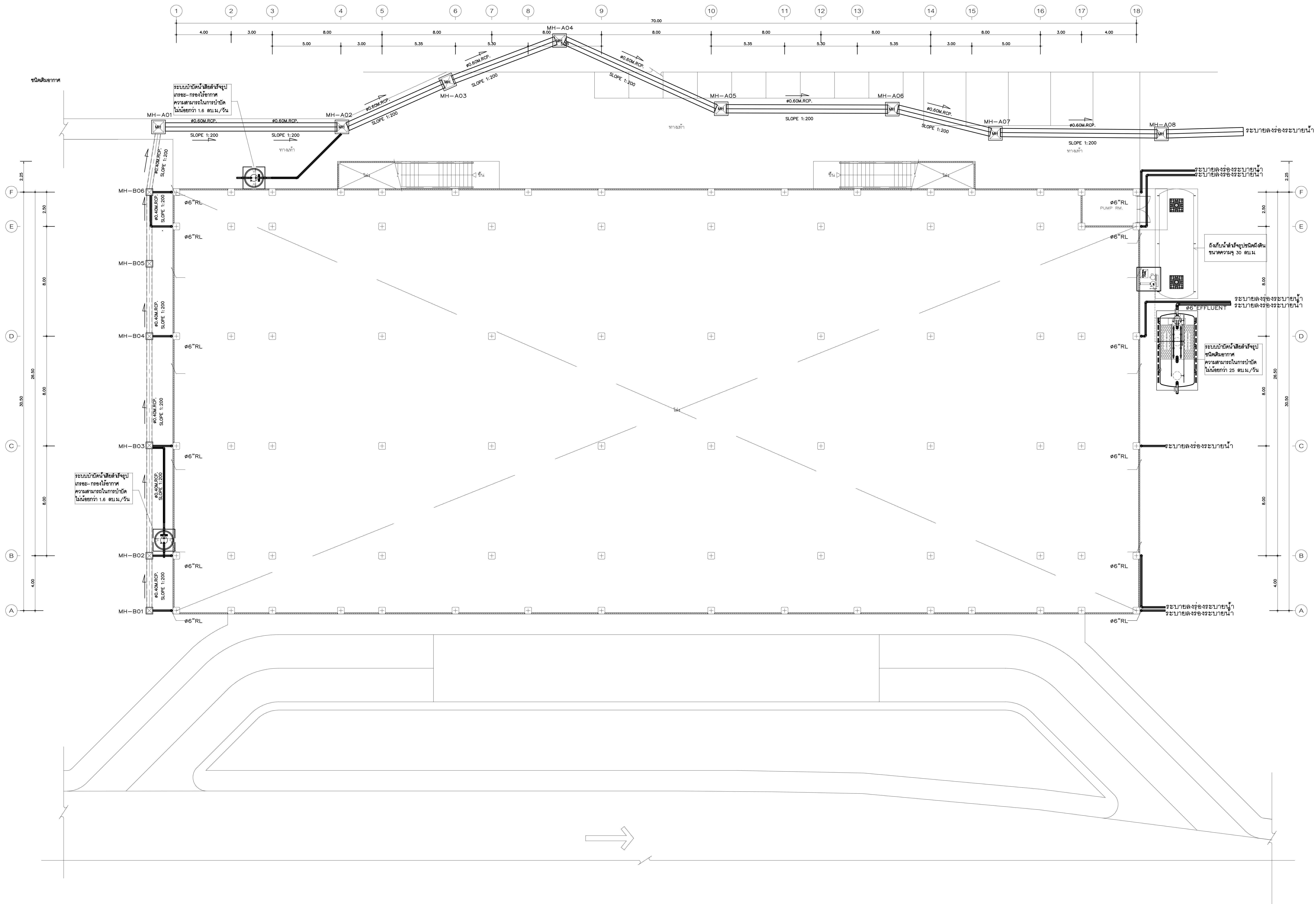
แผนระบบท่อระบายน้ำ ชั้นที่ 1
