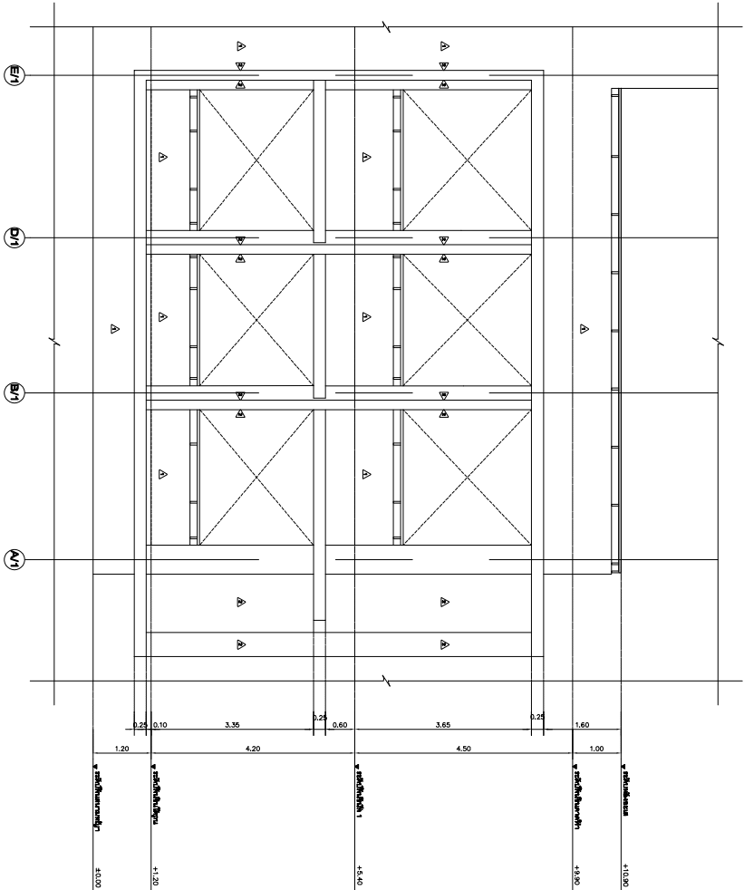
지붕면 2 1:500
